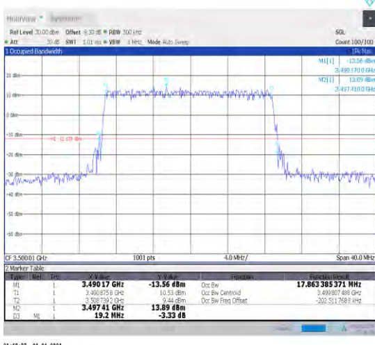
1-N78-3450-3550-30-20-M-5-DFT-256QAM-Outer_F ull-50@0-Ant1-17.863-19.200-≤20-PASS
