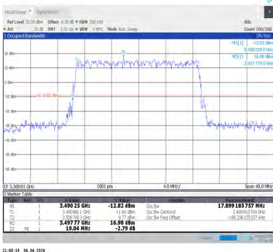
1-N78-3450-3550-30-20-M-3-DFT-16QAM-Outer_Ful I-50@0-Ant1-17.899-19.040-≤20-PASS
