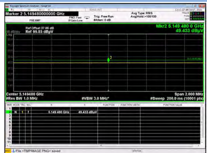
U-NII-1 11ac80 CH42 AV
