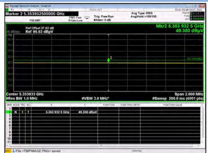
U-NII-2A 11ac80 CH58 AV
