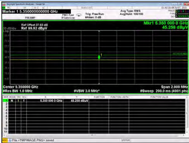
U-NII-2A 11n20 CH64 AV
