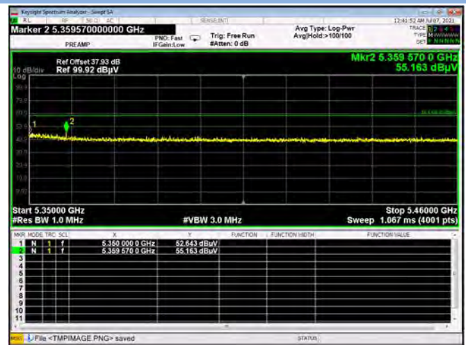
U-NII-2A 11n40 CH62 Peak
