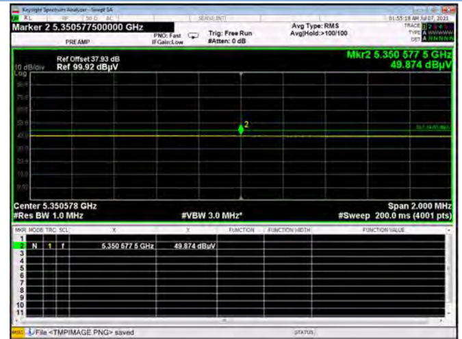
U-NII-2A 11ac40 CH62 AV
