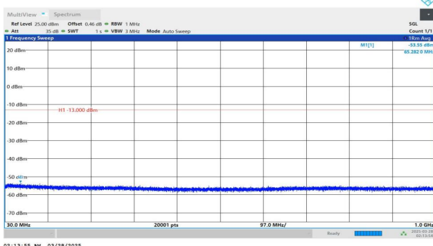
Band2-9400-1-30~1000MHz-PASS
