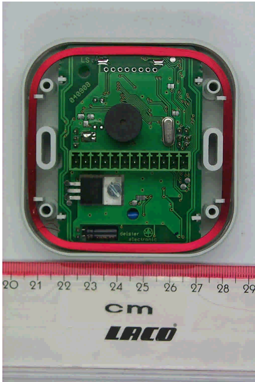
41092B_d.jpg PRD5 / SWH-4100, rear view
