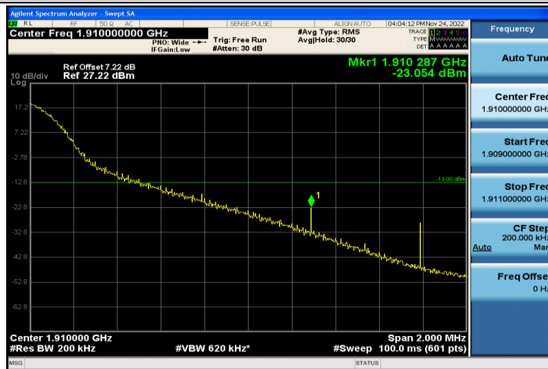
Band2-20MHz-16QAM-19100-1RB#99
