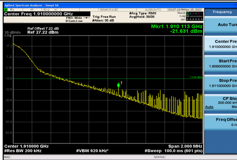
Band2-20MHz-64QAM-19100-1RB#99
