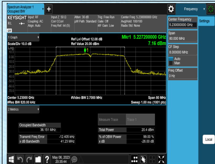
11AC40MIMO-Ant1-5230
