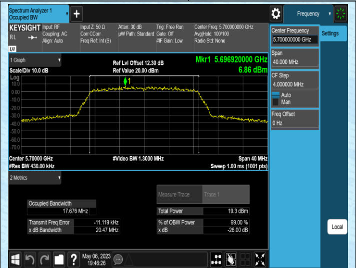
11N20MIMO-Ant2-5700
