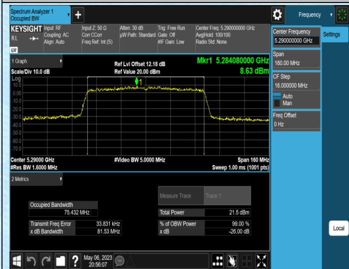
11AC80MIMO-Ant1-5290
