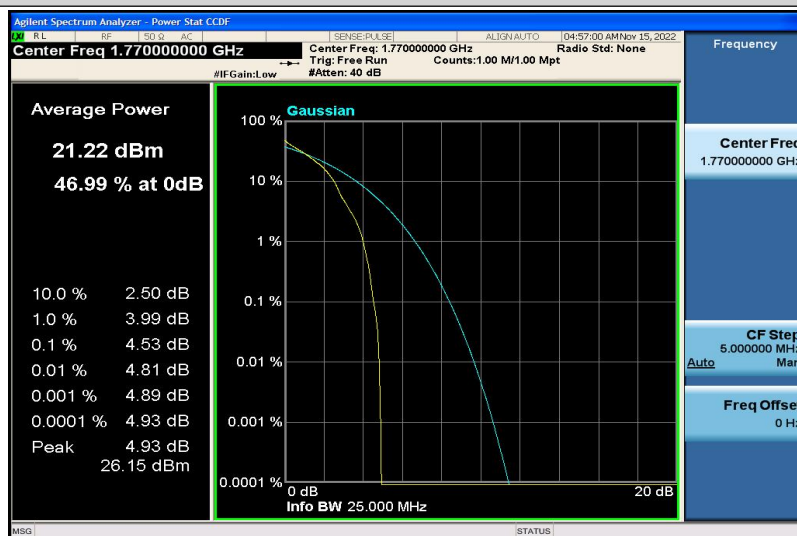
Band66-20MHz-QPSK-132572-1RB#0
