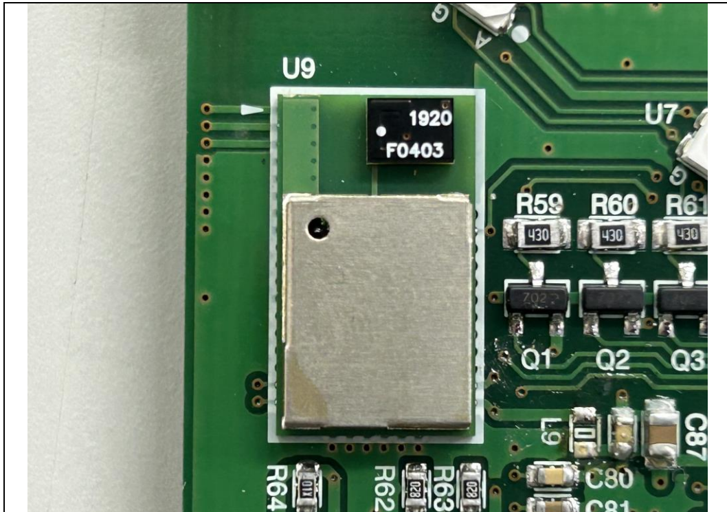
BT Module
