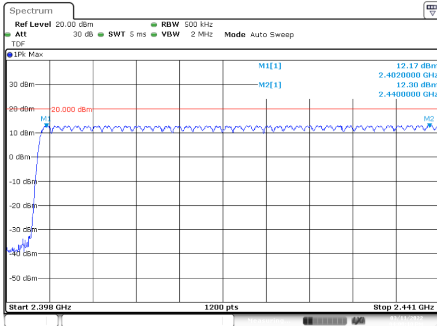
EDR – \pi/4 -DPSK
