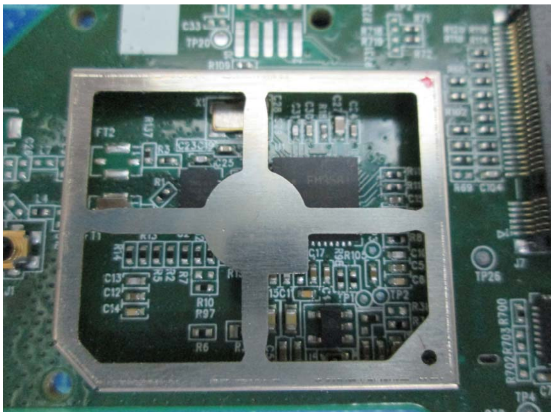
Zigbee Module
