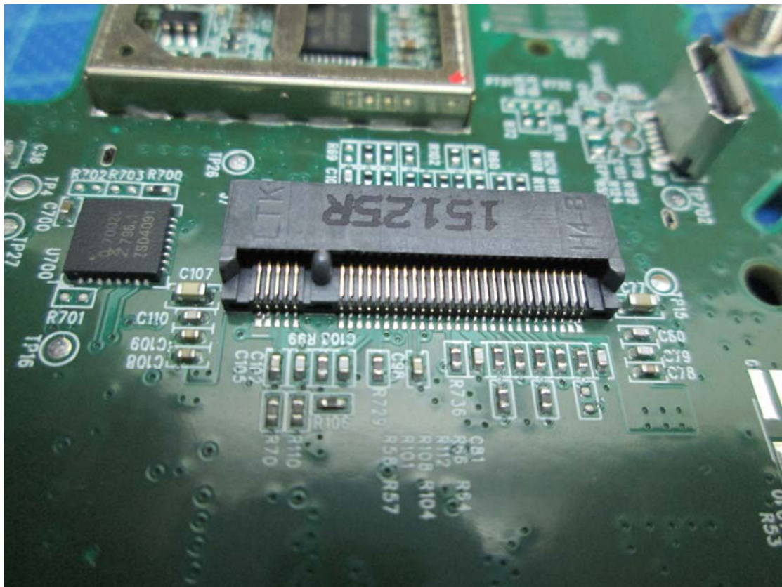
LTE Module
