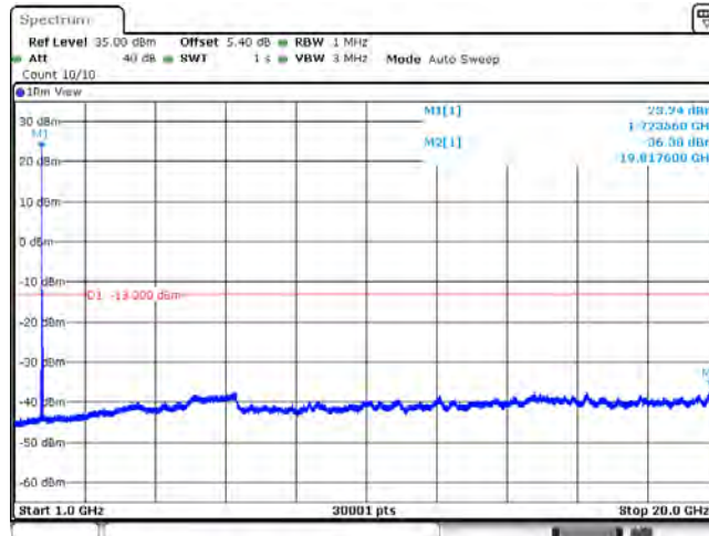
Band4_20MHz_QPSK_20175_1RB#0
