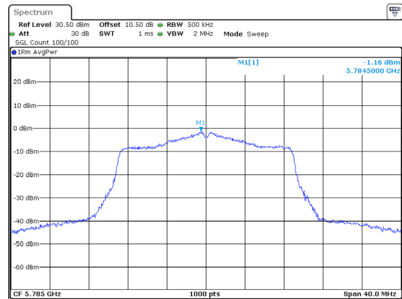
802.11ac20_5785MHz_Chain 1
