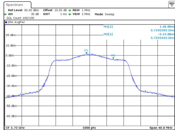
802.11ac20_5720MHz_Chain 1
