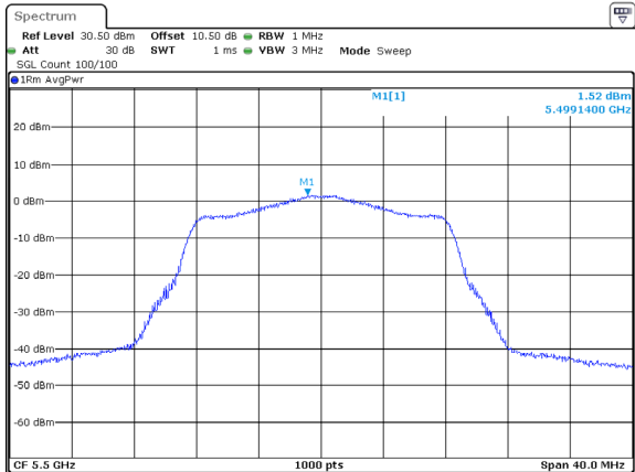
802.11a_5500MHz_Chain 2
