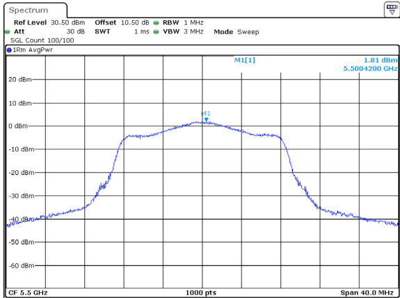
802.11a_5500MHz_Chain 1
