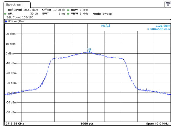
802.11ac20_5580MHz_Chain1
