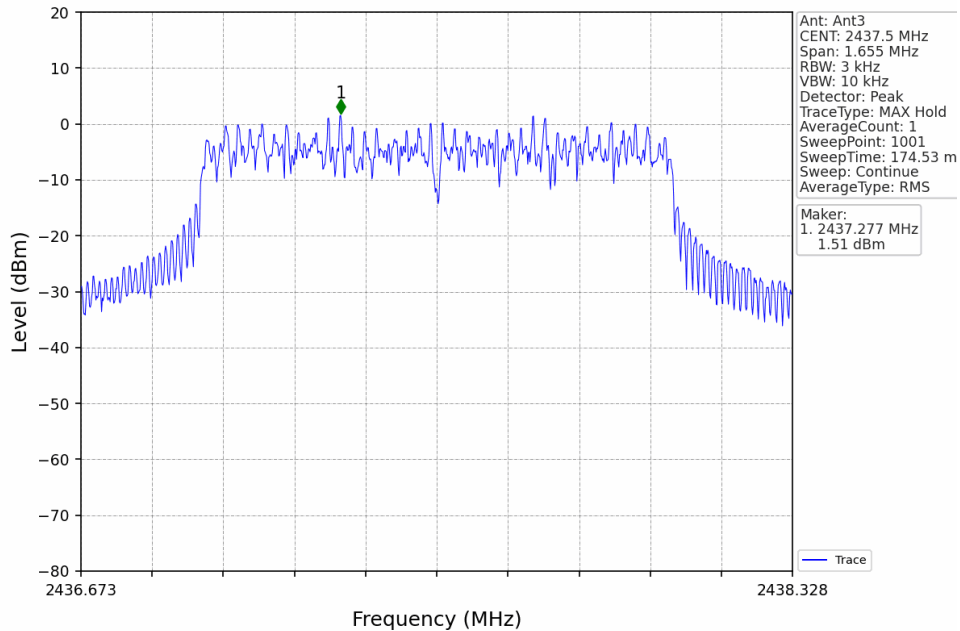
1.4M_MCH_2437.5MHz_MIMO_NTNV
