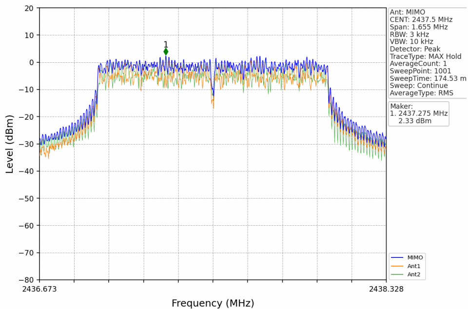
1.4M_MCH_2437.5MHz_MIMO_NTNV
