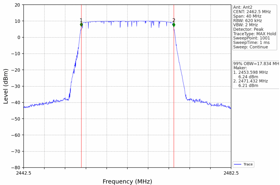
20M_HCH_2462.5MHz_Ant2_NTNV
