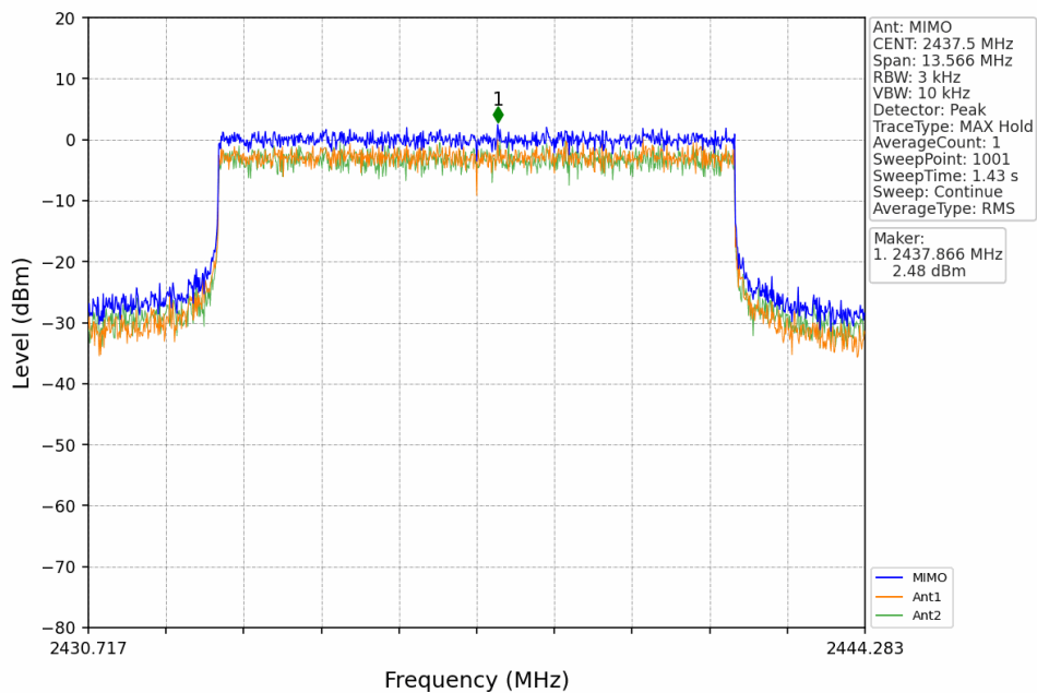
10M_MCH_2437.5MHz_MIMO_NTNV
