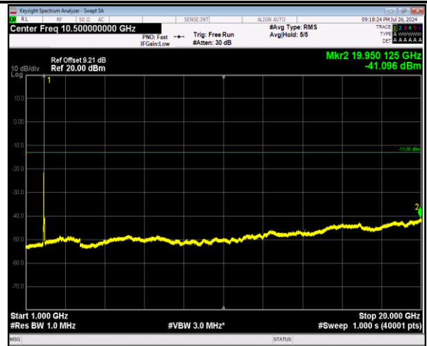
2-2-20MHz-20MHz-64QAM-64QAM-18801-18999-1RB#99- ORB#0-1000~20000MHz-PASS
