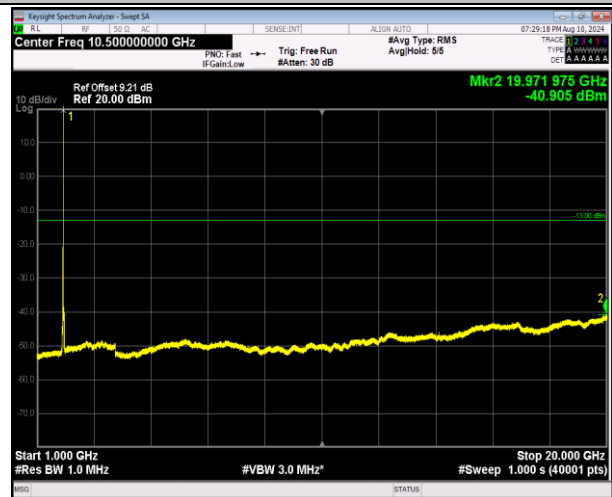
2-2-20MHz-20MHz-16QAM-16QAM-18801-18999-1RB#99- ORB#0-1000~20000MHz-PASS
