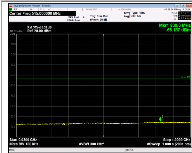
2-2-20MHz-20MHz-QPSK-QPSK-18801-18999-1RB#99-99- 0RB#0-30~1000MHz-PASS
