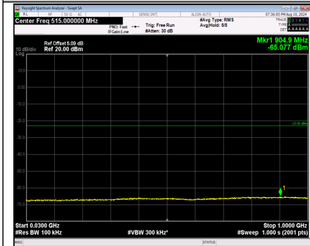
2-2-20MHz-20MHz-QPSK-QPSK-18902-19100-100RB#0- -100RB#0-30~1000MHz-PASS
