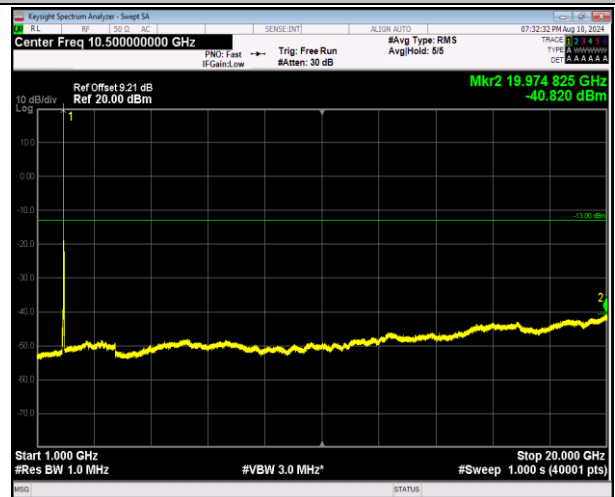
2-2-20MHz-20MHz-QPSK-QPSK-18902-19100-1RB#0-ORB #0-1000~20000MHz-PASS
