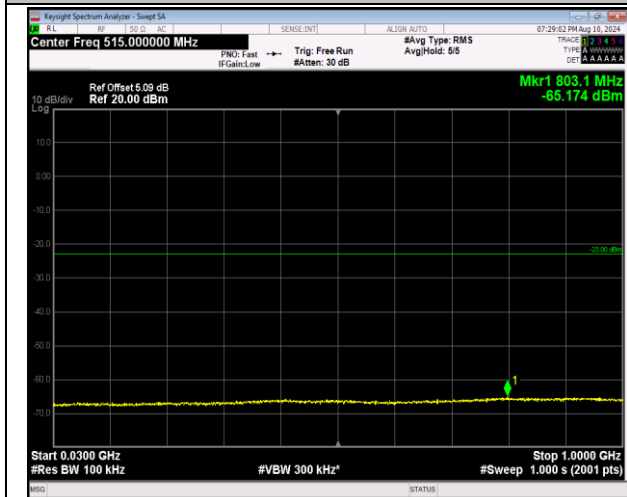
2-2-20MHz-20MHz-16QAM-16QAM-18801-18999-1RB#9 9-ORB#0-30~1000MHz-PASS
