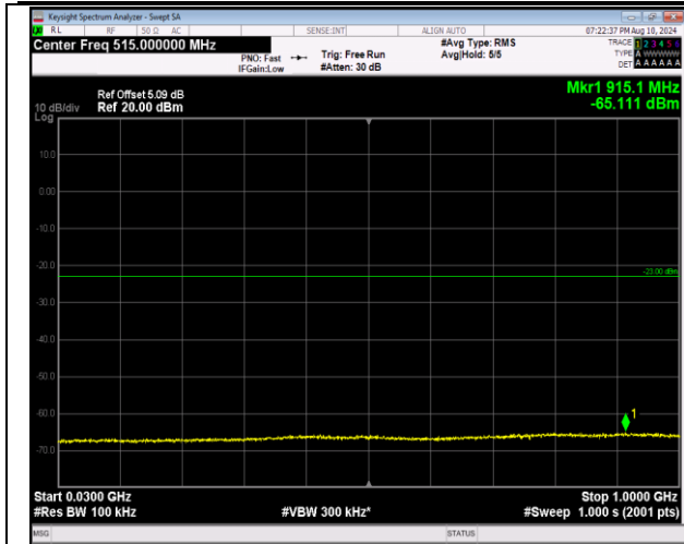
2-2-20MHz-20MHz-16QAM-16QAM-18700-18898-1RB#0 -ORB#0-30~1000MHz-PASS
