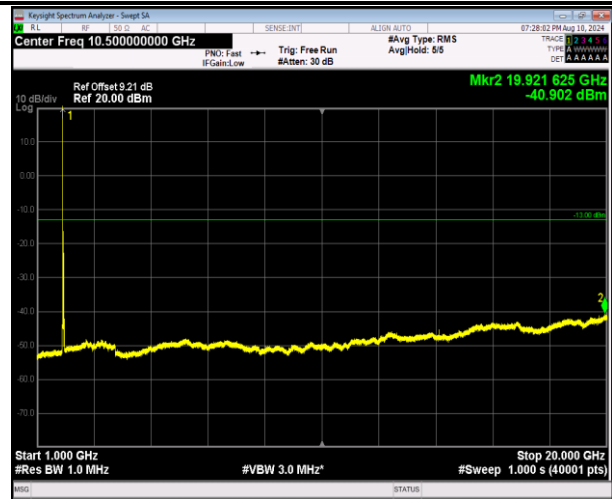
2-2-20MHz-20MHz-16QAM-16QAM-18801-18999-1RB#0-0 RB#0-1000~20000MHz-PASS
