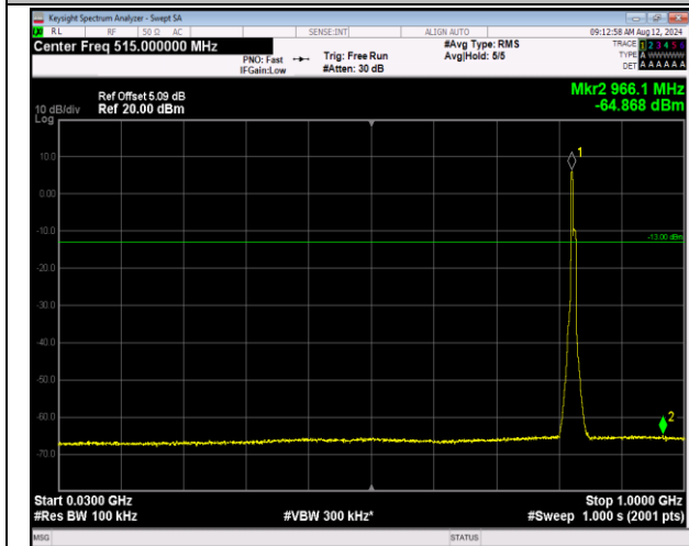
5-5-3MHz-5MHz-QPSK-QPSK-20416-20455-15RB#0-25 RB#0-30~1000MHz-PASS
