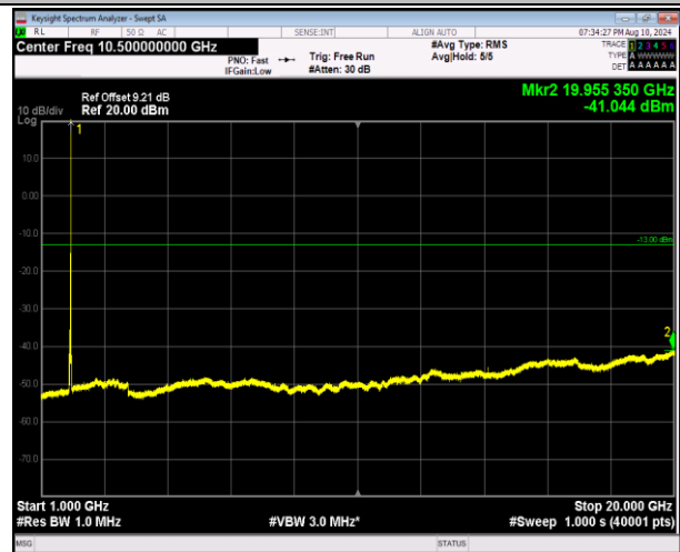
2-2-20MHz-20MHz-16QAM-16QAM-18902-19100-1RB#99- 0RB#0-1000~20000MHz-PASS
