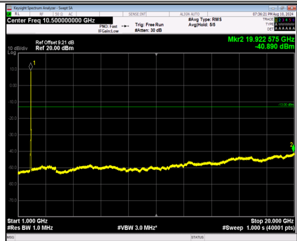
2-2-20MHz-20MHz-QPSK-QPSK-18902-19100-100RB#0-1 00RB#0-1000~20000MHz-PASS
