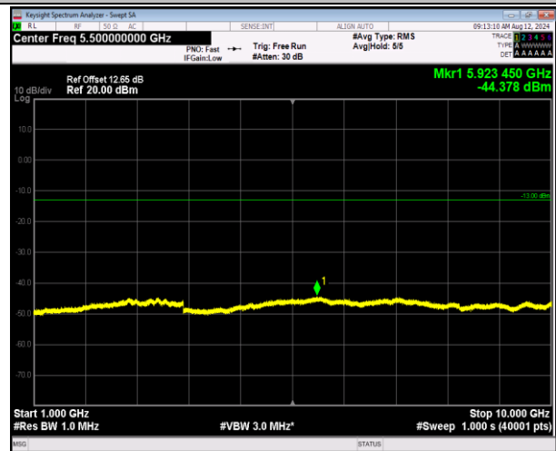
5-5-3MHz-5MHz-QPSK-QPSK-20416-20455-15RB#0-25RB #0-1000~10000MHz-PASS
