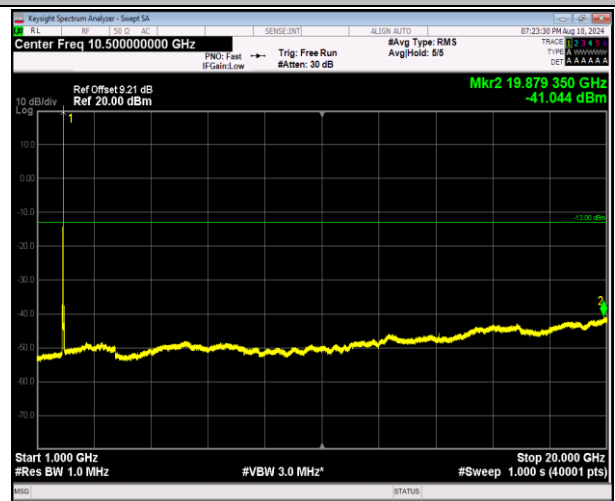
2-2-20MHz-20MHz-QPSK-QPSK-18700-18898-1RB#99-0R B#0-1000~20000MHz-PASS
