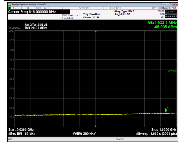
2-2-20MHz-20MHz-QPSK-QPSK-18700-18898-1RB#0-1 RB#99-30~1000MHz-PASS
