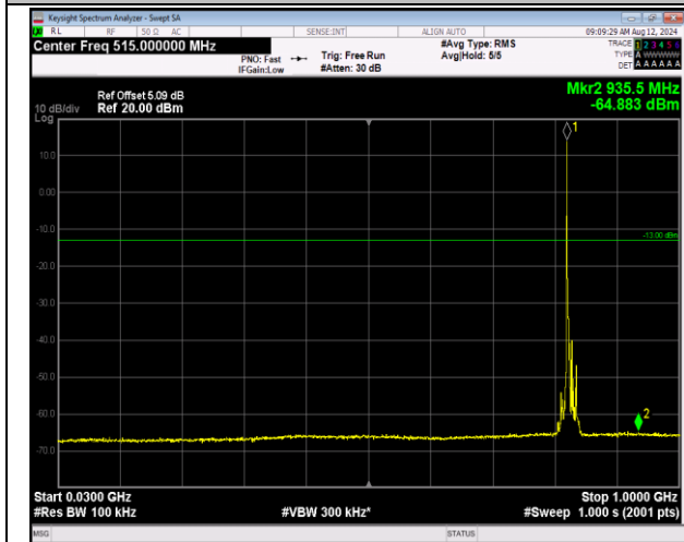
5-5-3MHz-5MHz-QPSK-QPSK-20416-20455-1RB#0-0RB #0-30~1000MHz-PASS
