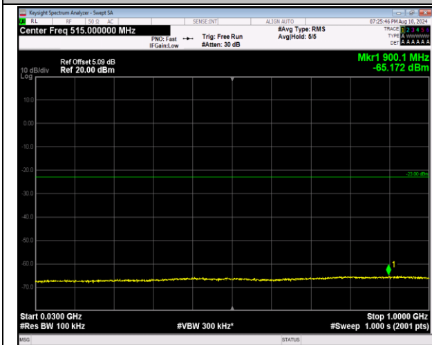
2-2-20MHz-20MHz-QPSK-QPSK-18700-18898-100RB#0 -100RB#0-30~1000MHz-PASS
