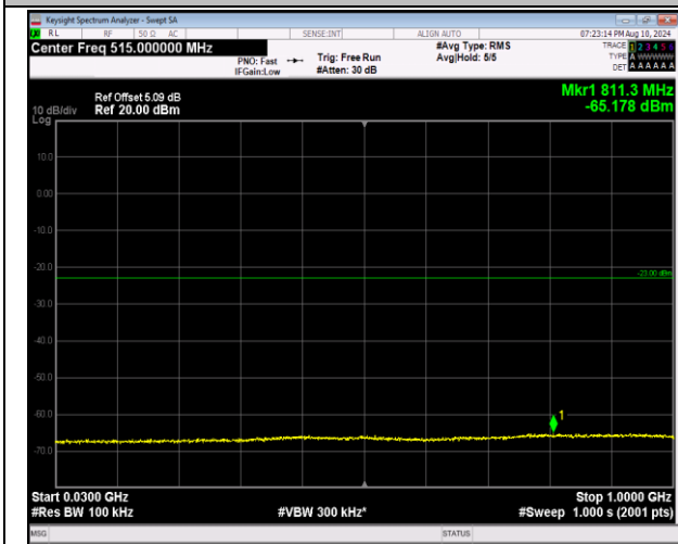
2-2-20MHz-20MHz-QPSK-QPSK-18700-18898-1RB#99-0 ORB#0-30~1000MHz-PASS
