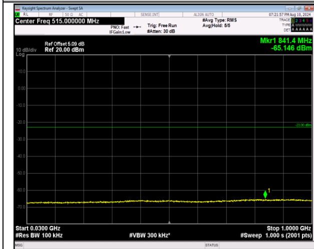
2-2-20MHz-20MHz-QPSK-QPSK-18700-18898-1RB#0-0 RB#0-30~1000MHz-PASS
