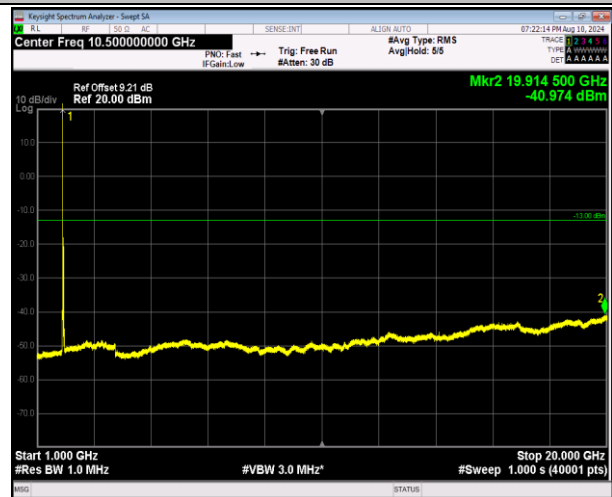
2-2-20MHz-20MHz-QPSK-QPSK-18700-18898-1RB#0-0RB #0-1000~20000MHz-PASS
