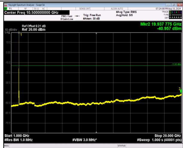
2-2-20MHz-20MHz-16QAM-16QAM-18700-18898-1RB#99- ORB#0-1000~20000MHz-PASS
