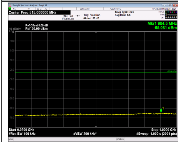
2-2-20MHz-20MHz-QPSK-QPSK-18902-19100-1RB#99-99- 0RB#0-30~1000MHz-PASS
