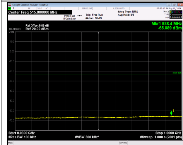
2-2-20MHz-20MHz-QPSK-QPSK-18902-19100-1RB#0-0 RB#0-30~1000MHz-PASS
