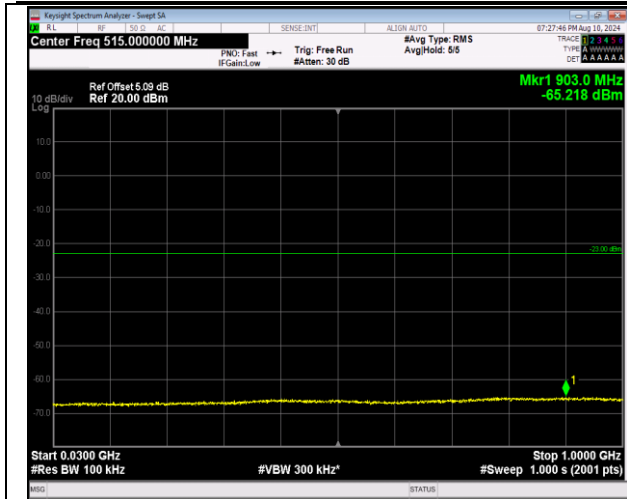
2-2-20MHz-20MHz-16QAM-16QAM-18801-18999-1RB#0 -ORB#0-30~1000MHz-PASS
