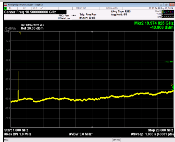
2-2-20MHz-20MHz-QPSK-QPSK-18801-18999-1RB#0-ORB #0-1000~20000MHz-PASS
