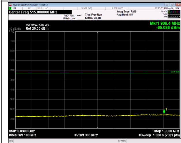
2-2-20MHz-20MHz-16QAM-16QAM-18700-18898-1RB#9 9-ORB#0-30~1000MHz-PASS
