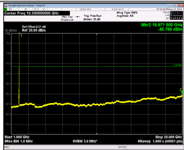
2-2-20MHz-20MHz-QPSK-QPSK-18902-19100-1RB#99-0R B#0-1000~20000MHz-PASS
