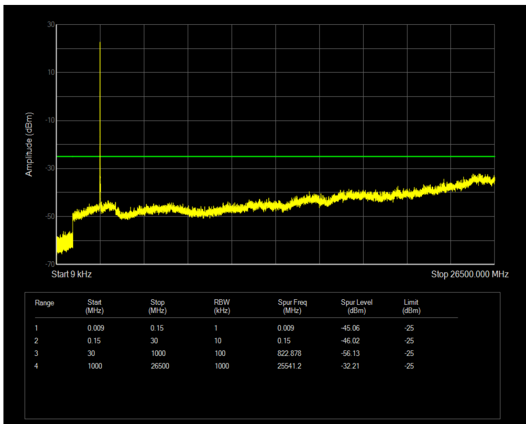
Band41(2555-2655) QPSK BW=10MHz Channel=40290 RB Size=1 Position=#0
