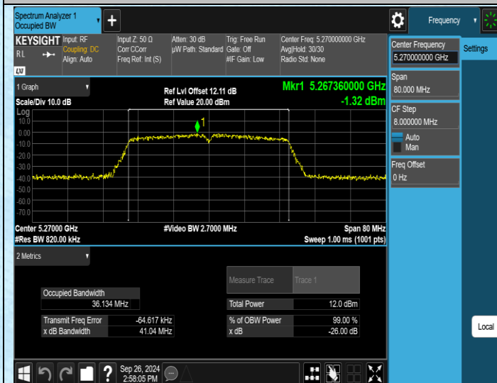
11N40MIMO-Ant1-5270
