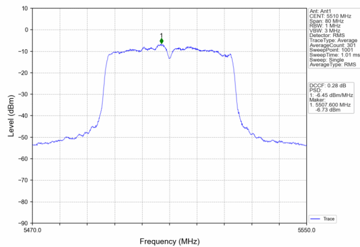
802.11n(HT40) MCH_5550MHz_AntA_NTNV
