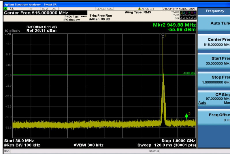
Band5-5MHz-QPSK-20425-1RB#0-30~1000MHz
