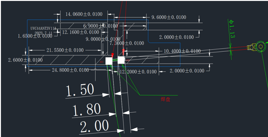
天线尺寸/ANT Size
