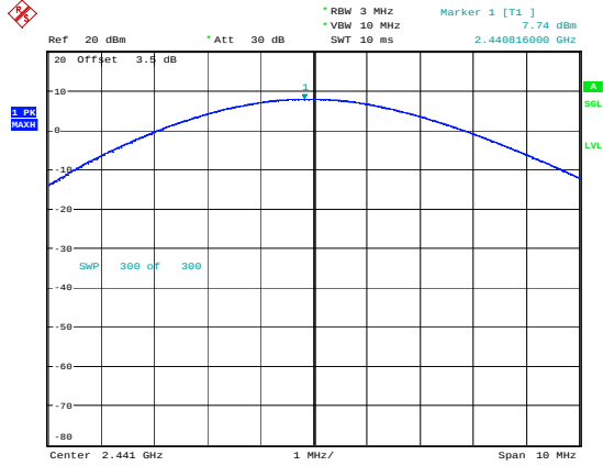
\pi/4 -DQPSK_Middle 7.74dBm
