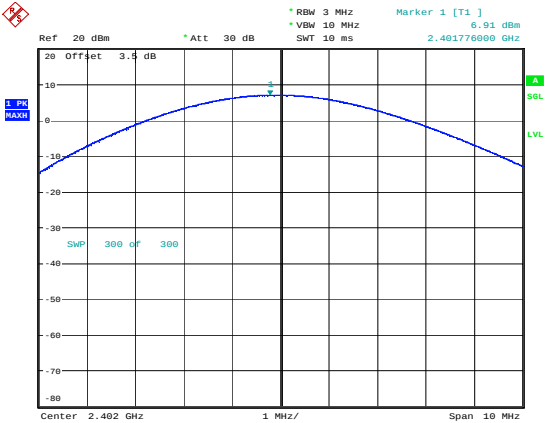
\pi/4 -DQPSK_Low 6.91dBm
