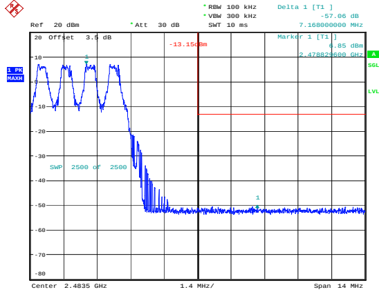
GFSK_Hopping_Upper 57.06dB
