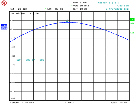
\pi/4 -DQPSK_High 7.80dBm
