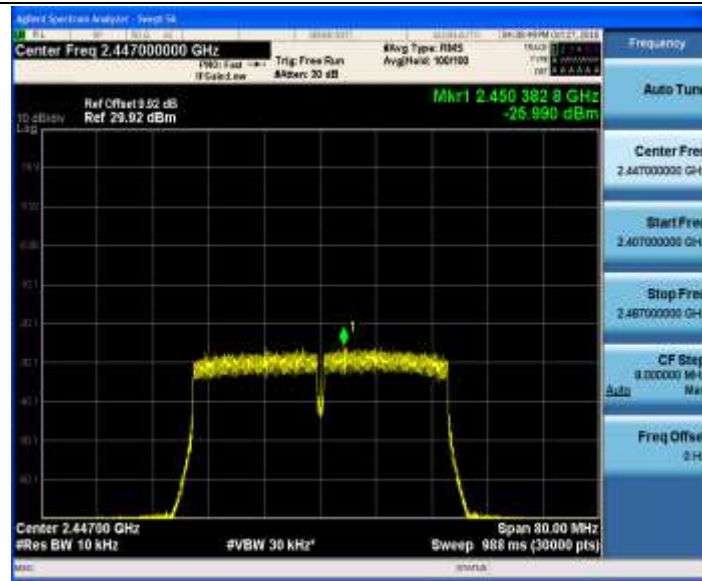
11N40MIMO_Ant2_2447
