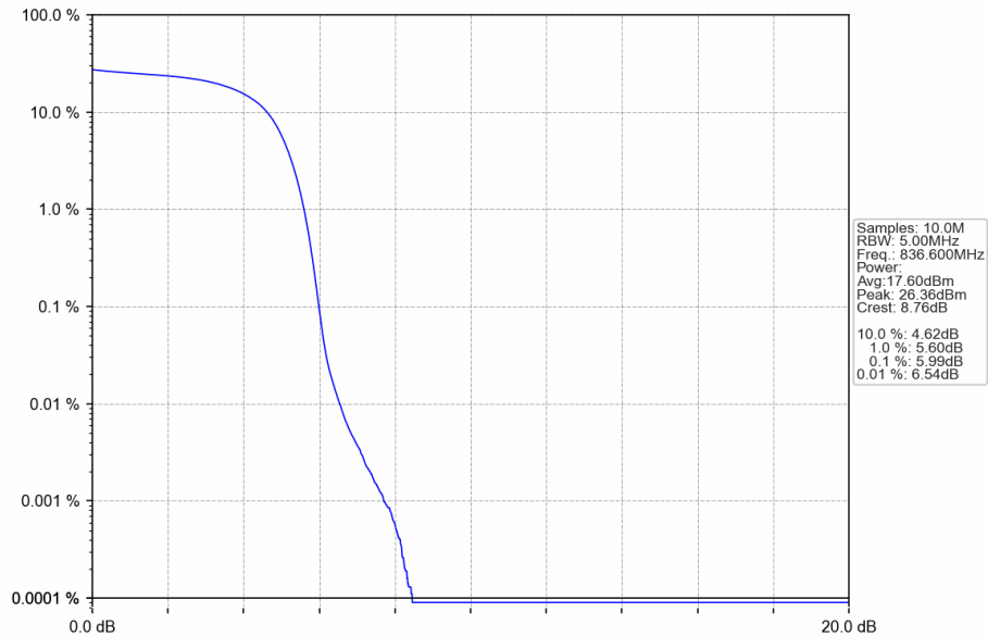
Band5_HSUPA_MCH_836.6MHz_Subtest 1_NTNV
