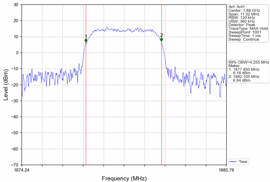
Band2_HSUPA_MCH_1880MHz_Subtest 1_NTNV
