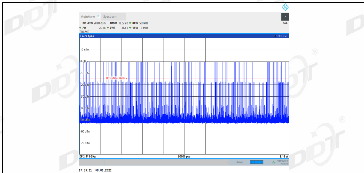
3DH1_Ant1_Hop
