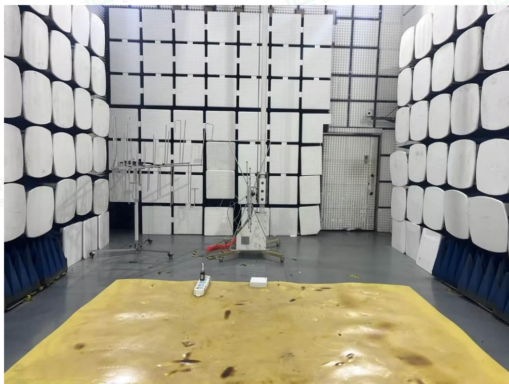
Fig. 2 (30MHz-1GHz)
