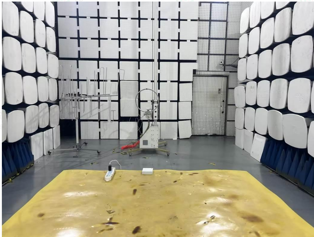
Fig. 1(Below 30MHz)
