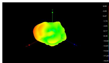
2500MHz
