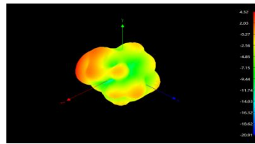
2400MHz
