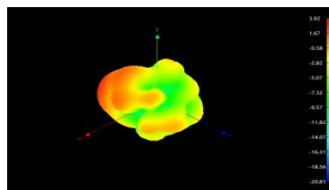
2450MHz
