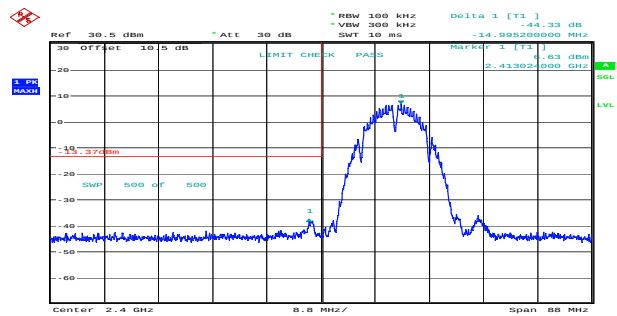
b_2412MHz_Chain 1 44.33dB
