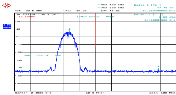
b_2462MHz_Chain 0 47.48dB
