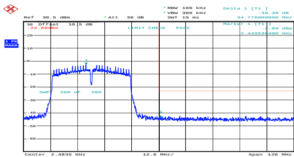
n40_2452MHz_Chain 0 39.39dB
