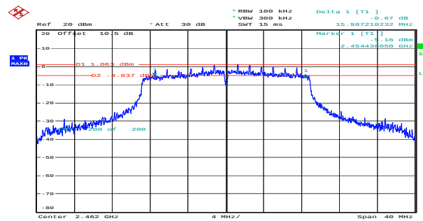
n20_2462MHz_Chain 1 15.987MHz
