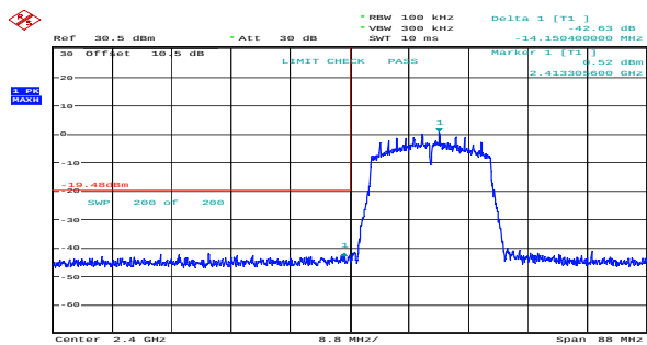
n20_2412MHz_Chain 0 42.63dB
