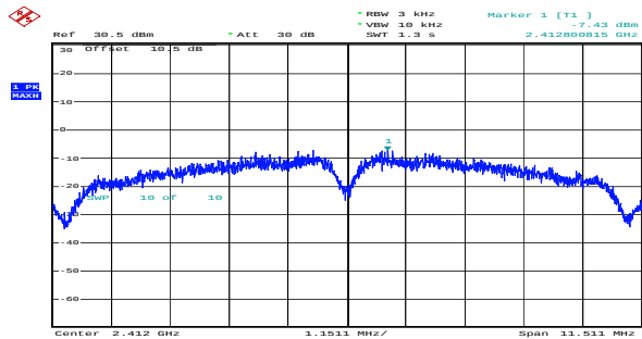
b_2412MHz_Chain 0 -7.43dBm/3kHz
