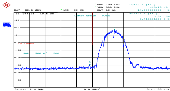
b_2412MHz_Chain 0 45.78dB
