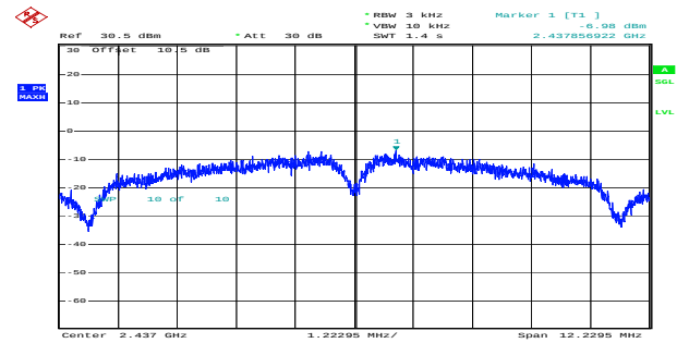
b_2437MHz_Chain 1 -6.98dBm/3kHz
