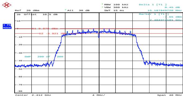
n20_2412MHz_Chain 0 15.188MHz
