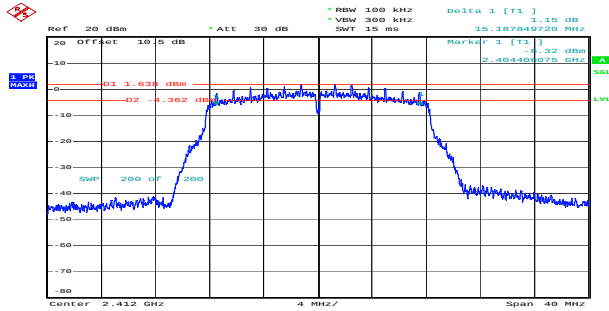
g_2412MHz_Chain 0 15.188MHz
