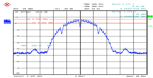
b_2437MHz_Chain 1 8.153MHz
