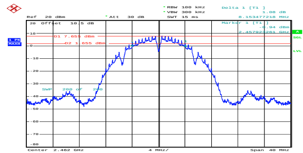
b_2462MHz_Chain 1 8.153MHz
