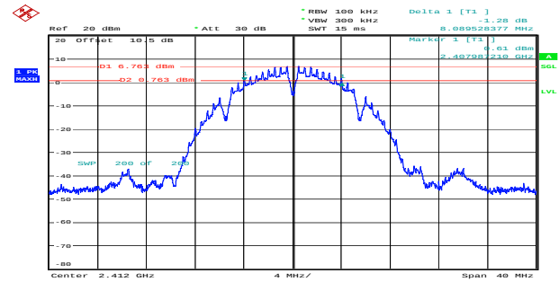
b_2412MHz_Chain 1 8.090MHz
