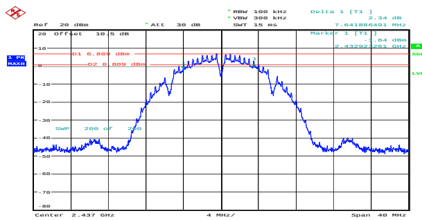
b_2437MHz_Chain 0 7.642MHz
