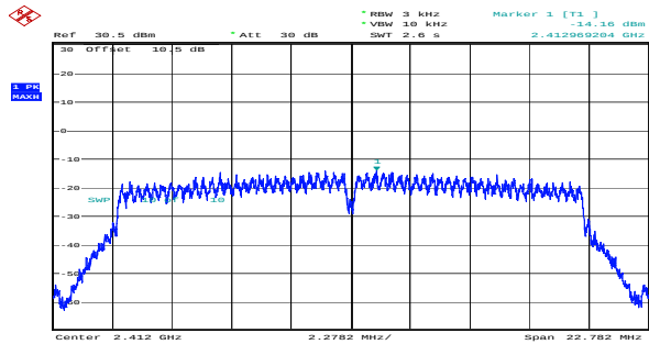
n20_2412MHz_Chain 0 -14.16dBm/3kHz
