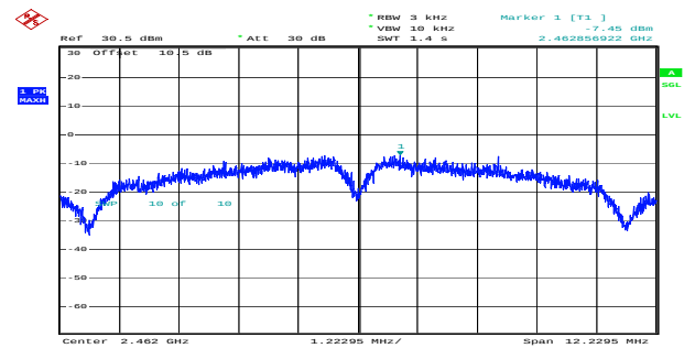
b_2462MHz_Chain 1 -7.45dBm/3kHz
