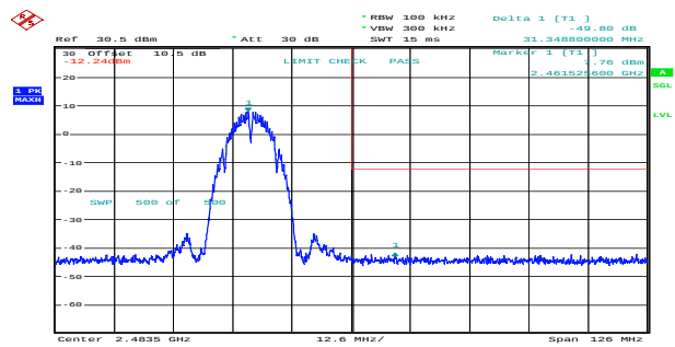
b_2462MHz_Chain 1 49.80dB
