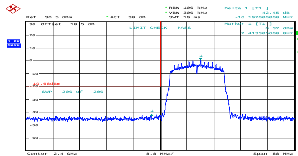
n20_2412MHz_Chain 1 42.45dB
