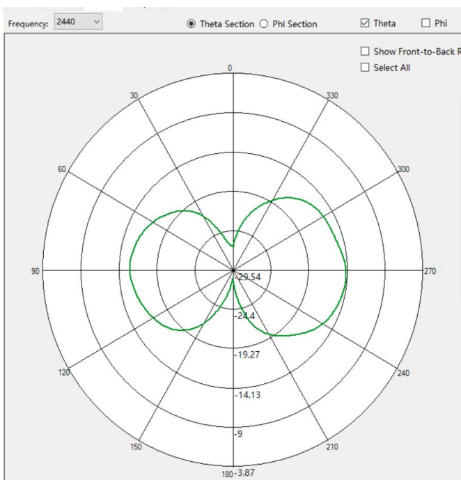
Vertical:2440MHz
