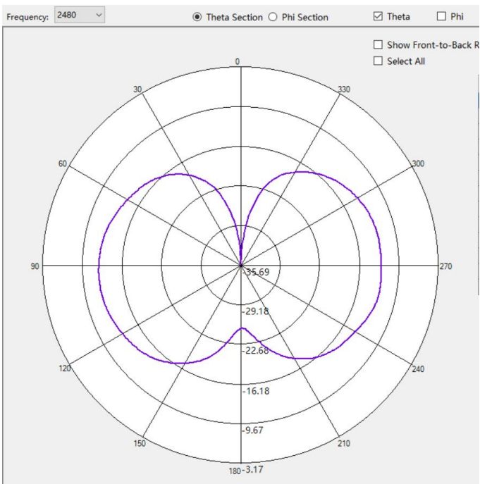
Vertical:2480MHz
