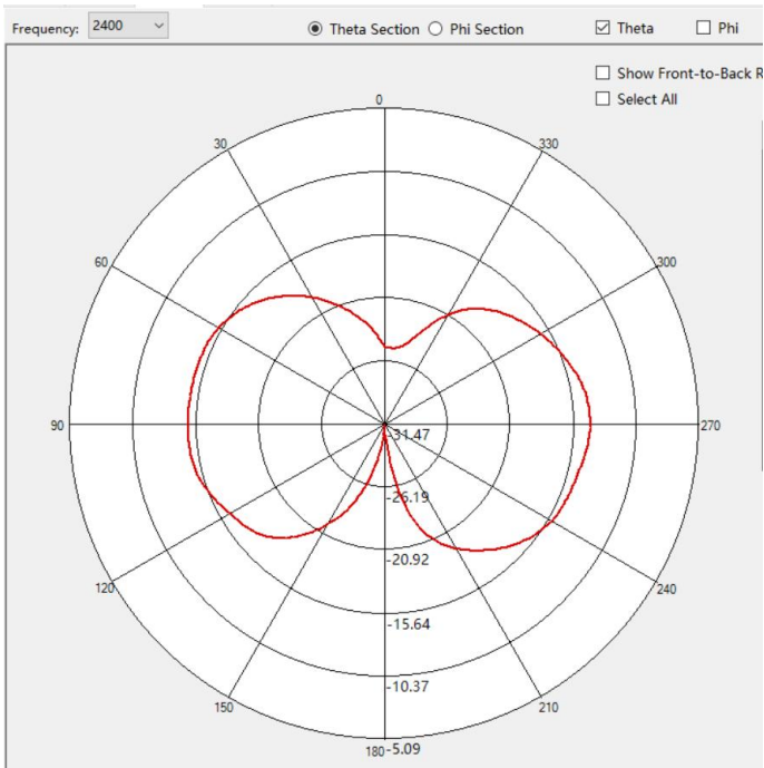
Vertical:2400MHz
