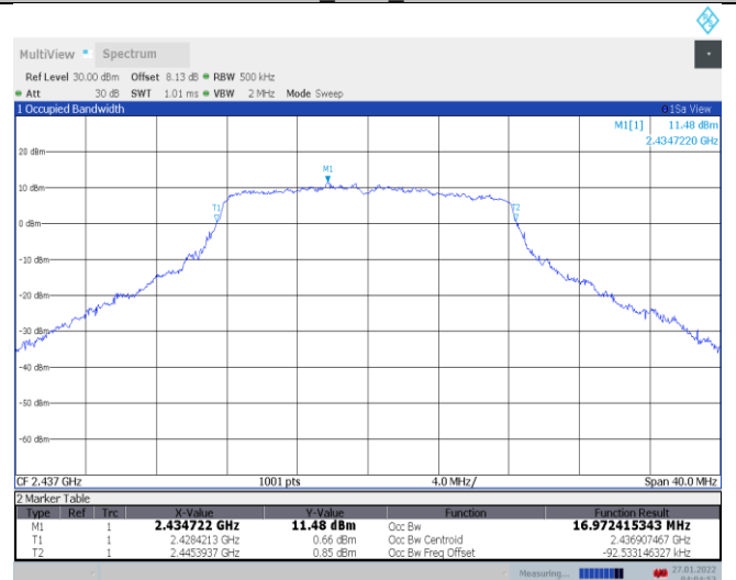
11G_Ant1_2437
