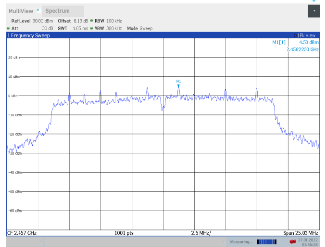
11N20SISO_Ant1_2457
