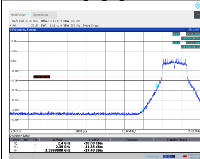
11G_Ant1_Low_2417
