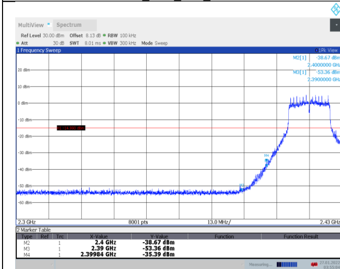
11G_Ant1_Low_2422
