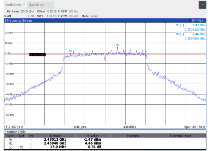
11G_Ant1_2457
