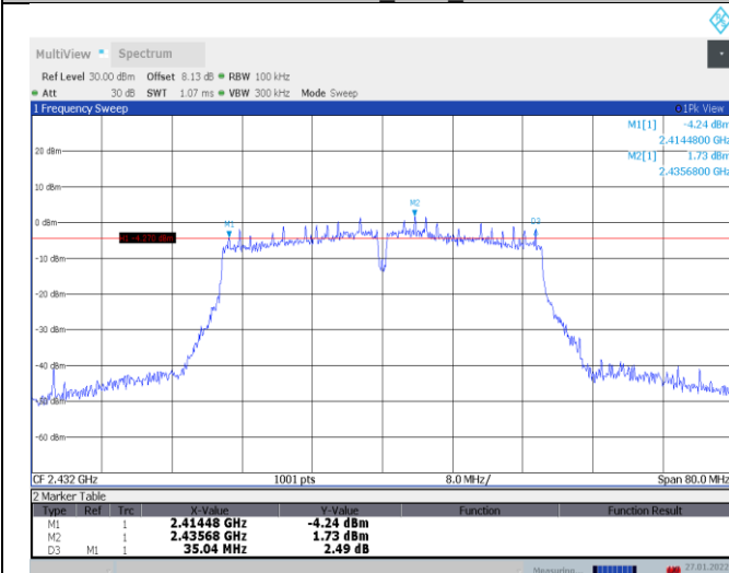
11N40SISO_Ant1_2432
