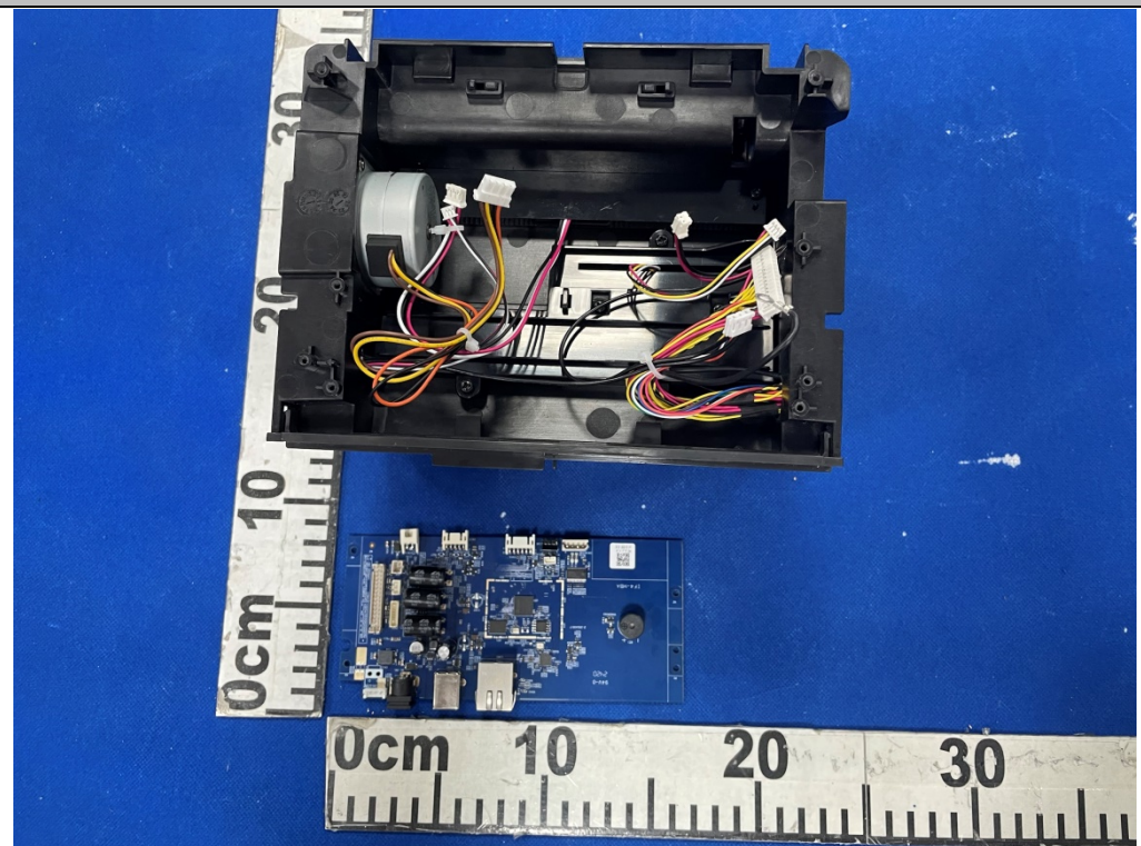
EUT Photo
