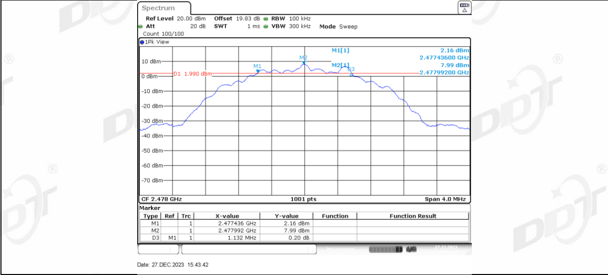
BLE_2M_Ant1_2478
