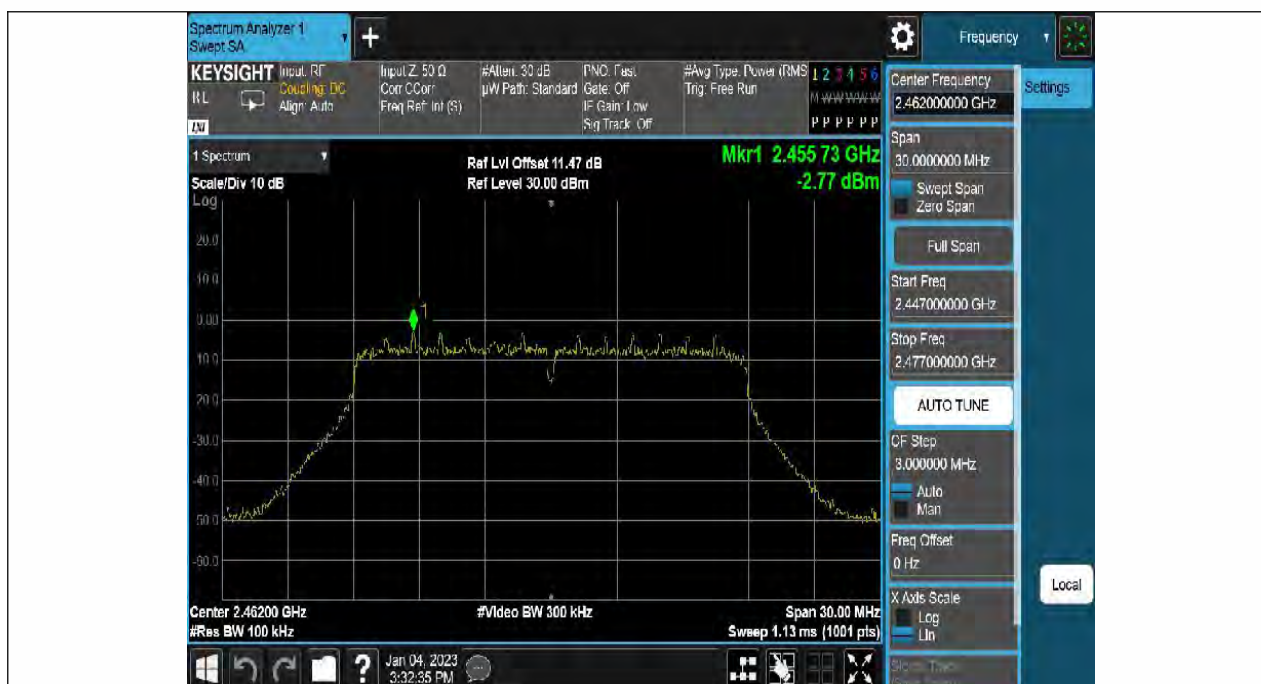
11N20SISO-Ant1-2462-0~Reference--2.77
