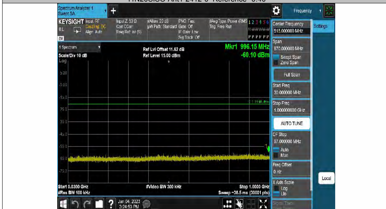
11N20SISO-Ant1-2412-30~1000--0.40
