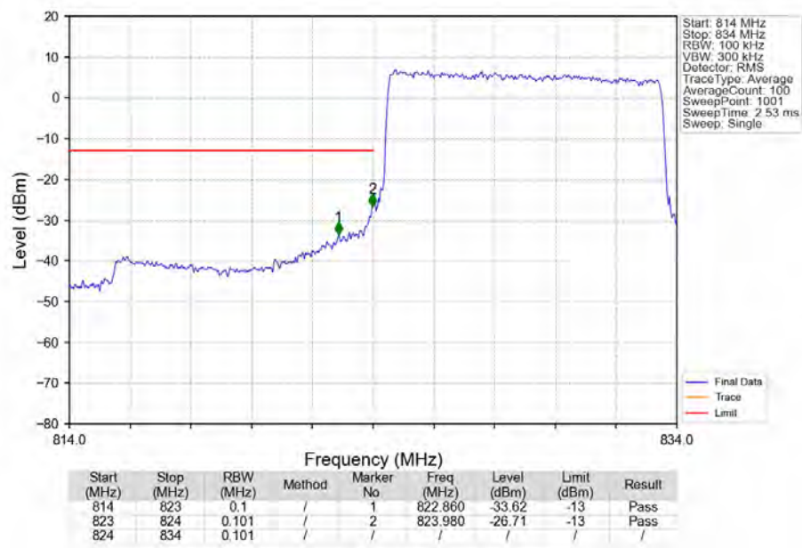
Band5_10MHz_QPSK_LCH_829MHz_RB_50_0_NTNV
