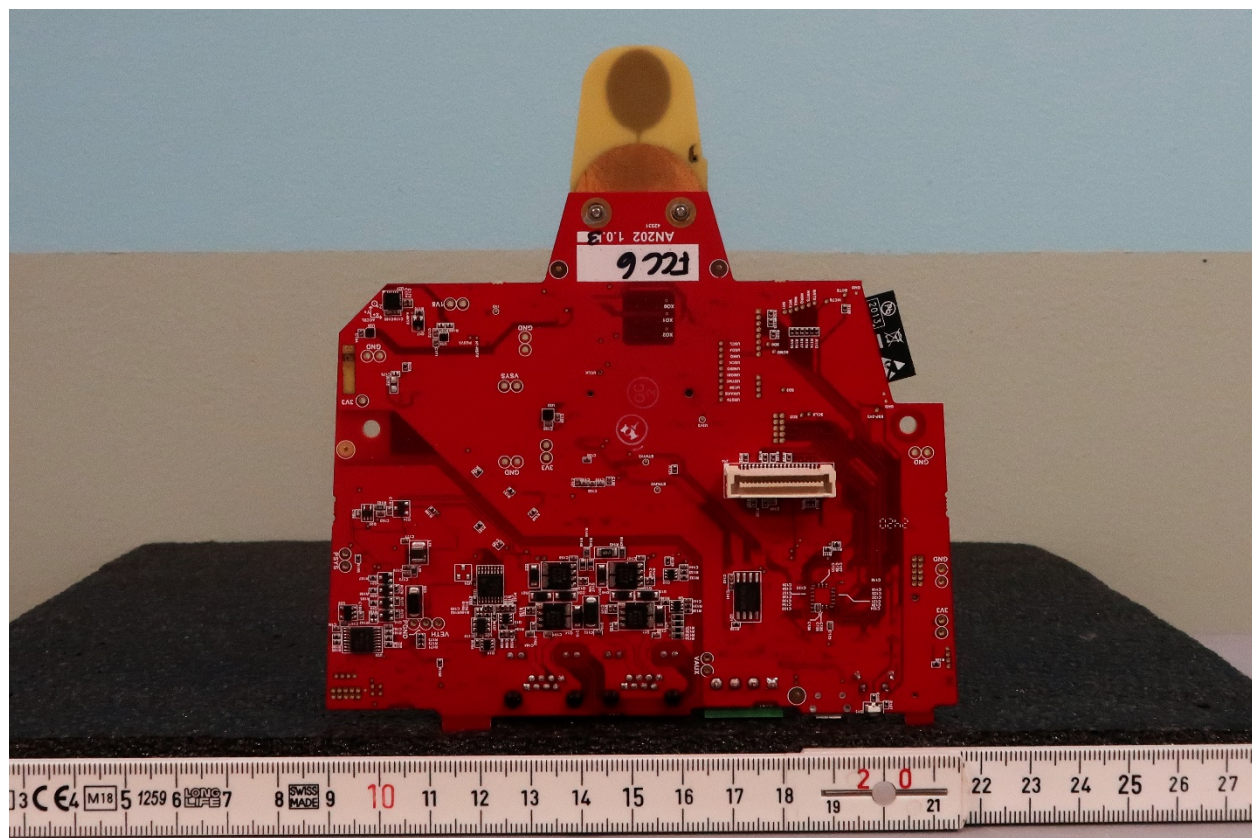
Module Rear
