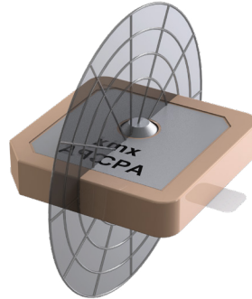
YZ-Plane Gain
