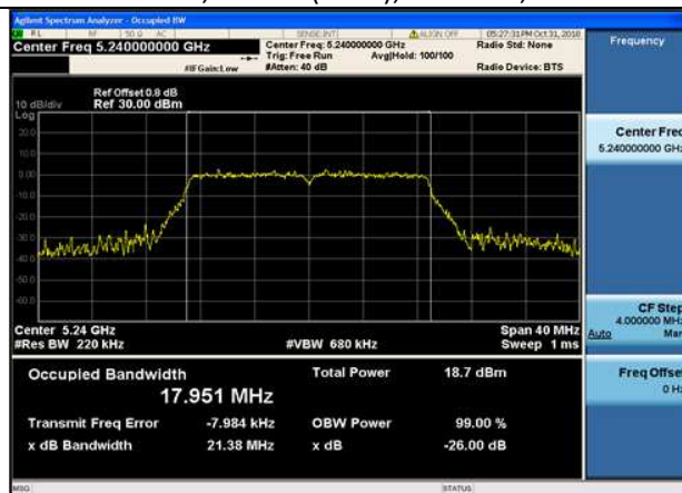
U-NII-1,802.11n(HT20),5240MHz,Ant0
