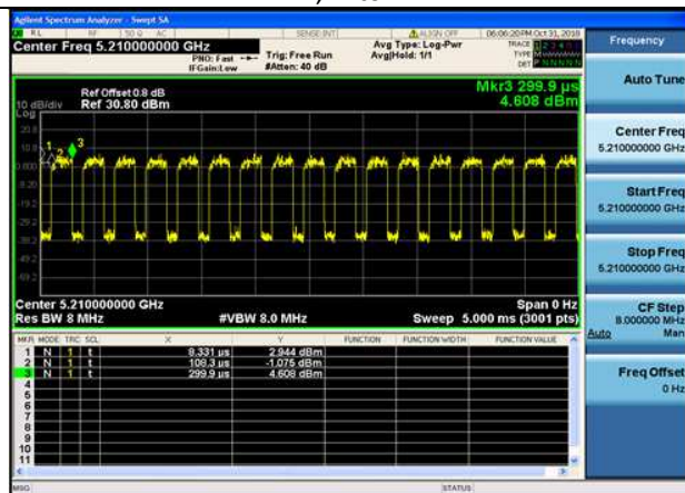
U-NII-1,802.11ac(VHT80),5210MHz ,Ant0
