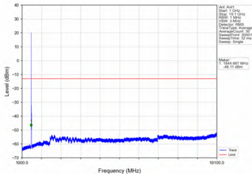
n2 30kHz SISO NTN 20MHz DFT-s-OFDM QPSK 1860MHz Edge 1RB Left
