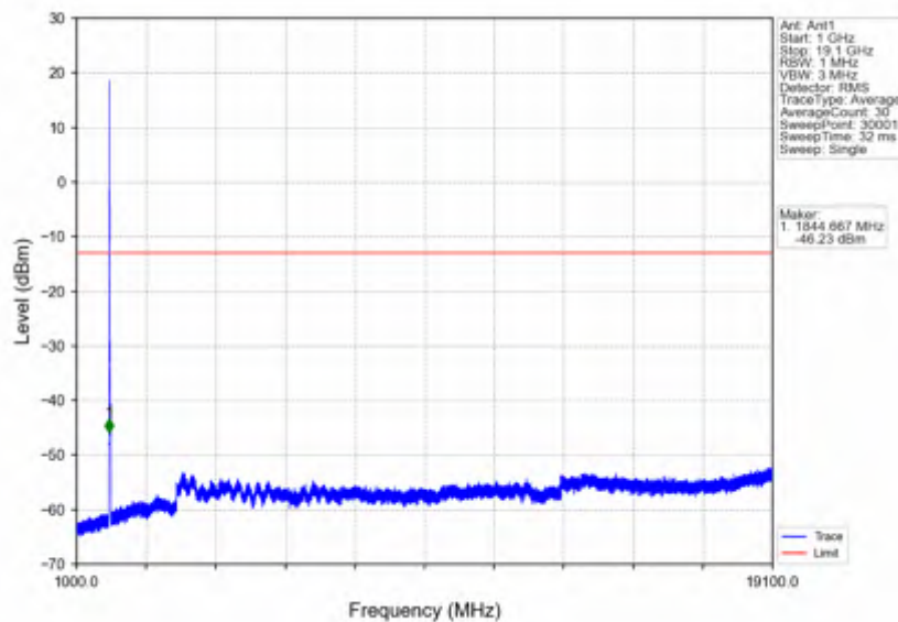
n2 30kHz SISO NTV 20MHz CP-OFDM QPSK 1880MHz Edge 1RB Left
