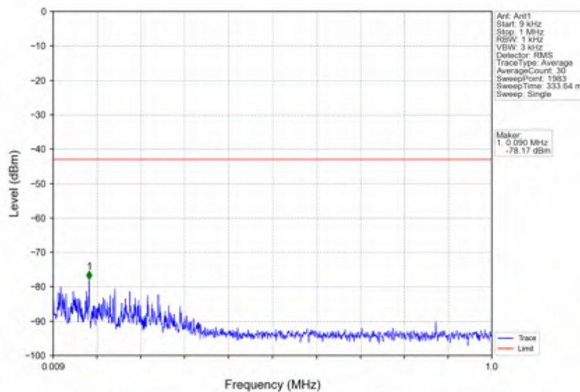
n2_30kHz_SISO_NTNV_20MHz_CP-OFDM QPSK_1860MHz_Edge_1RB_Left
