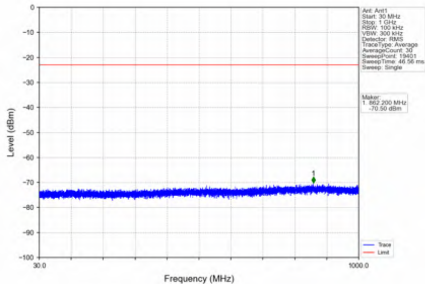
n2_30kHz_SISO_NTNV_20MHz_DFT-s-OFDM QPSK_1900MHz_Inner_1RB_Right
