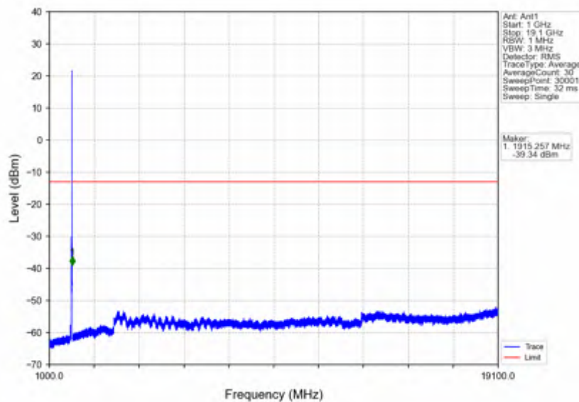
n2_30kHz_SISO_NTNV_20MHz_DFT-s-OFDM QPSK_1860MHz_Edge_1RB_Left
