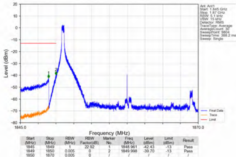
n2_30kHz_SISO_NTNV_20MHz_DFT-s-OFDM QPSK_1860MHz_Edge_1RB_Left
