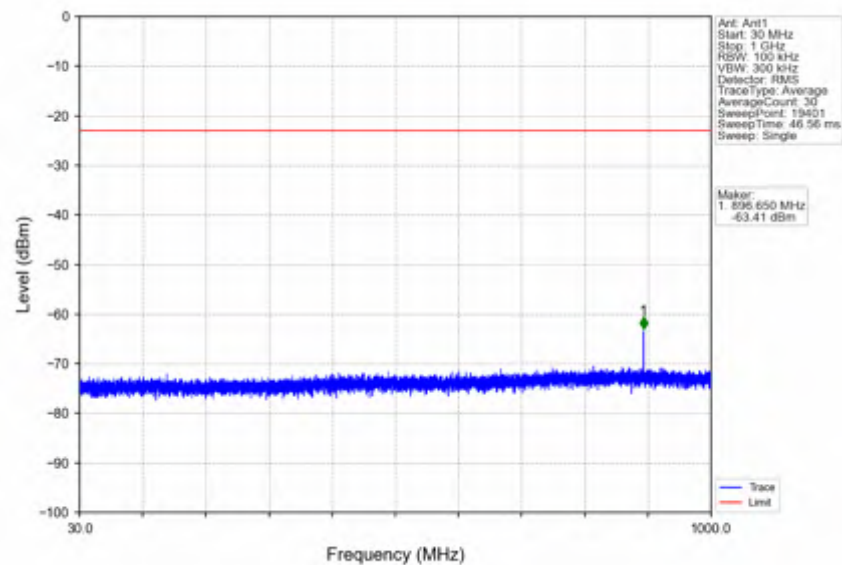
n2 30kHz SISO NTN 20MHz CP-OFDM QPSK 1880MHz Edge 1RB Left
