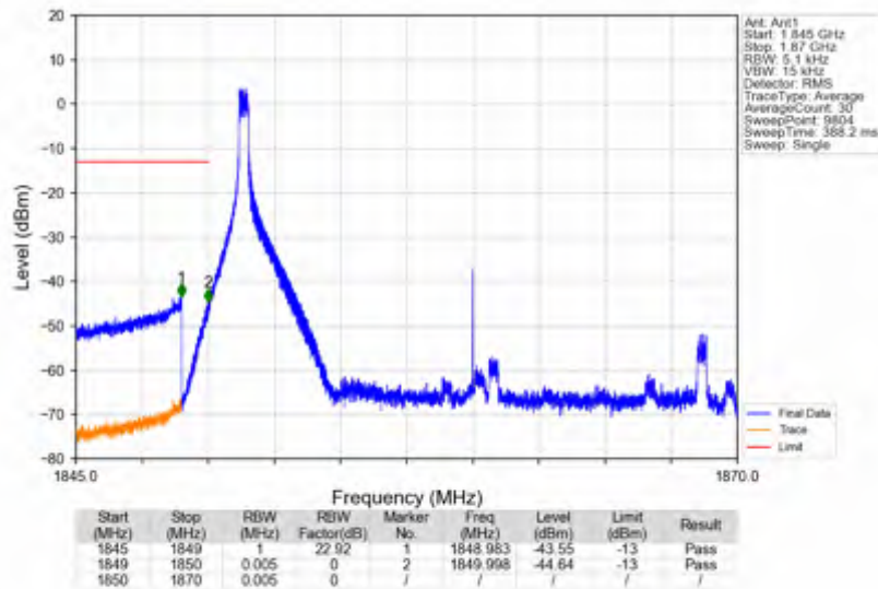
n2_30kHz_SISO_NTNV_20MHz_DFT-s-OFDM_QPSK_1860MHz_Inner_1RB_Left
