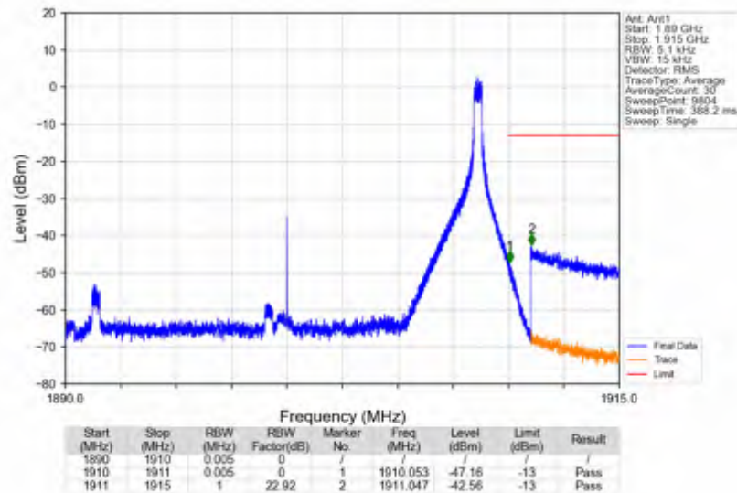
n2_30kHz_SISO_NTNV_20MHz_CP-OFDM_QPSK_1900MHz_Inner_1RB_Right
