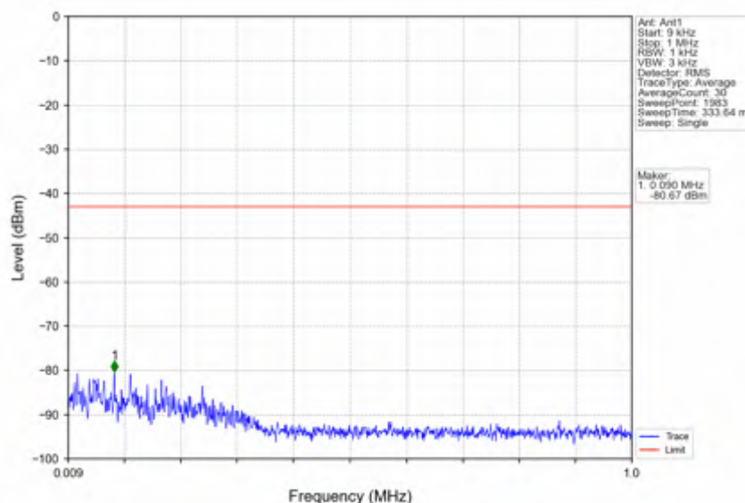
n2 30kHz SISO NTN 15MHz CP-OFDM QPSK 1857.5MHz Edge 1RB Left
