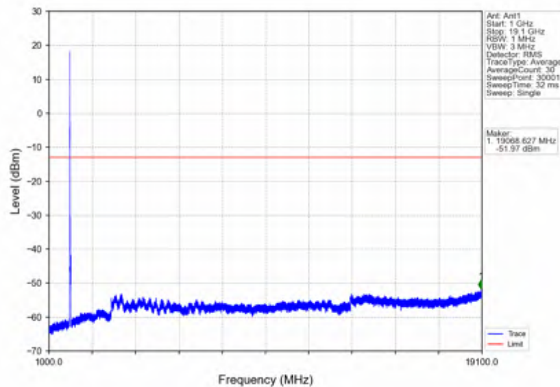
n2 30kHz SISO NTN 20MHz CP-OFDM QPSK 1880MHz Edge 1RB Left
