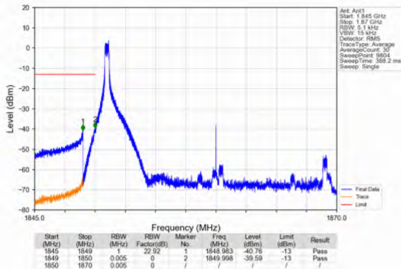
n2_30kHz_SISO_NTNV_20MHz_DFT-s-OFDM_PI/2_BPSK_1860MHz_Edge_1RB_Left
