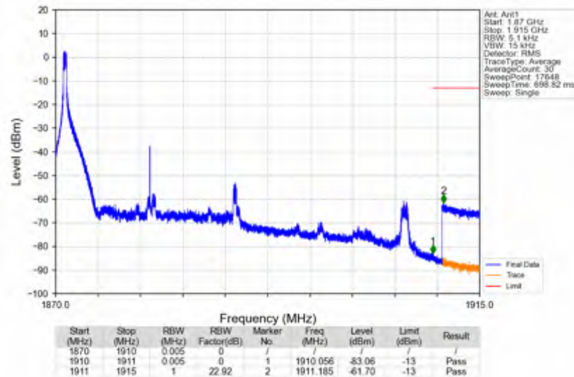
n2_30kHz_SISO_NTNV_20MHz_DFT-s-OFDM QPSK_1880MHz_Edge_1RB_Left
