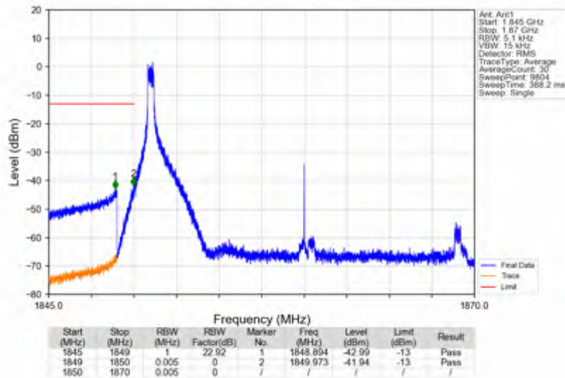
n2_30kHz_SISO_NTNV_20MHz_CP-OFDM QPSK_1860MHz_Edge_1RB_Left
