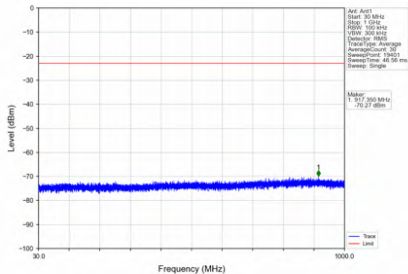
n2 30kHz SISO NTN 20MHz DFT-s-OFDM QPSK 1860MHz Edge 1RB Left
