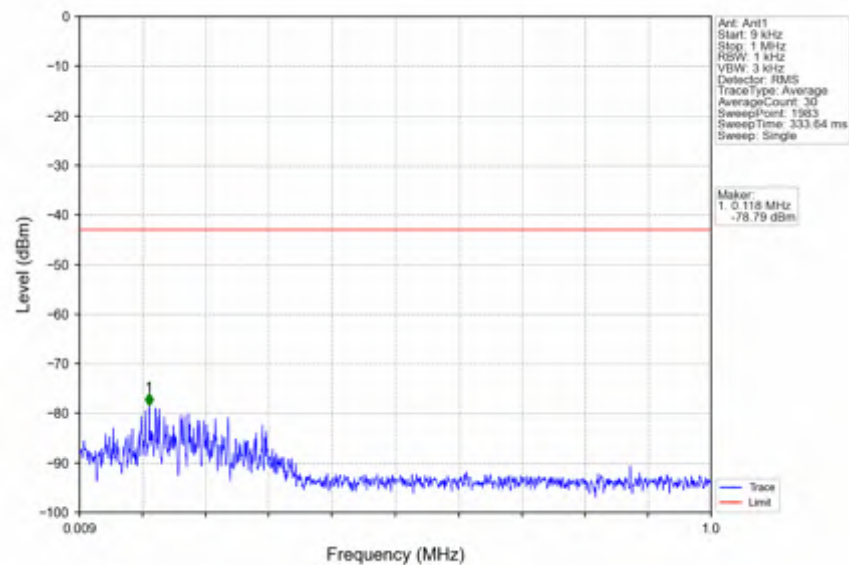
n2_30kHz_SISO_NTNV_20MHz_DFT-s-OFDM_QPSK_1860MHz_Inner_1RB_Left
