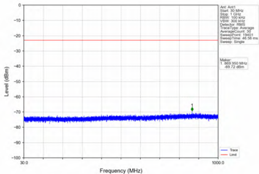
n2_30kHz_SISO_NTNV_20MHz_CP-OFDM QPSK_1860MHz_Edge_1RB_Left
