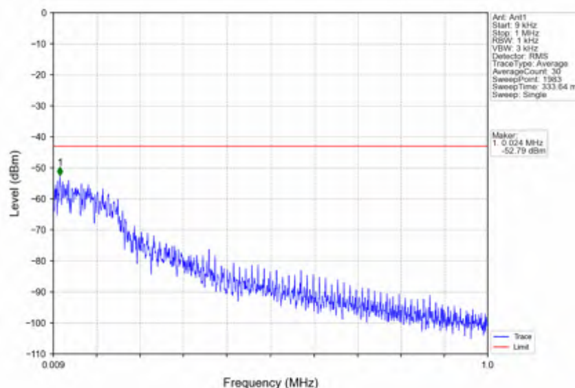
n5 15kHz SISO NTV 5MHz CP-OFDM QPSK 826.5MHz Edge 1RB Left
