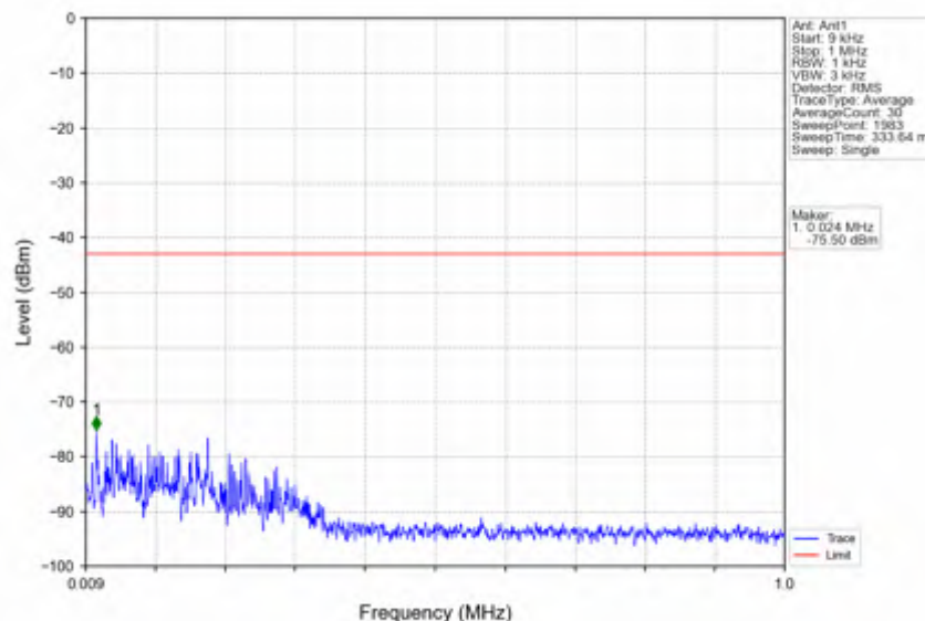
n2_30kHz_SISO_NTNV_20MHz_CP-OFDM_QPSK_1900MHz_Inner_1RB_Right
