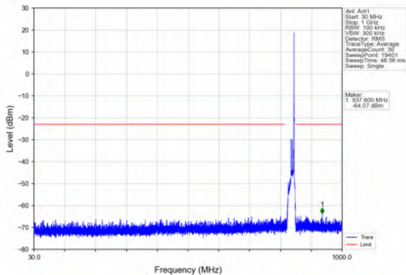
n5 15kHz SISO NTV 10MHz CP-OFDM QPSK 844MHz Edge 1RB Right
