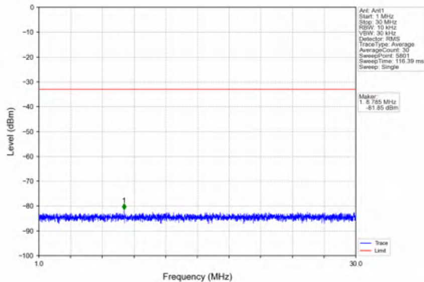
n2_30kHz_SISO_NTNV_20MHz_DFT-s-OFDM PI/2 BPSK_1860MHz_Edge_1RB_Left
