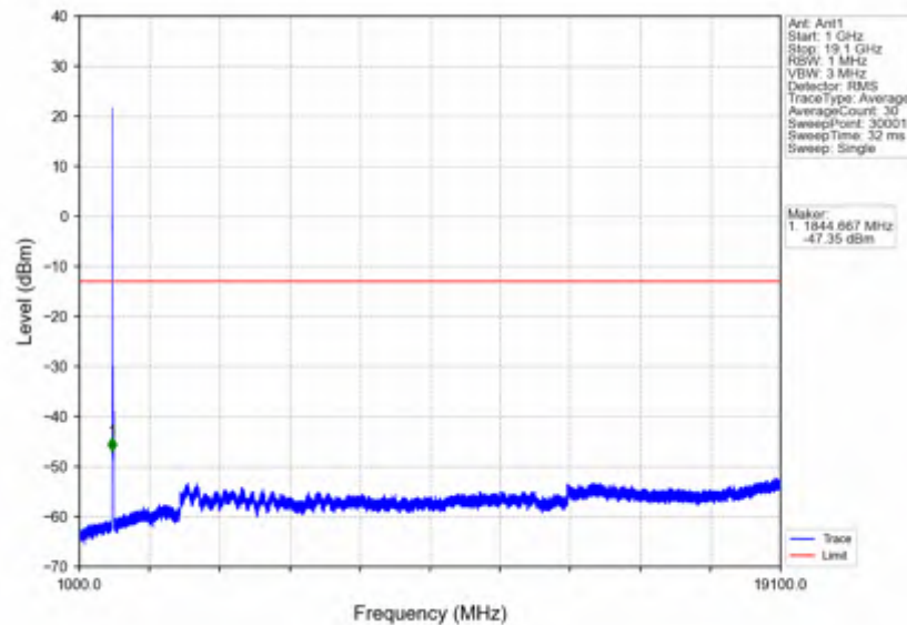
n2_30kHz_SISO_NTNV_20MHz_DFT-s-OFDM QPSK_1860MHz_Inner_1RB_Left
