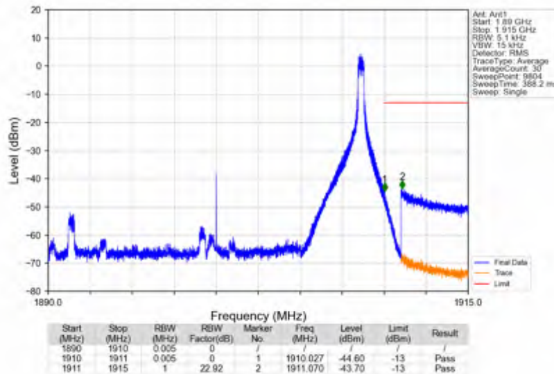
n2_30kHz_SISO_NTNV_20MHz_DFT-s-OFDM QPSK_1900MHz_Inner_1RB_Right
