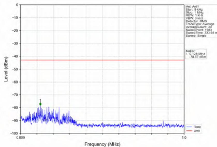
n2_30kHz_SISO_NTNV_20MHz_DFT-s-OFDM QPSK_1880MHz_Edge_1RB_Left
