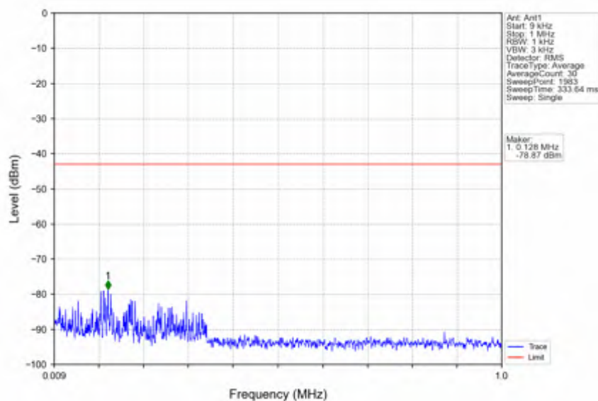
n2_30kHz_SISO_NTNV_20MHz_DFT-s-OFDM_PI/2_BPSK_1860MHz_Edge_1RB_Left
