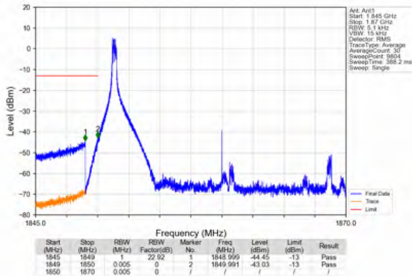
n2_30kHz_SISO_NTNV_20MHz_DFT-s-OFDM PI/2 BPSK_1860MHz_Inner_1RB_Left
