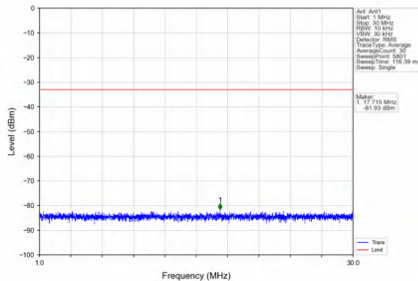
n2_30kHz_SISO_NTNV_20MHz_DFT-s-OFDM QPSK_1880MHz_Edge_1RB_Left
