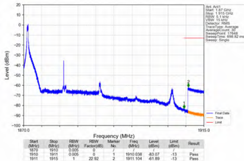
n2 30kHz SISO NTV 20MHz CP-OFDM QPSK 1880MHz Edge 1RB Left
