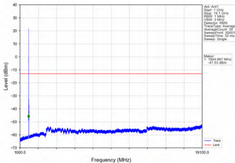
n2_30kHz_SISO_NTNV_20MHz_DFT-s-OFDM PI/2 BPSK_1880MHz_Edge_1RB_Left
