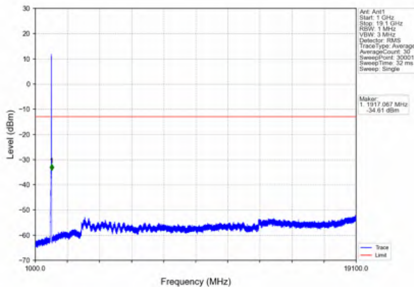
n2_30kHz_SISO_NTNV_20MHz_DFT-s-OFDM QPSK_1900MHz_Inner_1RB_Right
