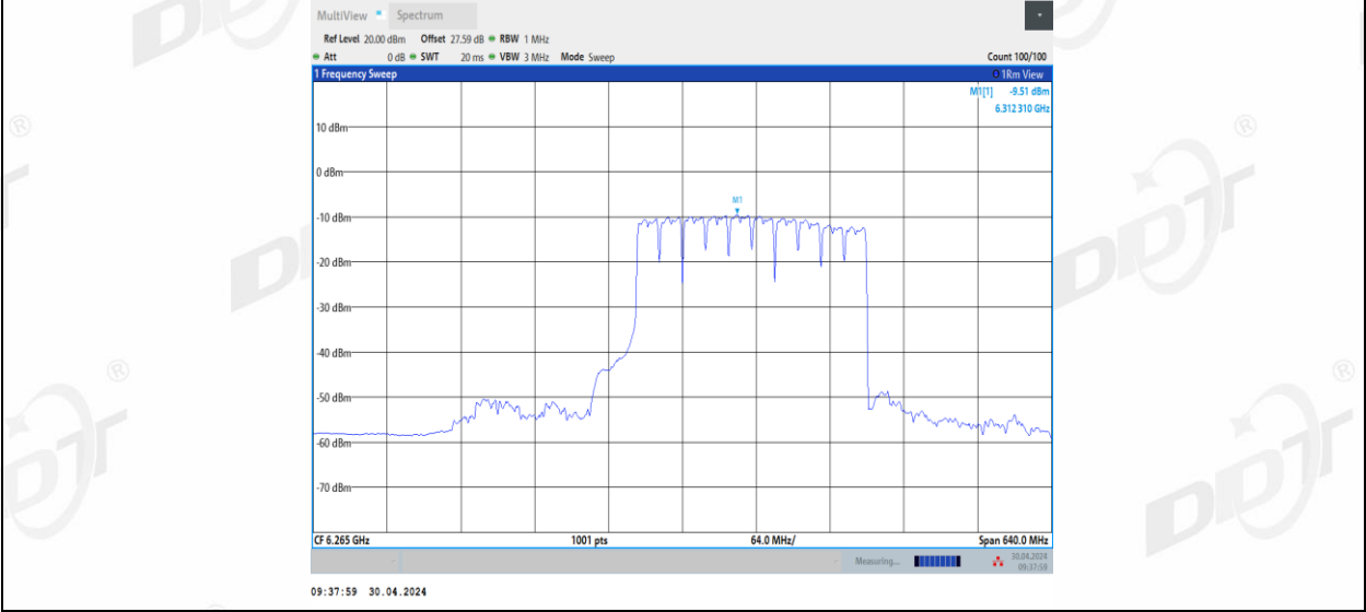
11BE320MIMO_Ant3_6265_2*996+484_8
