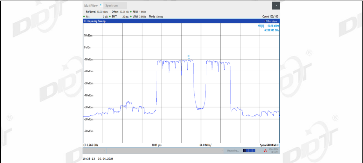
11BE320MIMO_Ant1_6265_2*996+484_11
