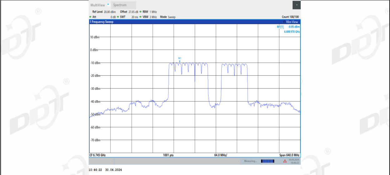
11BE320MIMO_Ant2_6745_2*996+484_11
