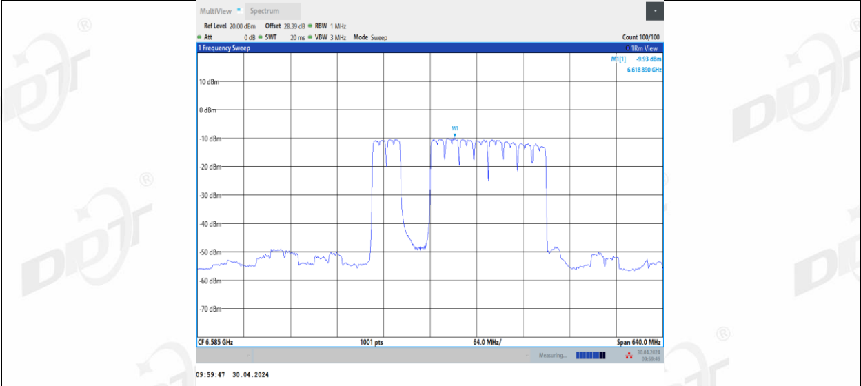
11BE320MIMO_Ant1_6585_2*996+484_9
