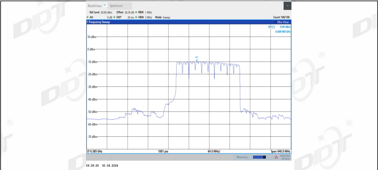
11BE320MIMO_Ant1_6585_2*996+484_8
