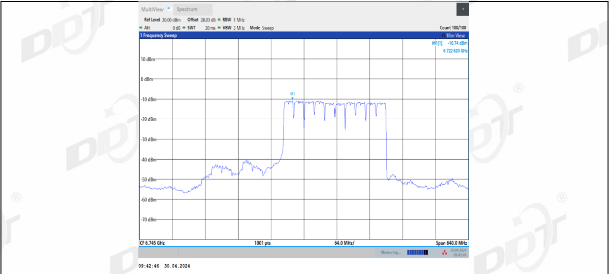
11BE320MIMO_Ant1_6745_2*996+484_8
