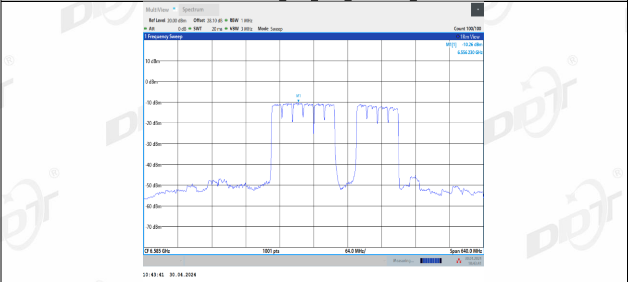
11BE320MIMO_Ant3_6585_2*996+484_11
