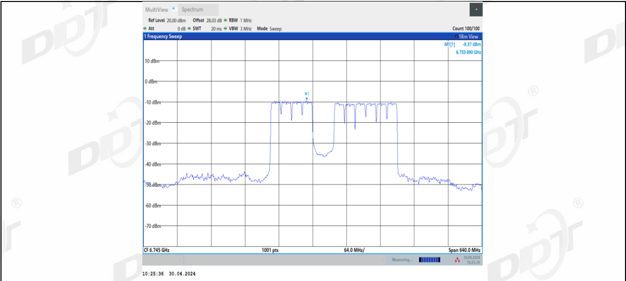
11BE320MIMO_Ant2_6745_2*996+484_10
