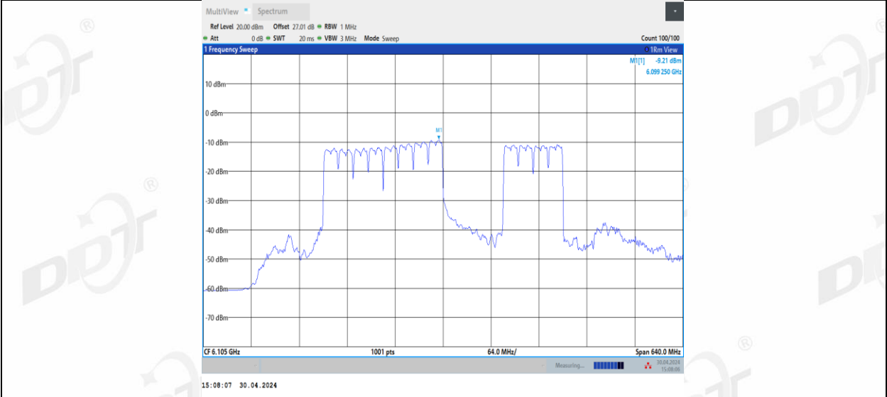
11BE320MIMO_Ant3_6105_3*996_4
