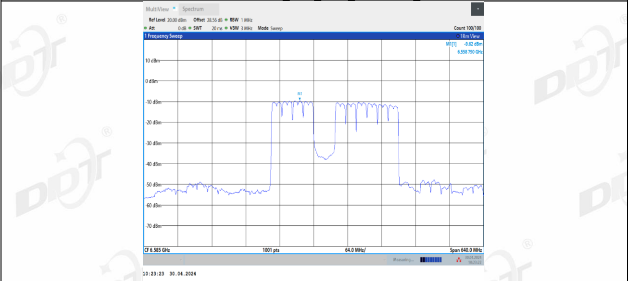
11BE320MIMO_Ant3_6585_2*996+484_10
