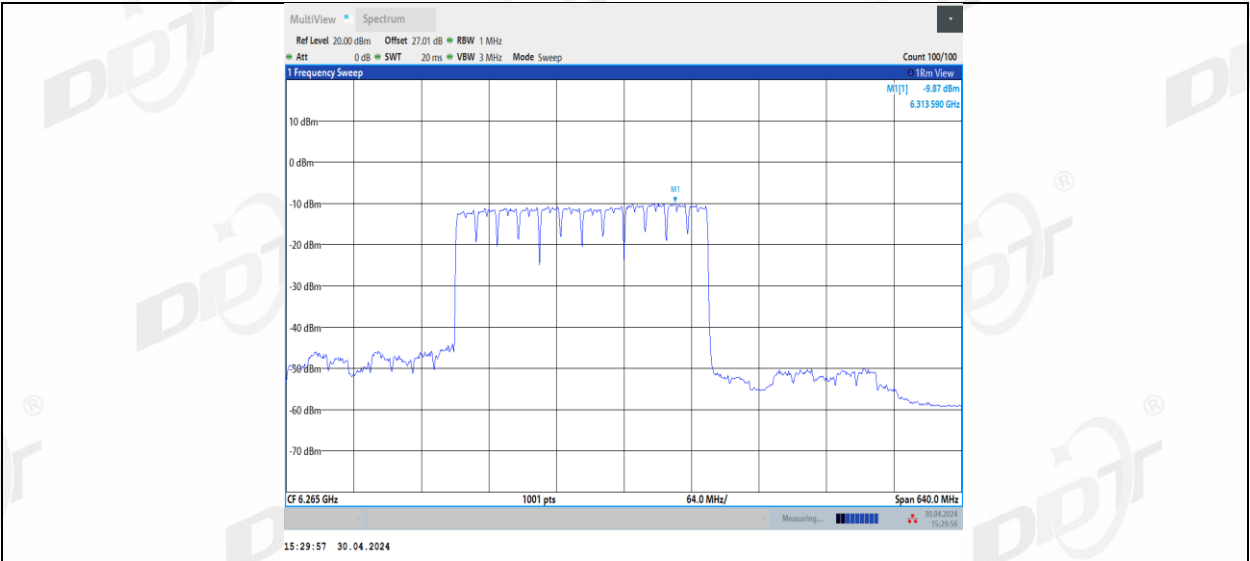
11BE320MIMO_Ant2_6265_2*996+484_7
