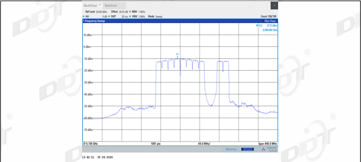
11BE320MIMO_Ant3_6105_2*996+484_12
