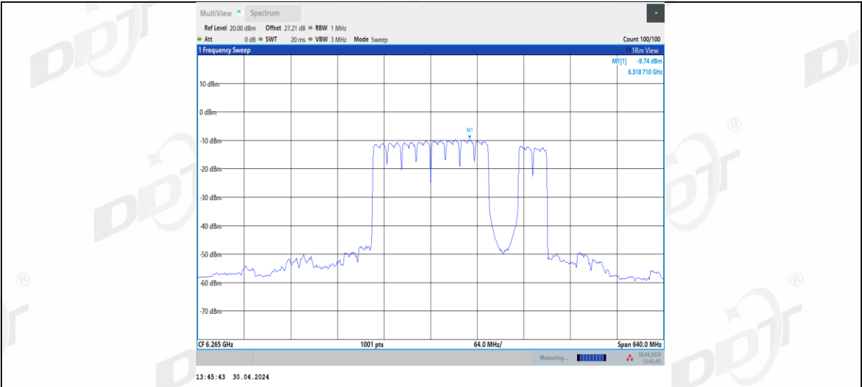
11BE320MIMO_Ant3_6265_2*996+484_12
