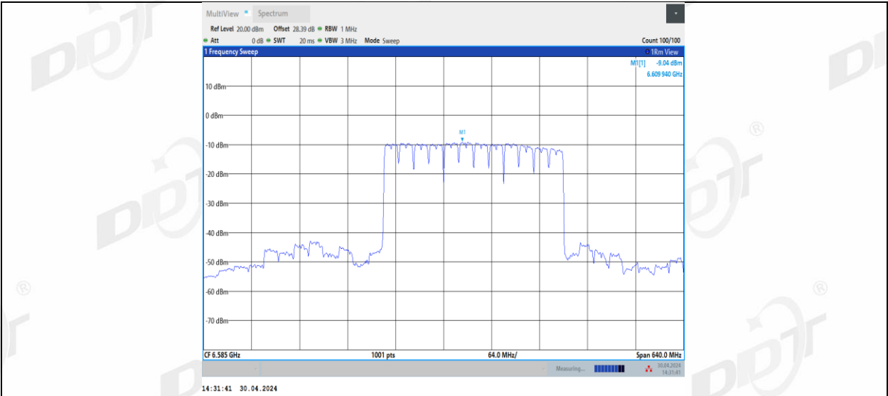
11BE320MIMO_Ant1_6585_3*996_2
