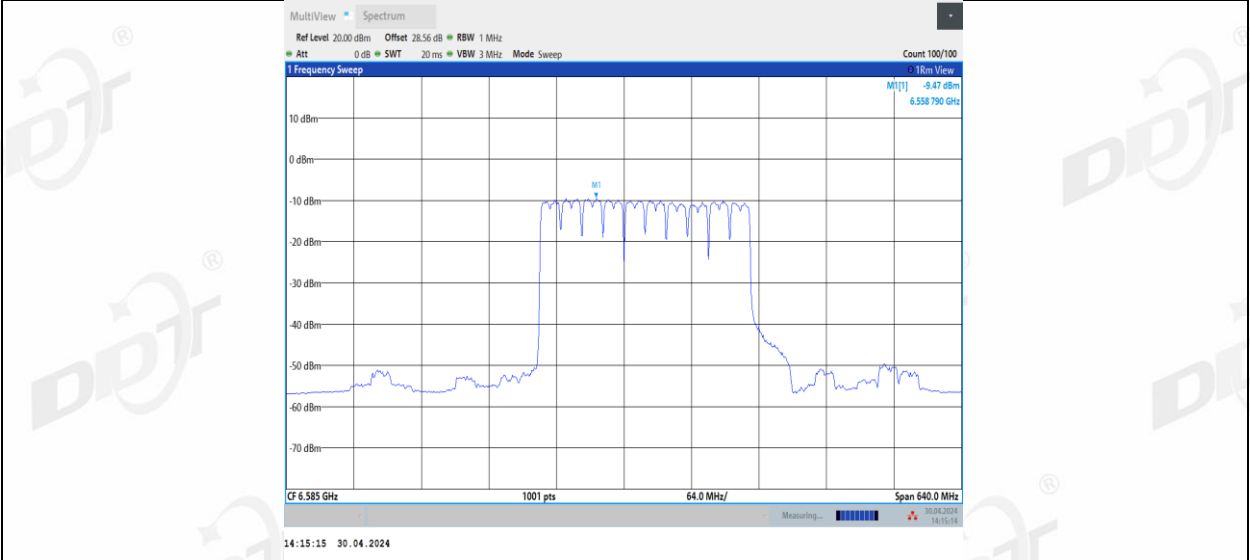
11BE320MIMO_Ant3_6585_3*996_1
