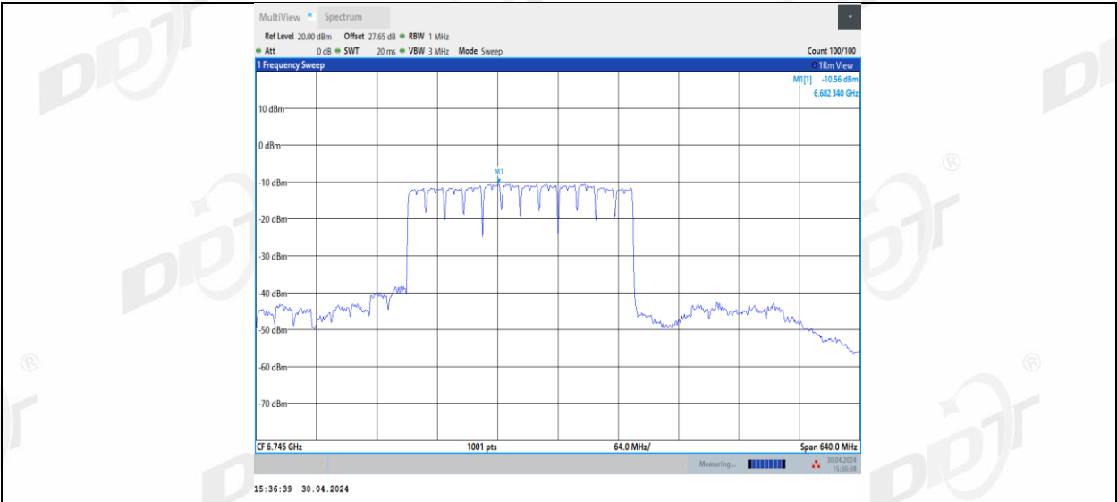
11BE320MIMO_Ant2_6745_2*996+484_7
