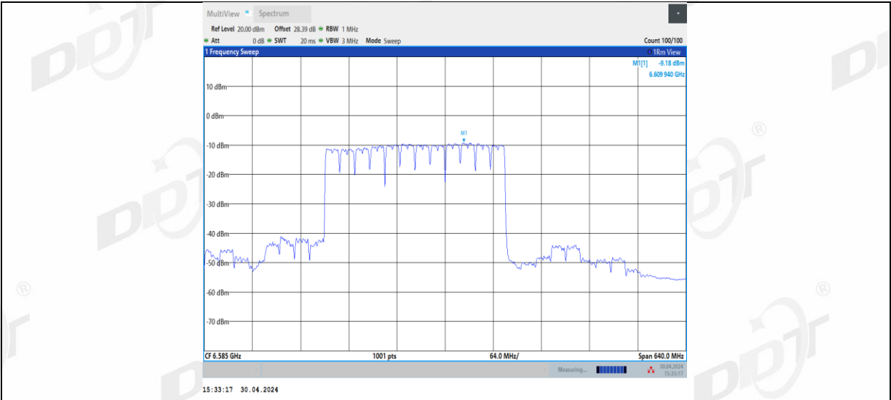
11BE320MIMO_Ant2_6585_2*996+484_7
