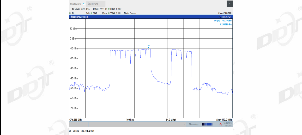
11BE320MIMO_Ant3_6265_3*996_4
