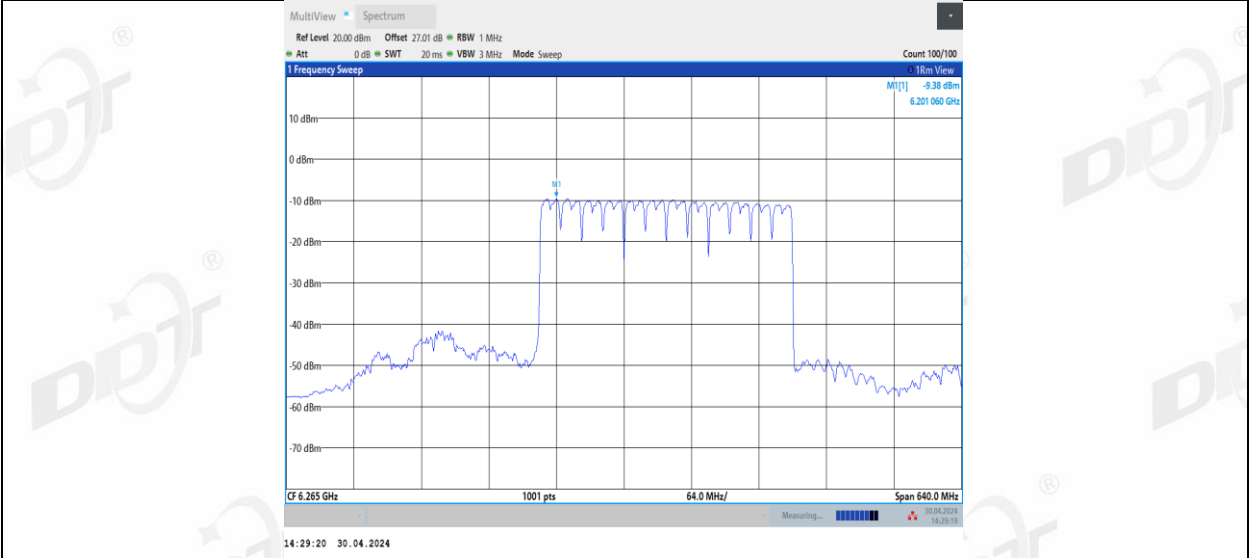
11BE320MIMO_Ant2_6265_3*996_2
