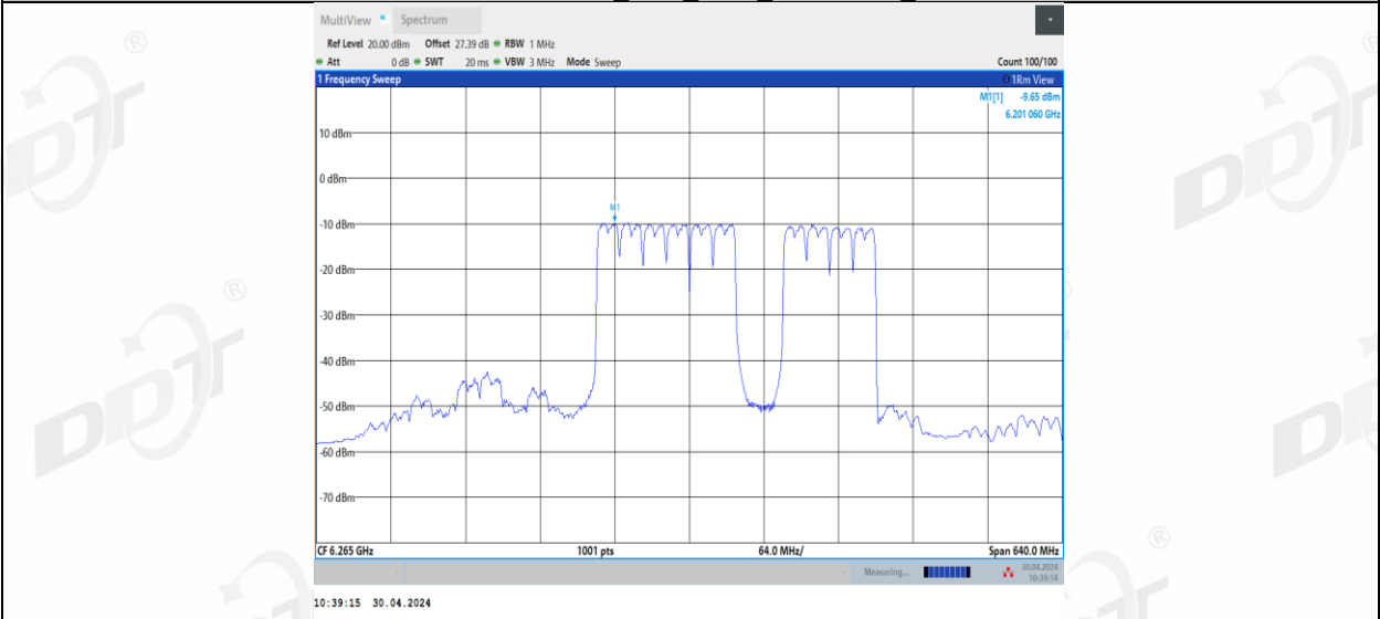
11BE320MIMO_Ant2_6265_2*996+484_11
