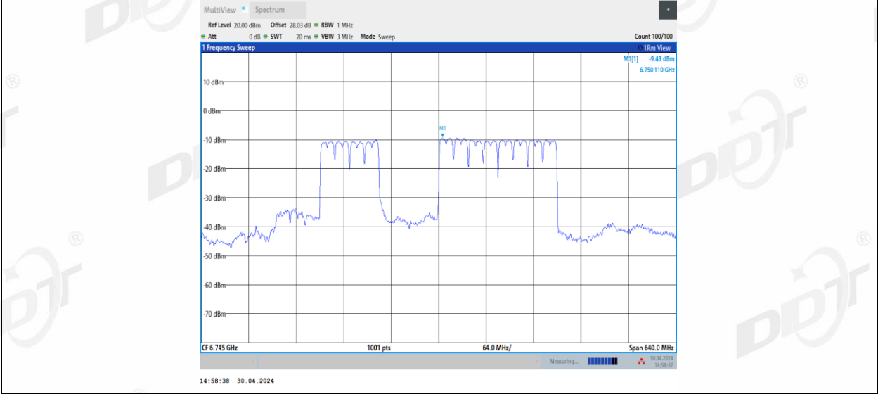
11BE320MIMO_Ant2_6745_3*996_3
