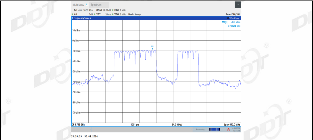
11BE320MIMO_Ant2_6745_3*996_4
