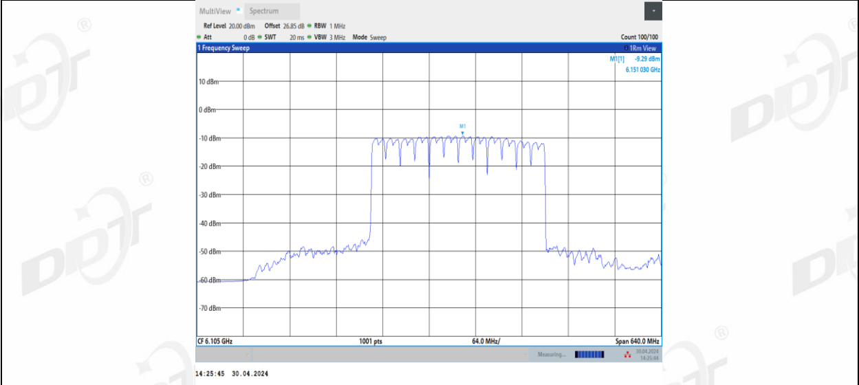
11BE320MIMO_Ant2_6105_3*996_2
