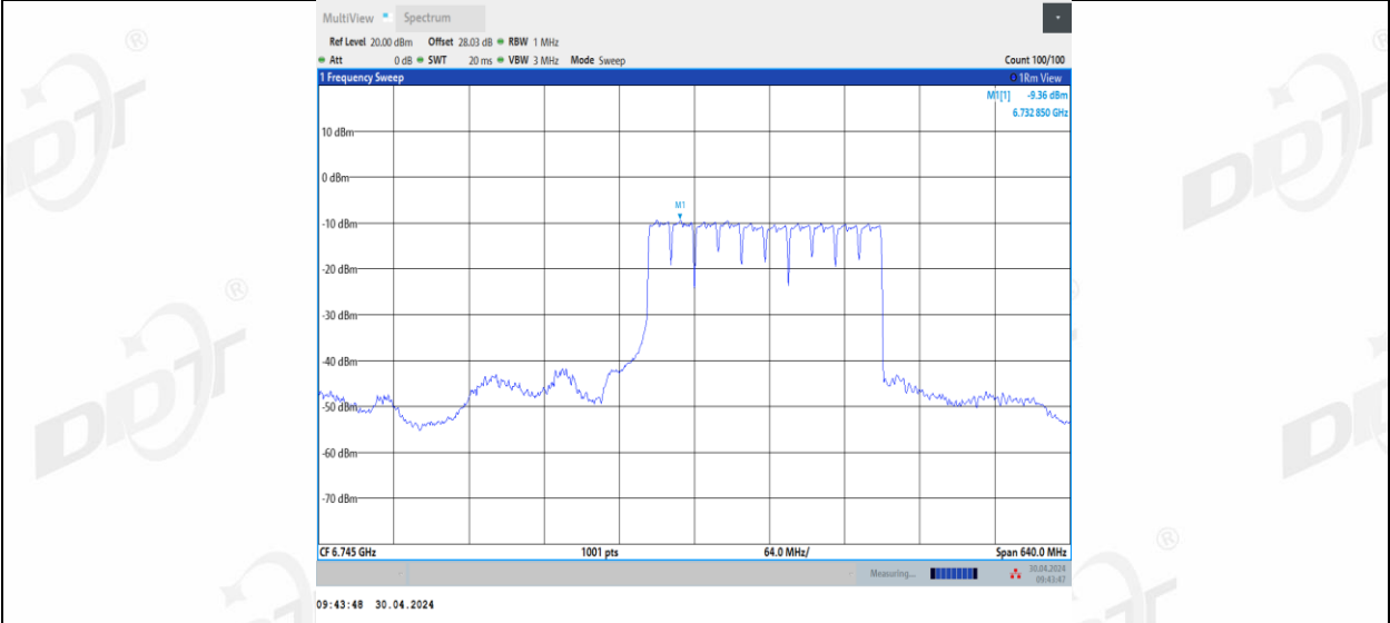
11BE320MIMO_Ant2_6745_2*996+484_8
