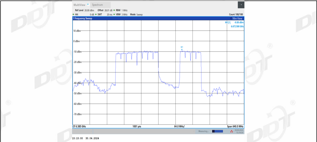
11BE320MIMO_Ant2_6585_3*996_4
