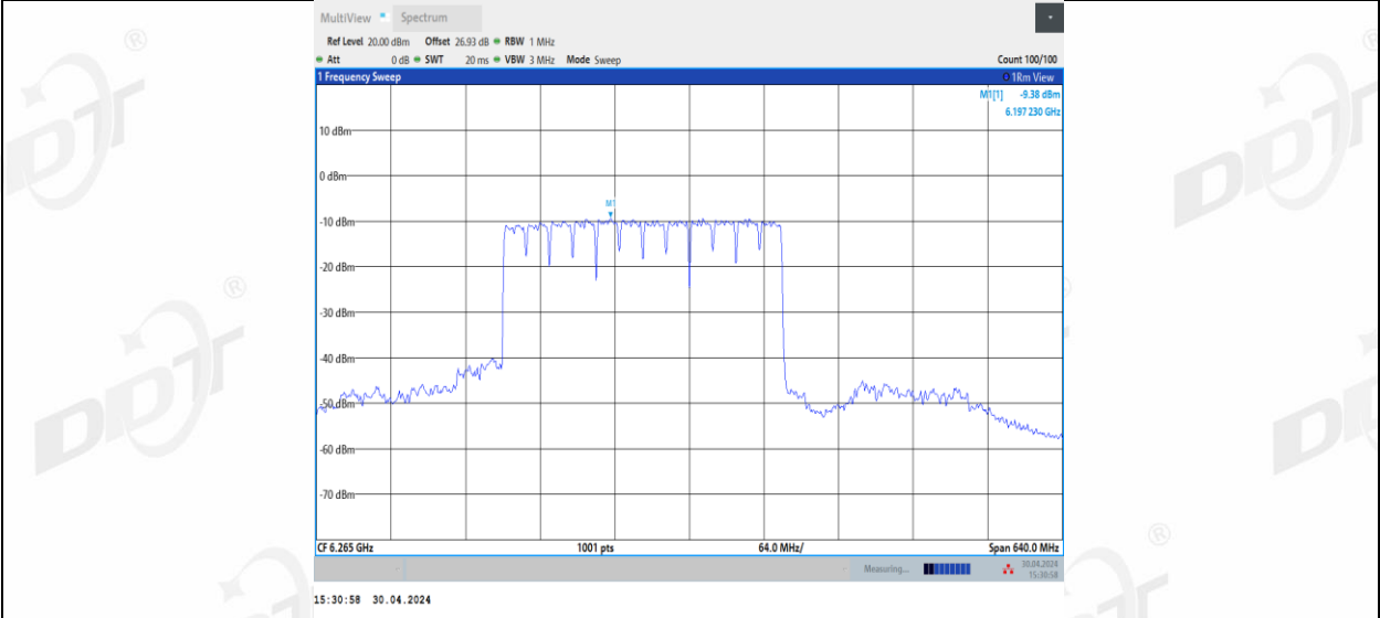
11BE320MIMO_Ant3_6265_2*996+484_7
