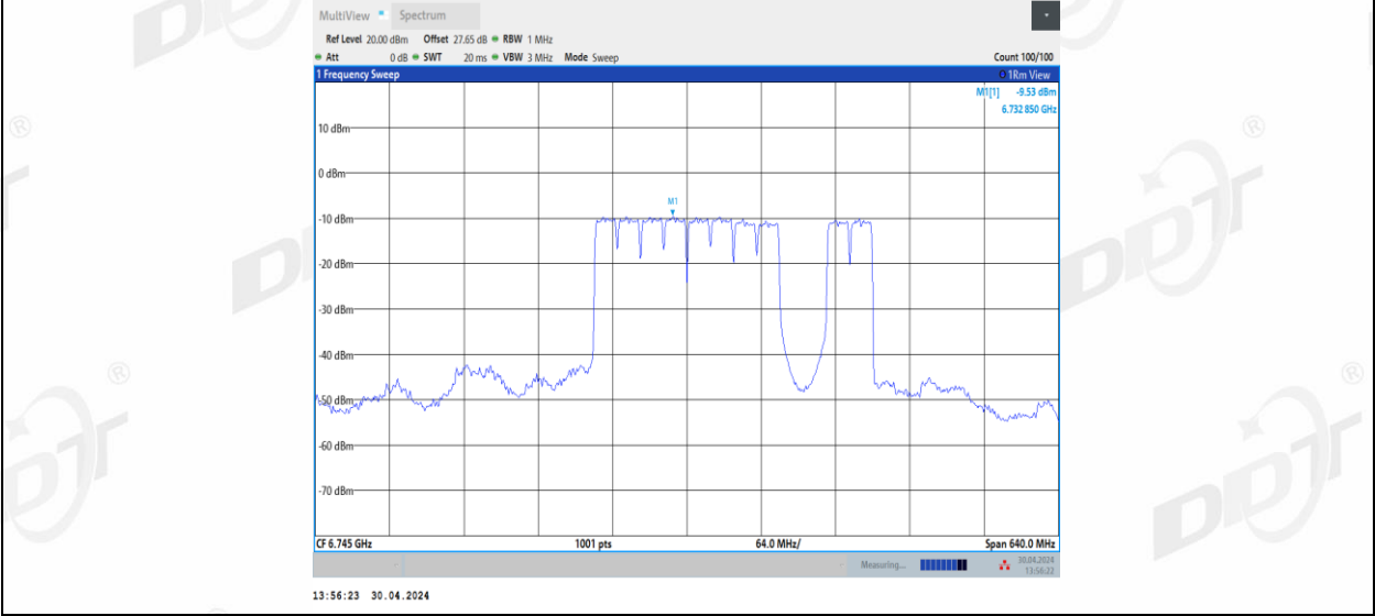
11BE320MIMO_Ant2_6745_2*996+484_12
