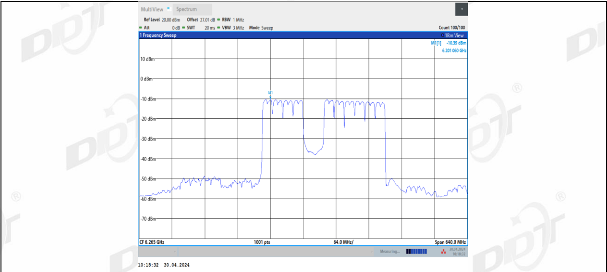
11BE320MIMO_Ant2_6265_2*996+484_10
