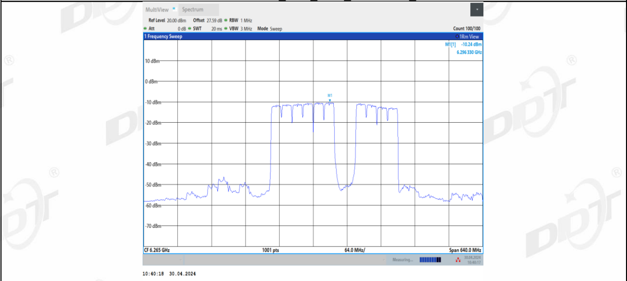
11BE320MIMO_Ant3_6265_2*996+484_11
