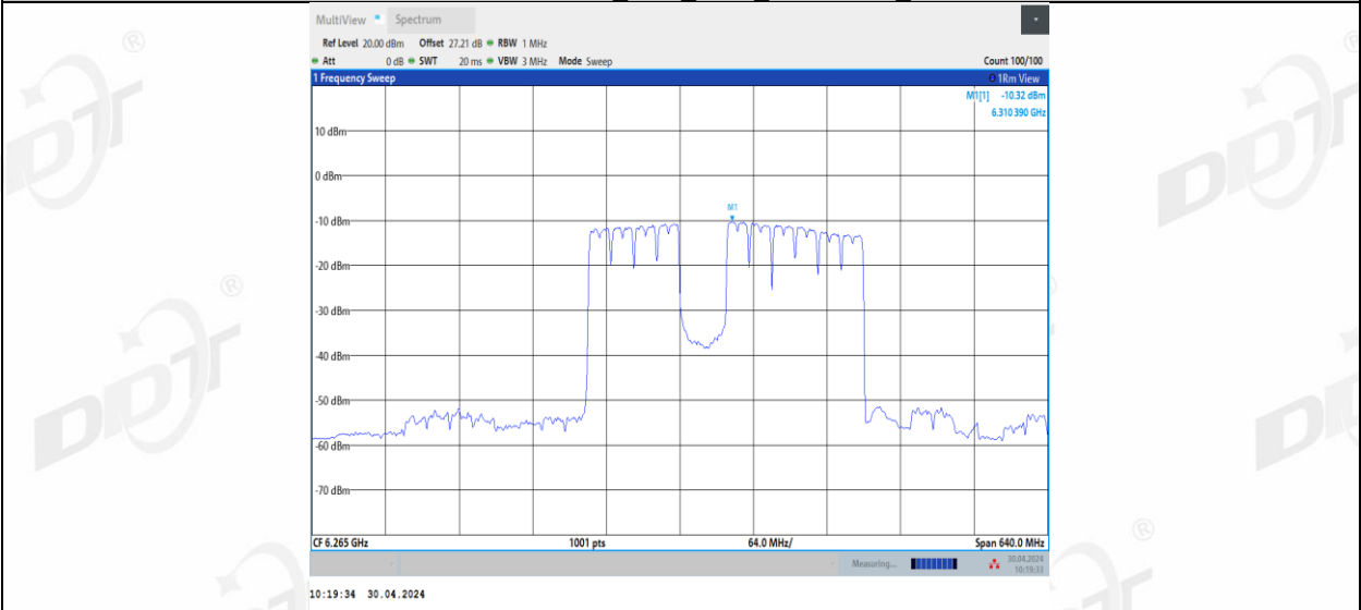
11BE320MIMO_Ant3_6265_2*996+484_10
