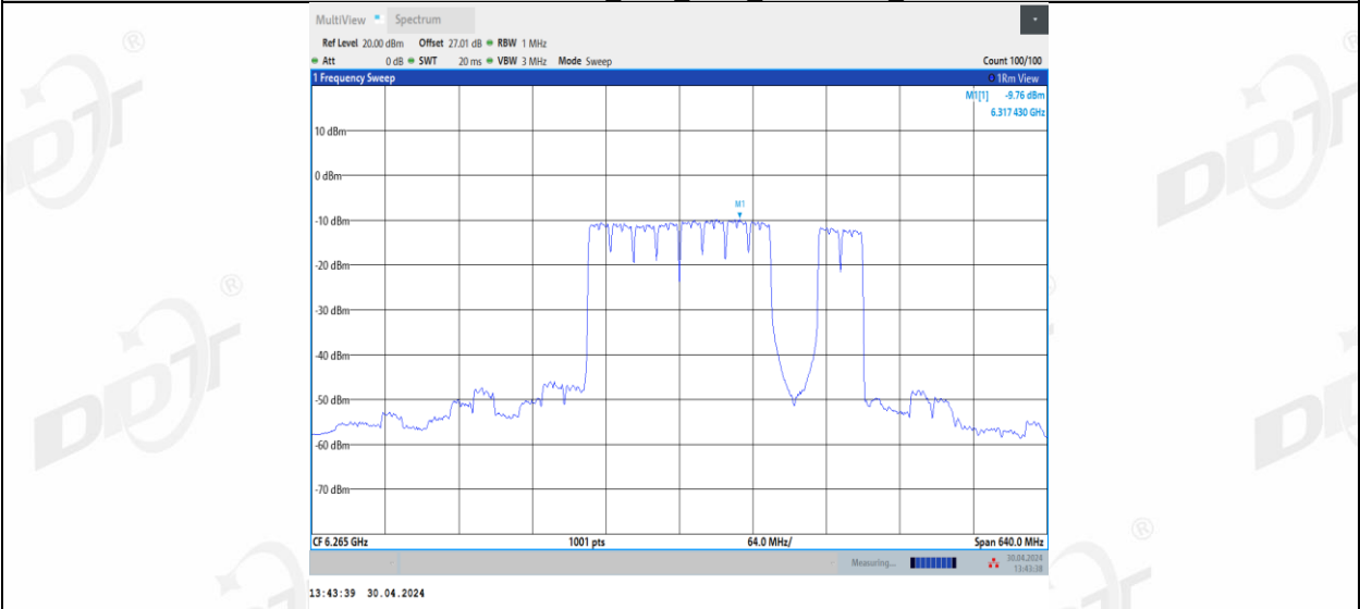
11BE320MIMO_Ant1_6265_2*996+484_12
