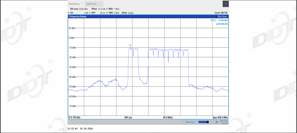
11BE320MIMO_Ant1_6745_2*996+484_9
