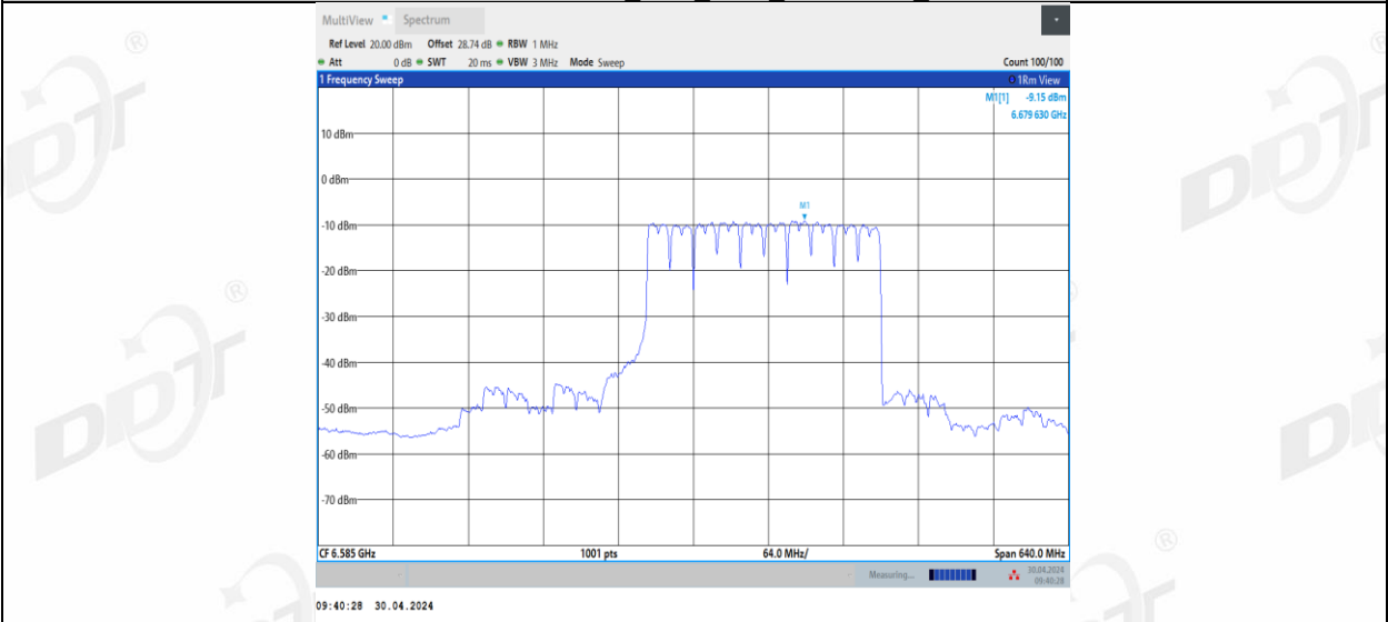
11BE320MIMO_Ant2_6585_2*996+484_8
