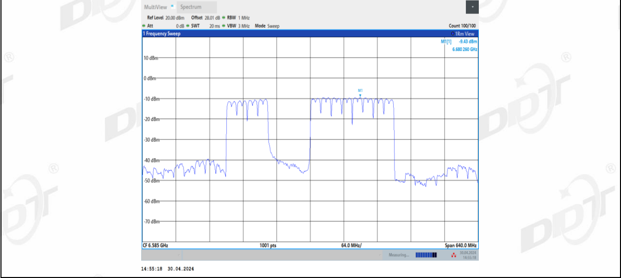
11BE320MIMO_Ant2_6585_3*996_3
