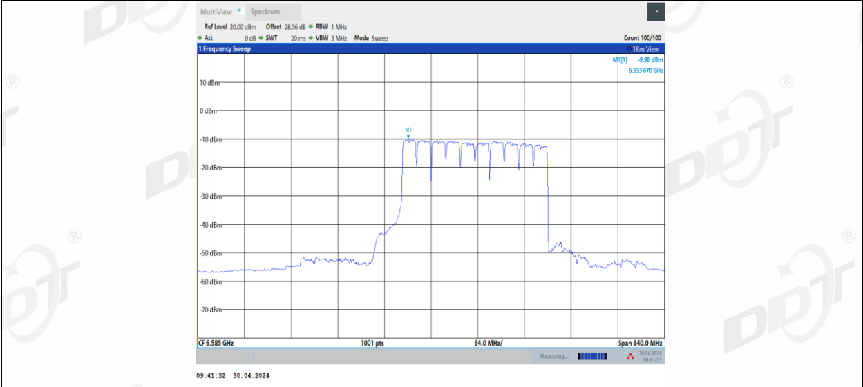
11BE320MIMO_Ant3_6585_2*996+484_8
