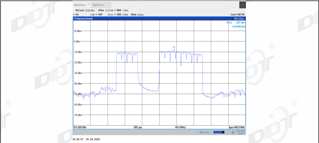
11BE320MIMO_Ant3_6265_3*996_3
