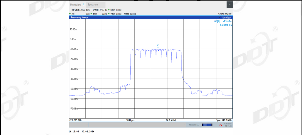
11BE320MIMO_Ant1_6585_3*996_1
