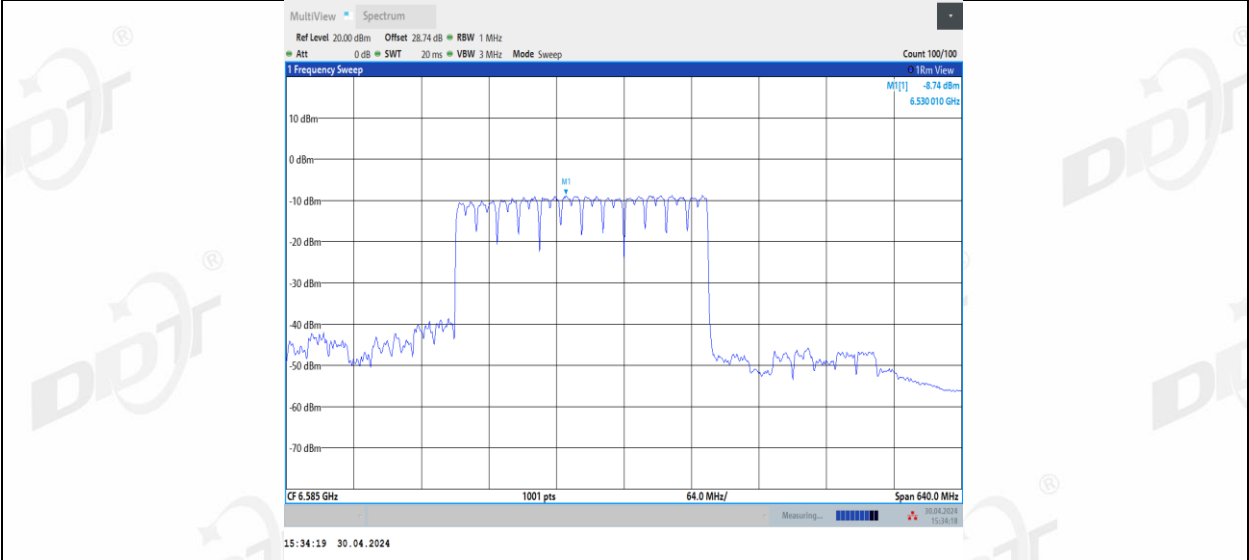
11BE320MIMO_Ant3_6585_2*996+484_7
