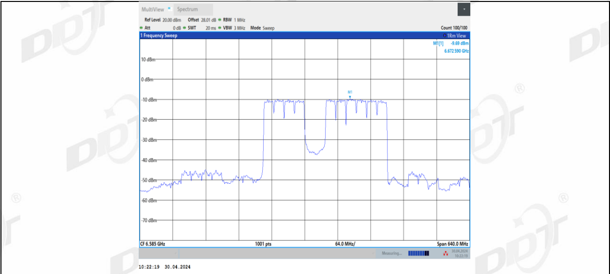
11BE320MIMO_Ant2_6585_2*996+484_10
