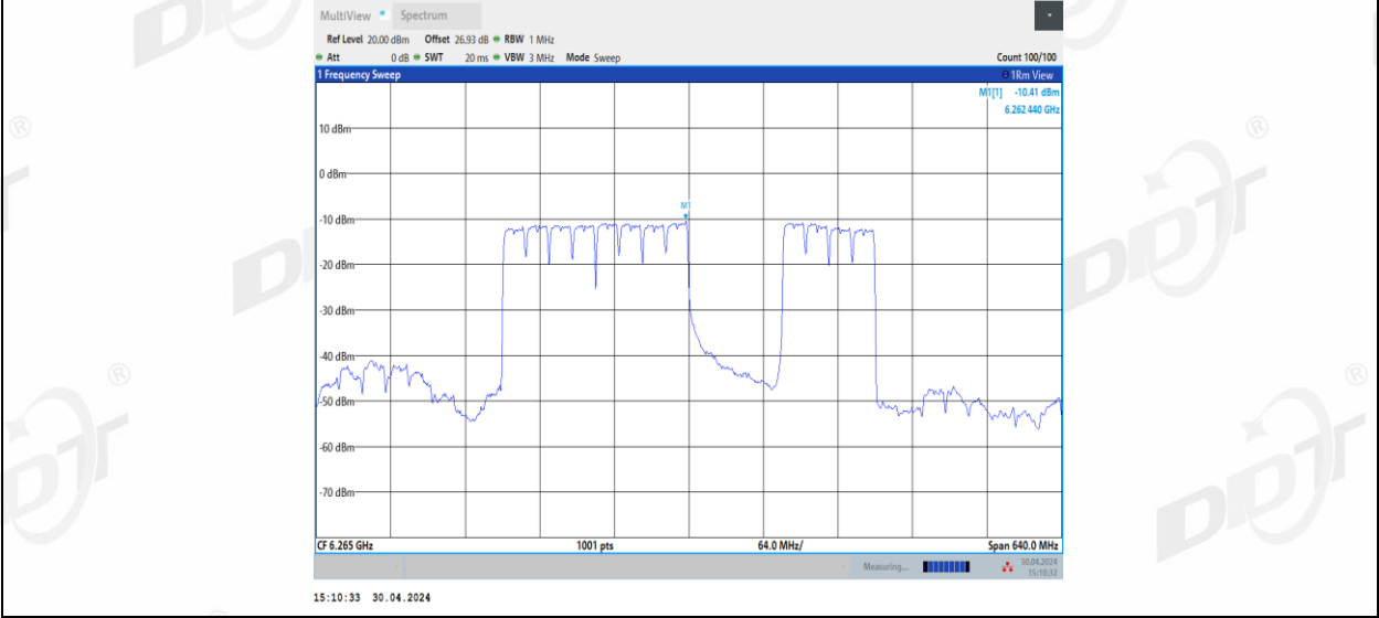
11BE320MIMO_Ant1_6265_3*996_4
