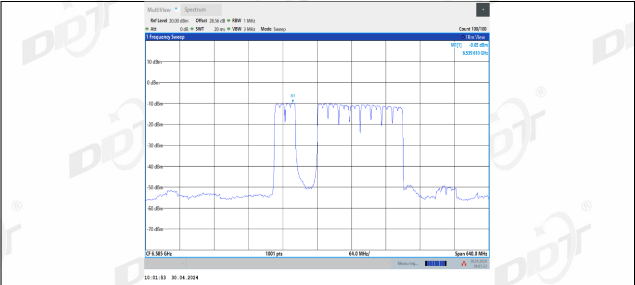
11BE320MIMO_Ant3_6585_2*996+484_9
