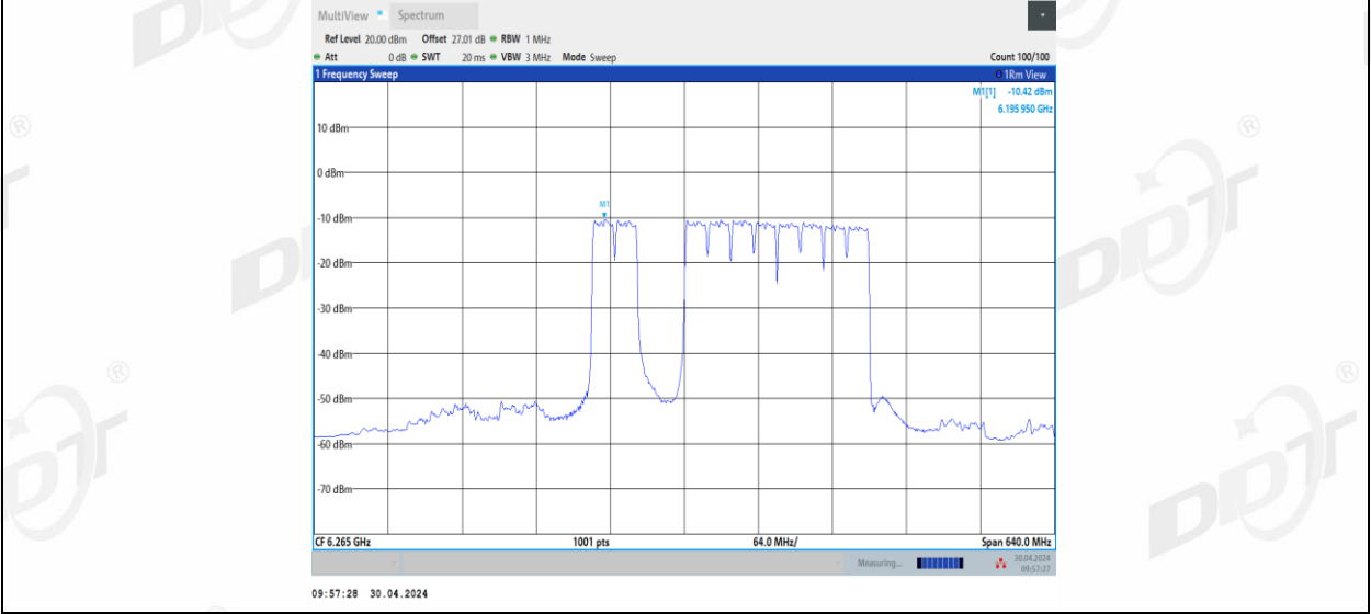
11BE320MIMO_Ant2_6265_2*996+484_9
