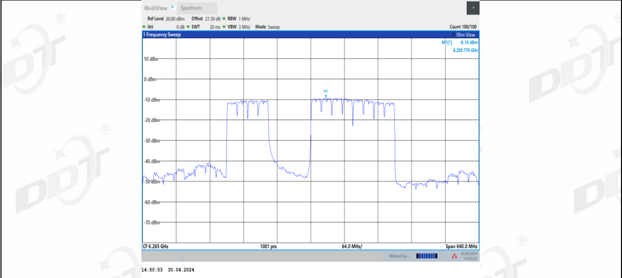
11BE320MIMO_Ant1_6265_3*996_3
