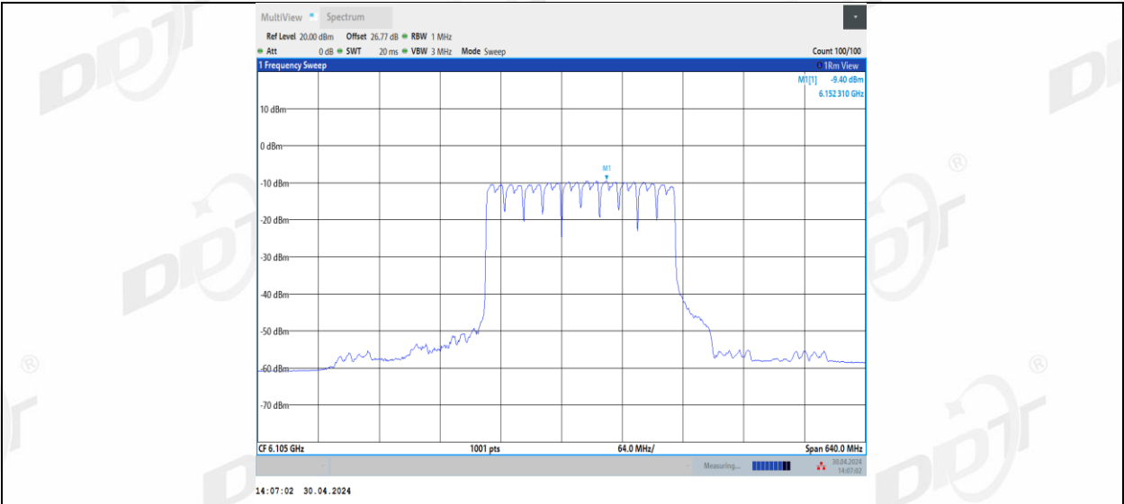
11BE320MIMO_Ant2_6105_3*996_1
