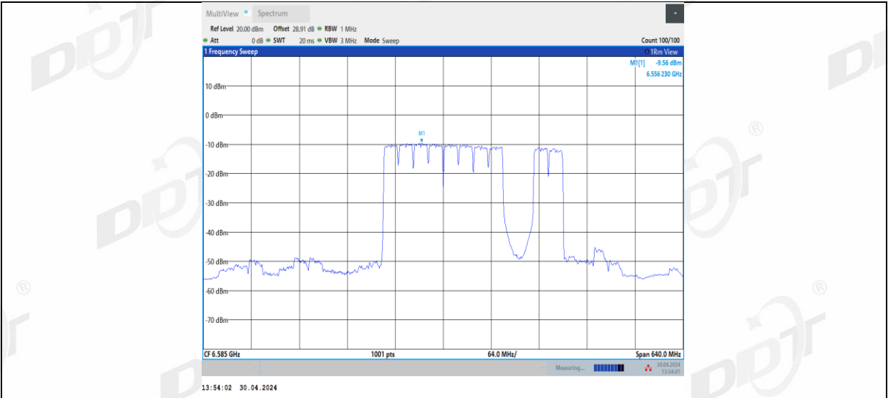
11BE320MIMO_Ant3_6585_2*996+484_12
