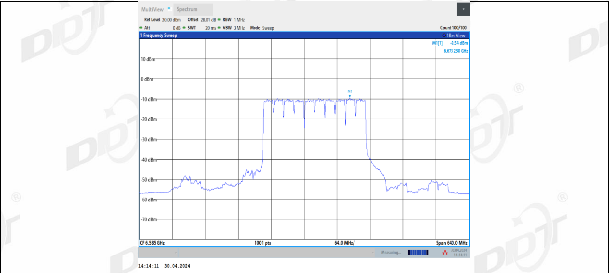
11BE320MIMO_Ant2_6585_3*996_1
