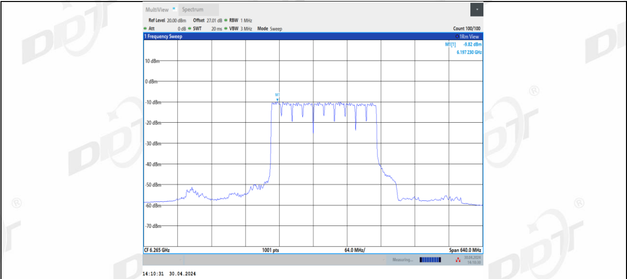
11BE320MIMO_Ant2_6265_3*996_1
