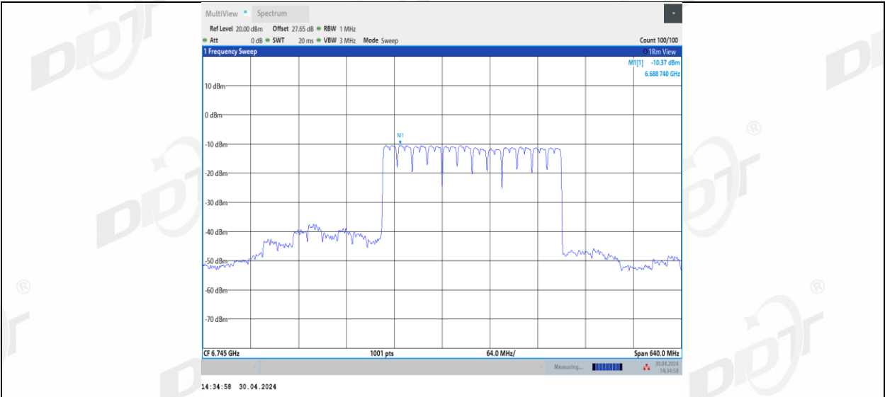
11BE320MIMO_Ant1_6745_3*996_2
