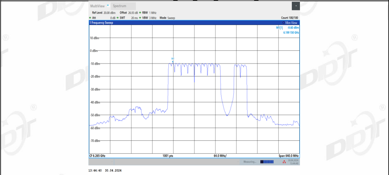
11BE320MIMO_Ant2_6265_2*996+484_12
