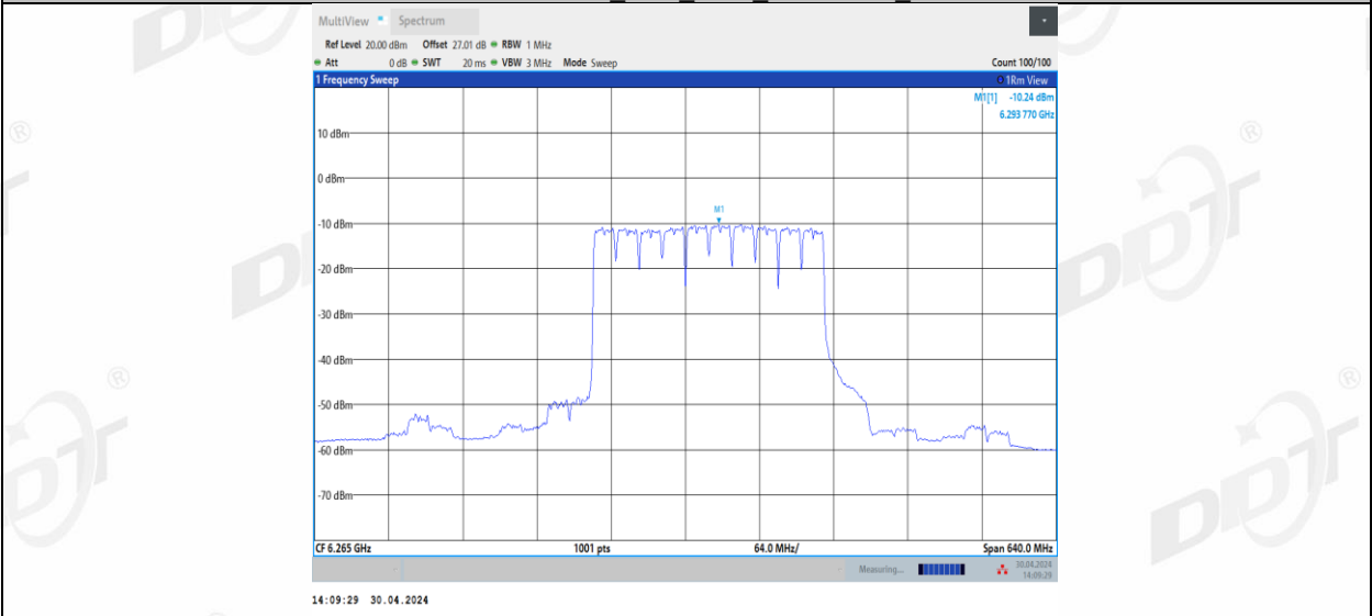
11BE320MIMO_Ant1_6265_3*996_1
