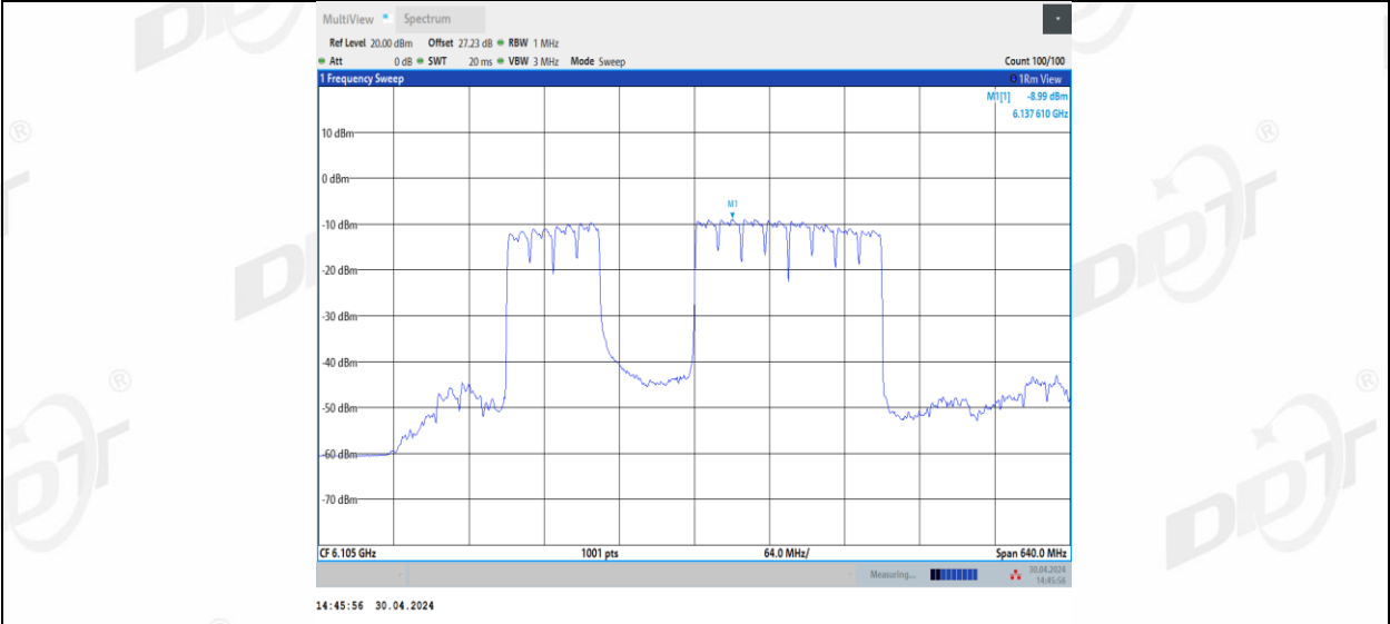
11BE320MIMO_Ant2_6105_3*996_3
