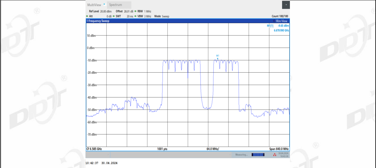
11BE320MIMO_Ant2_6585_2*996+484_11
