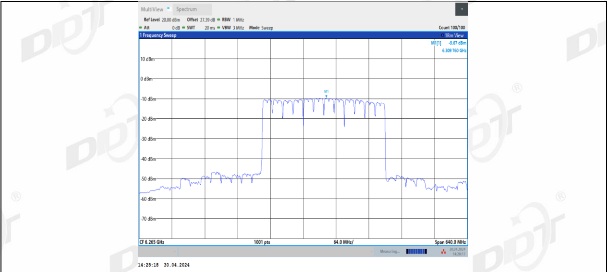
11BE320MIMO_Ant1_6265_3*996_2
