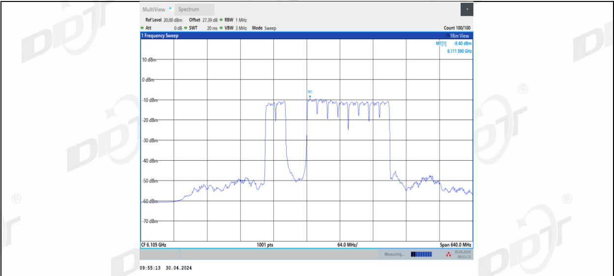
11BE320MIMO_Ant3_6105_2*996+484_9
