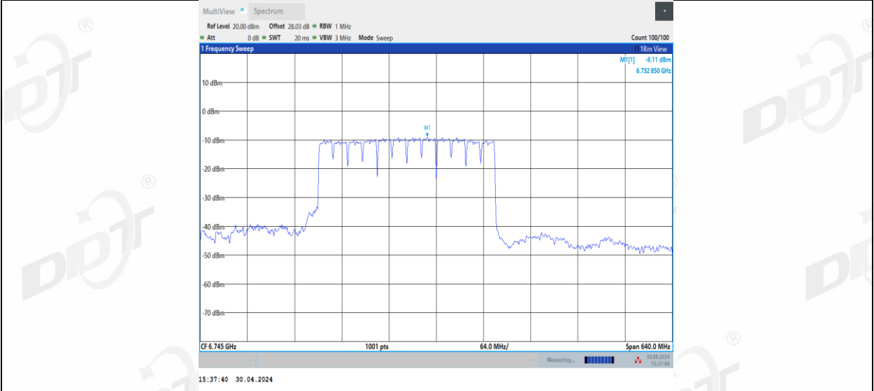
11BE320MIMO_Ant3_6745_2*996+484_7
