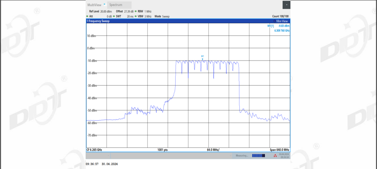
11BE320MIMO_Ant2_6265_2*996+484_8
