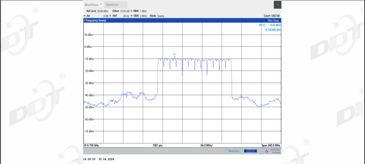
11BE320MIMO_Ant2_6745_3*996_2
