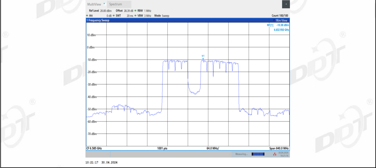
11BE320MIMO_Ant1_6585_2*996+484_10
