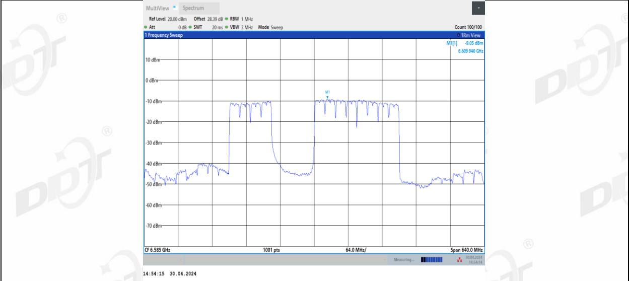
11BE320MIMO_Ant1_6585_3*996_3
