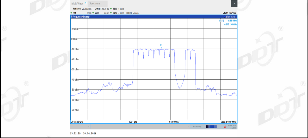
11BE320MIMO_Ant2_6585_2*996+484_12
