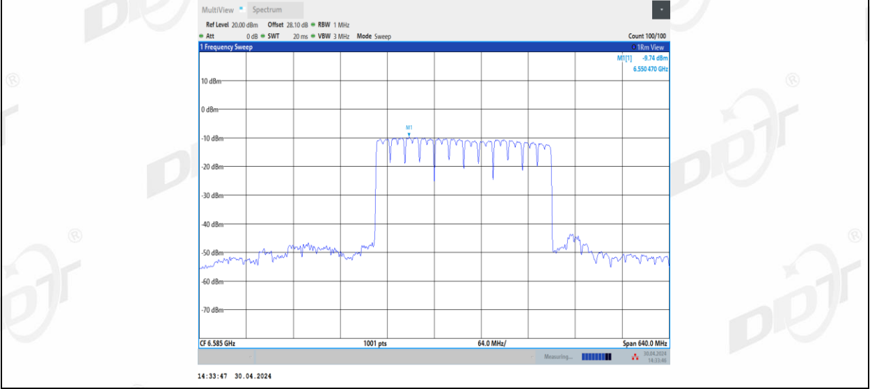
11BE320MIMO_Ant3_6585_3*996_2
