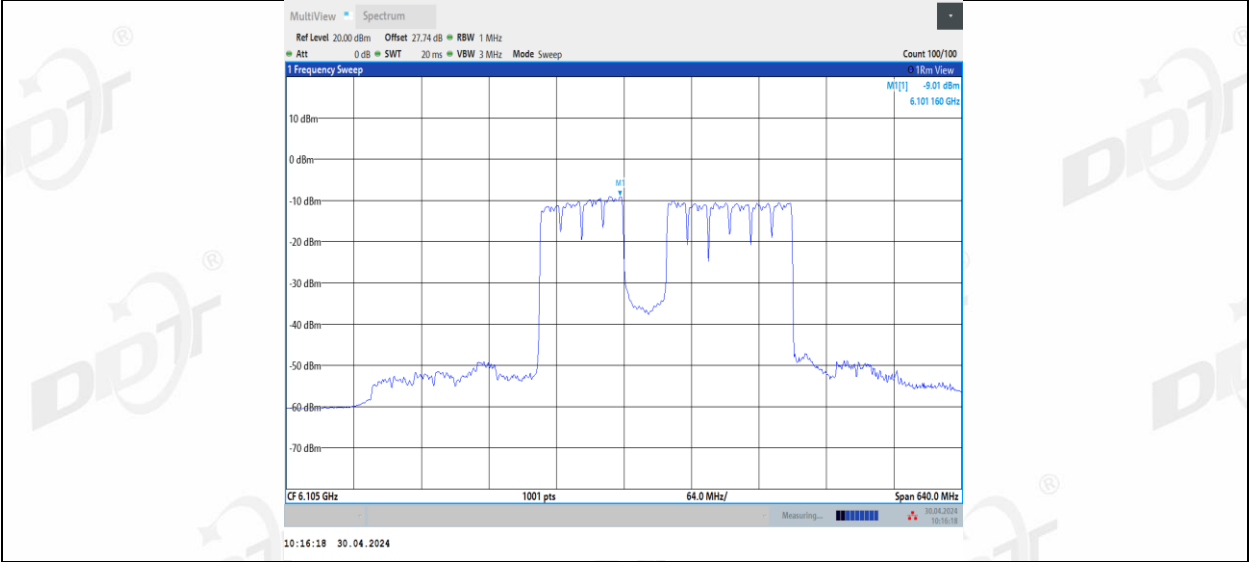
11BE320MIMO_Ant3_6105_2*996+484_10
