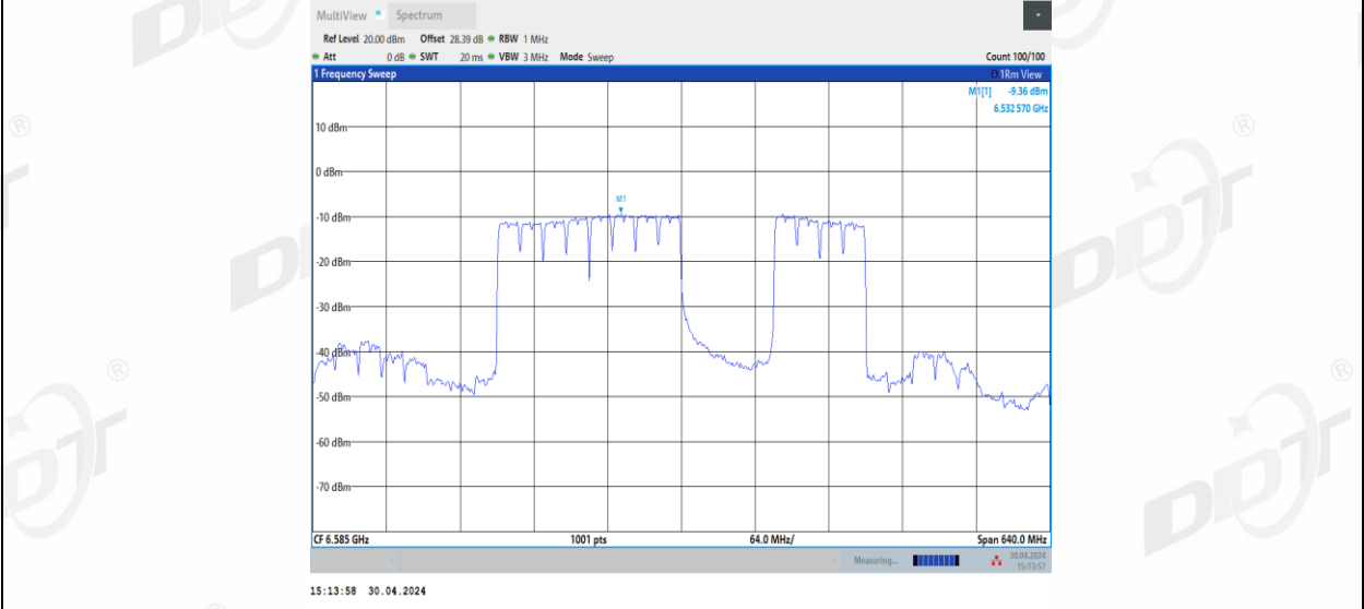
11BE320MIMO_Ant1_6585_3*996_4
