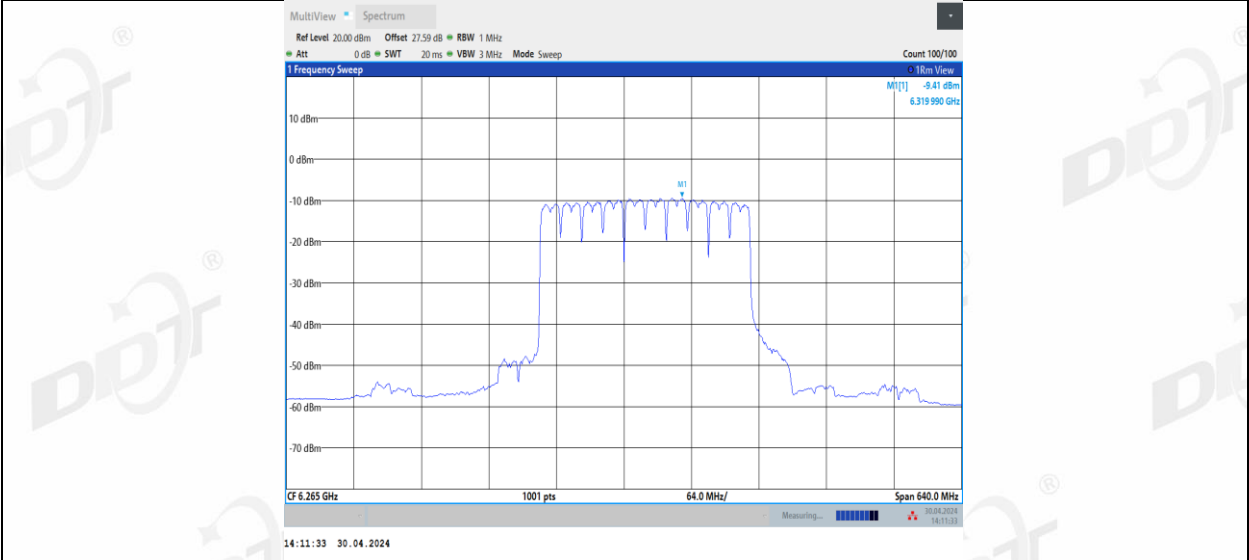
11BE320MIMO_Ant3_6265_3*996_1
