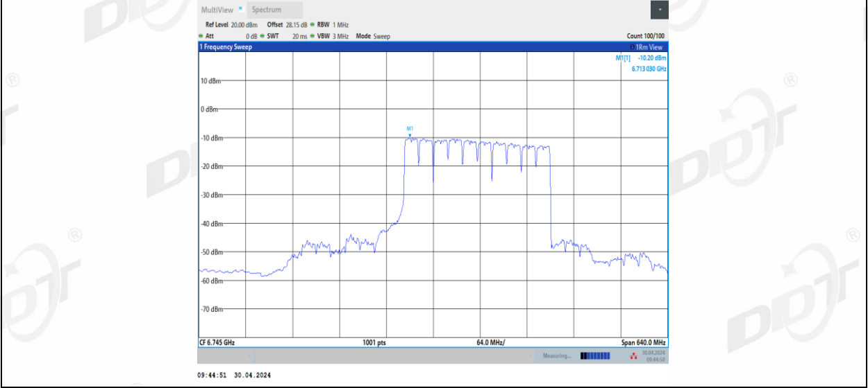
11BE320MIMO_Ant3_6745_2*996+484_8
