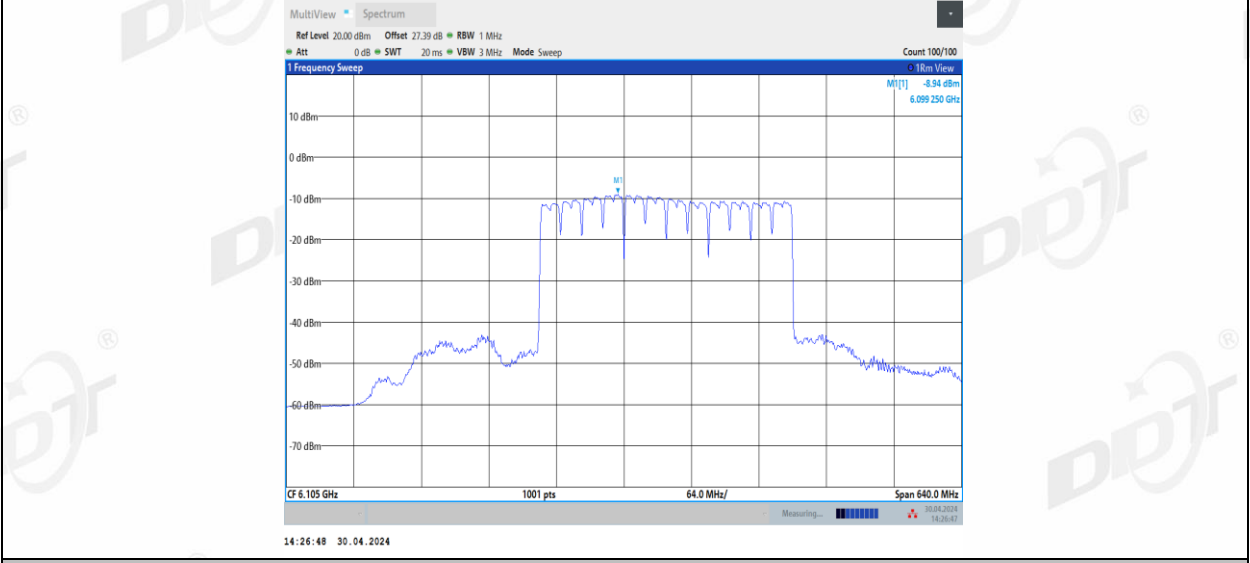
11BE320MIMO_Ant3_6105_3*996_2
