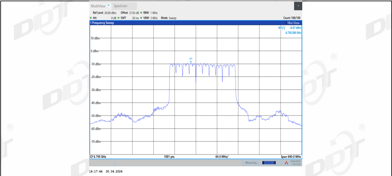
11BE320MIMO_Ant2_6745_3*996_1
