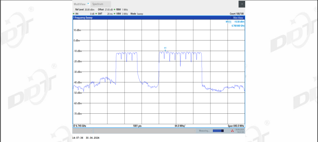
11BE320MIMO_Ant1_6745_3*996_3
