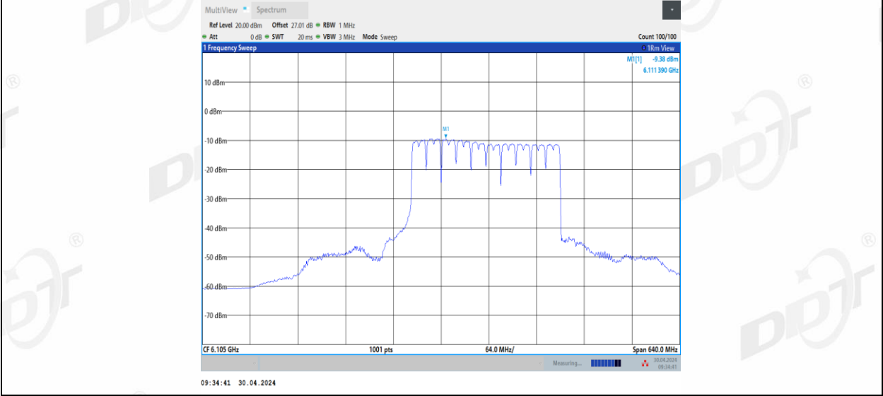
11BE320MIMO_Ant3_6105_2*996+484_8
