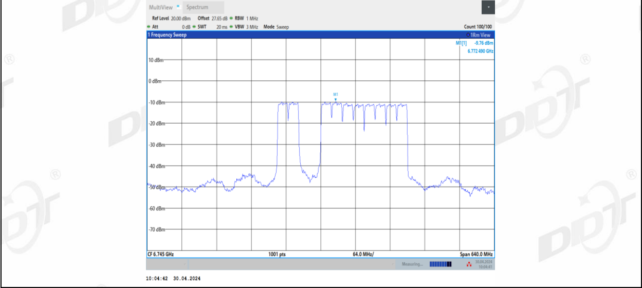
11BE320MIMO_Ant2_6745_2*996+484_9
