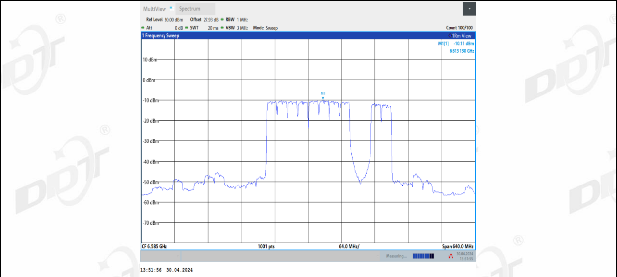
11BE320MIMO_Ant1_6585_2*996+484_12
