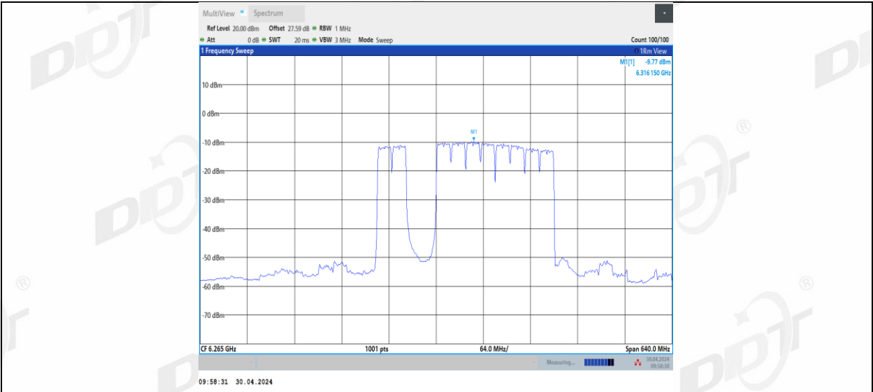
11BE320MIMO_Ant3_6265_2*996+484_9
