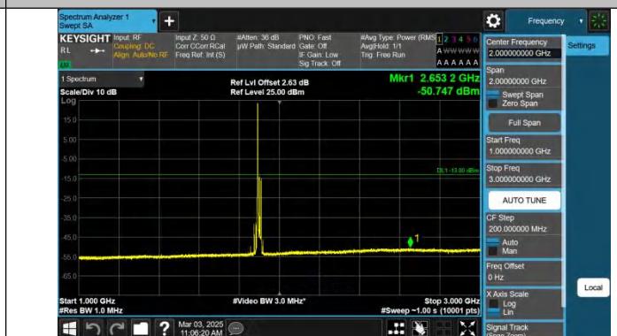
Band2-20MHz-QPSK-19100-1RB#0-1000~3000-PASS
