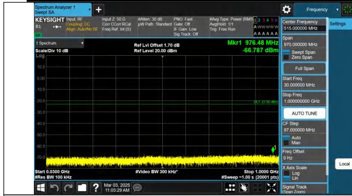
Band2-20MHz-QPSK-18700-1RB#0-30~1000-PASS
