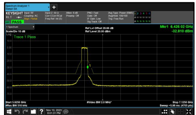
Figure 210 - A(Core 0) 802.11ax HE40 SU SP 6405 MHz (CH91)
