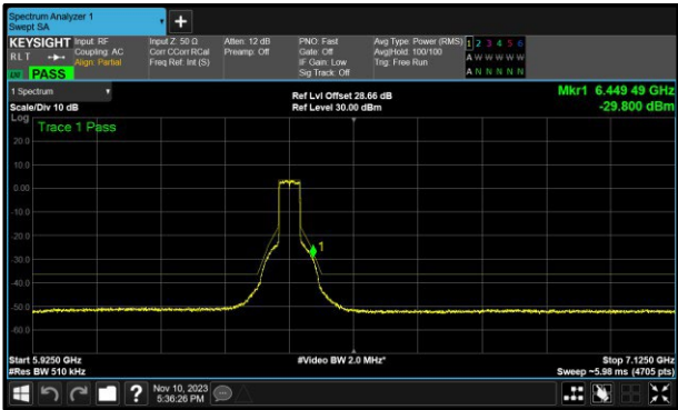
Figure 197- A(Core 0) 802.11ax HE40 SU SP 6405 MHz (CH91)
