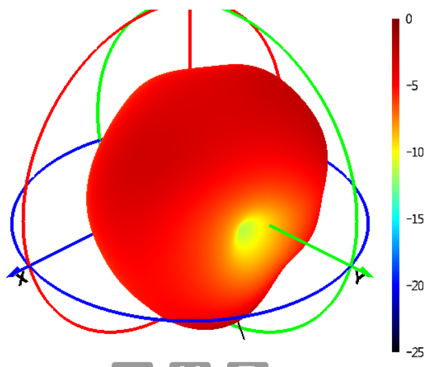
GSM1900
