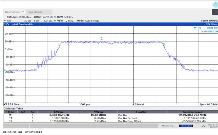
11BE20MIMO_Ant4_5320
