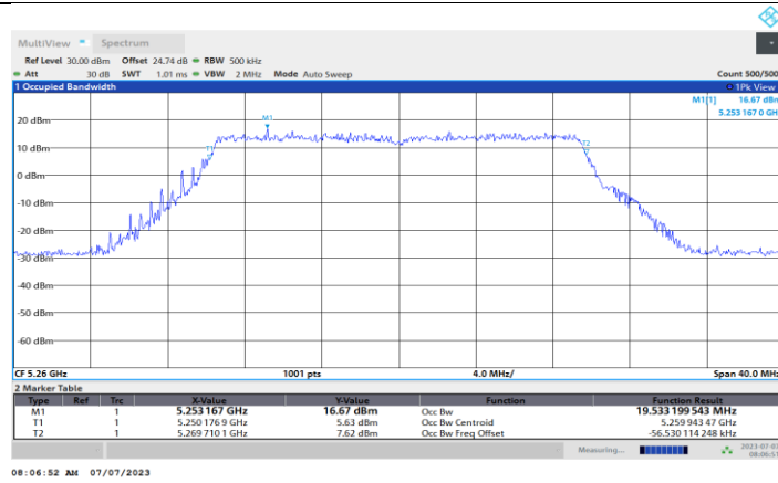
11BE20MIMO_Ant3_5260
