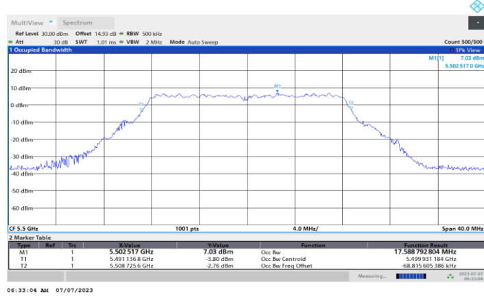
11A-CDD_Ant3_5500
