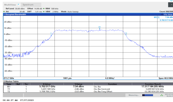
11A-CDD_Ant3_5700
