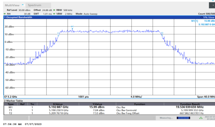
11BE20MIMO_Ant3_5200
