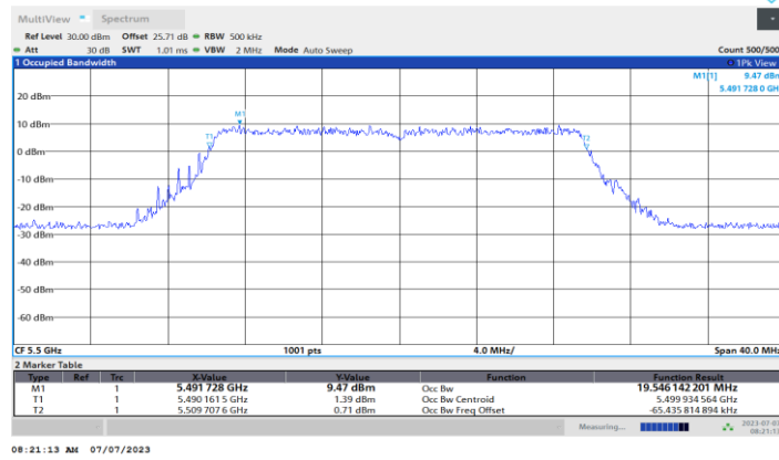
11BE20MIMO_Ant1_5500
