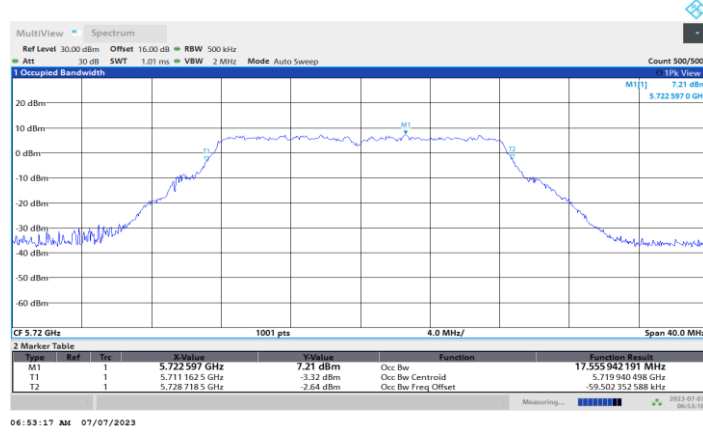
11A-CDD_Ant2_5720
