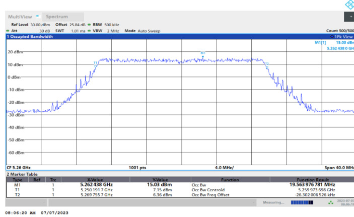
11BE20MIMO_Ant2_5260
