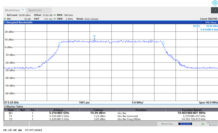
11BE20MIMO_Ant2_5320
