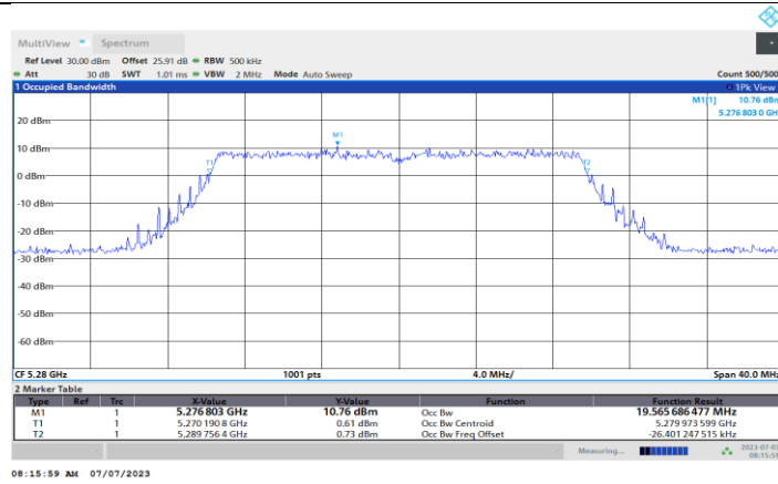
11BE20MIMO_Ant2_5280
