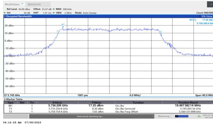
11BE20MIMO_Ant4_5745
