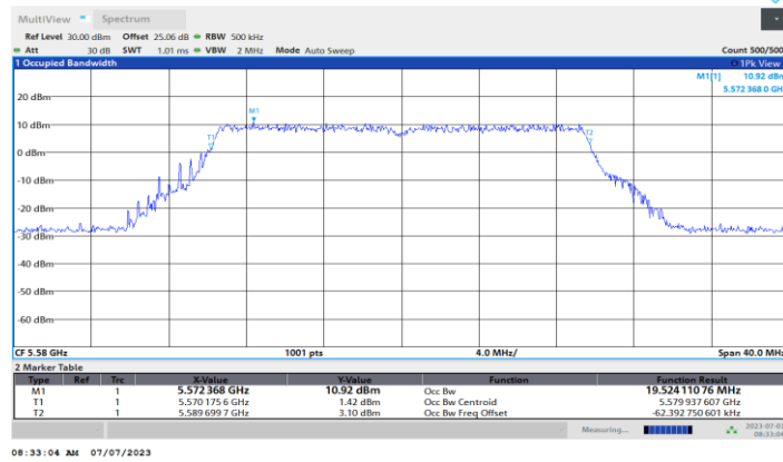
11BE20MIMO_Ant4_5580
