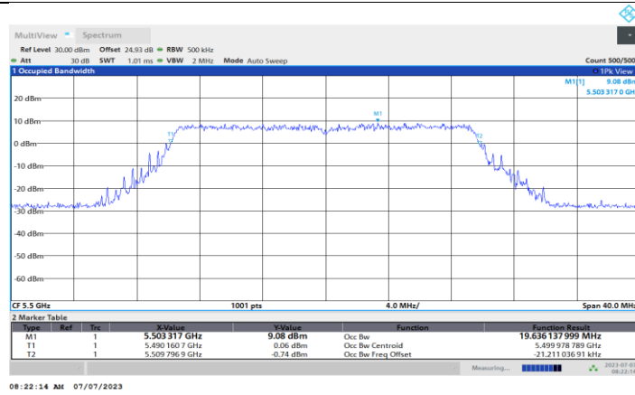
11BE20MIMO_Ant3_5500
