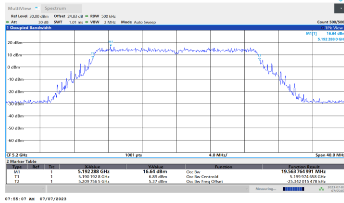
11BE20MIMO_Ant4_5200
