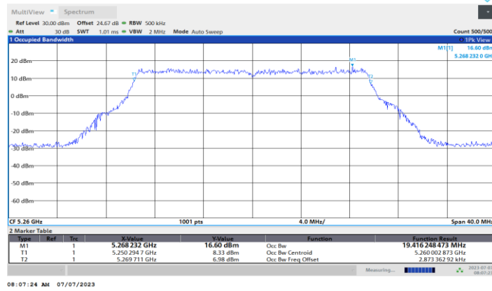
11BE20MIMO_Ant4_5260
