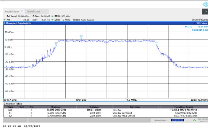
11BE20MIMO_Ant4_5700
