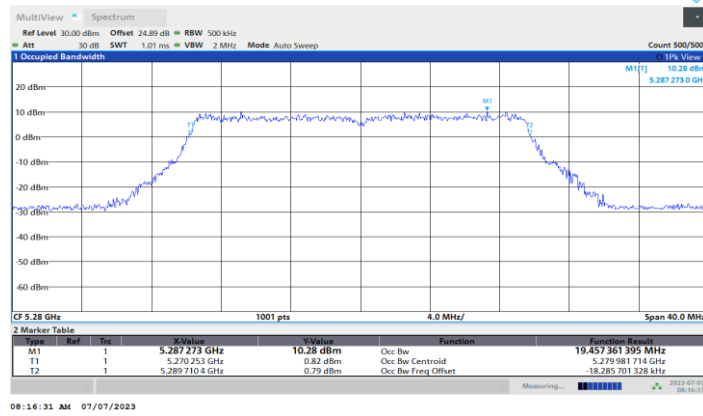
11BE20MIMO_Ant3_5280
