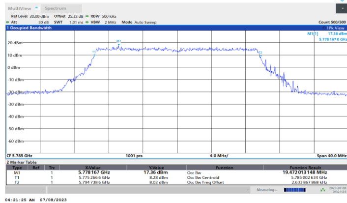
11BE20MIMO_Ant3_5785
