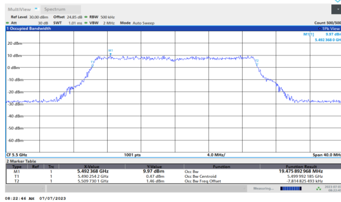
11BE20MIMO_Ant4_5500
