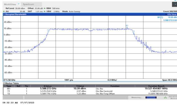
11BE20MIMO_Ant3_5580
