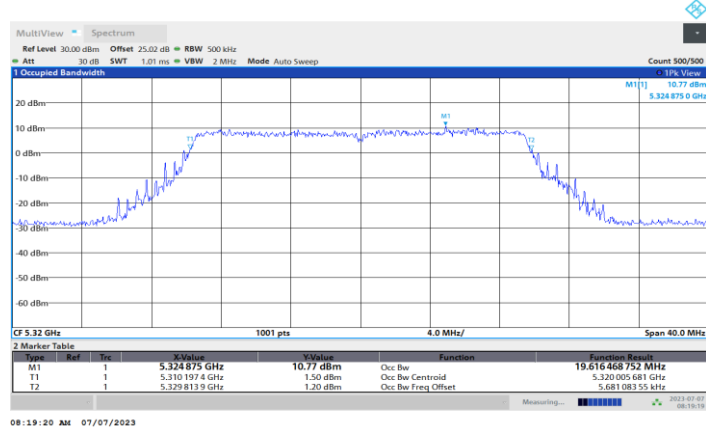
11BE20MIMO_Ant3_5320
