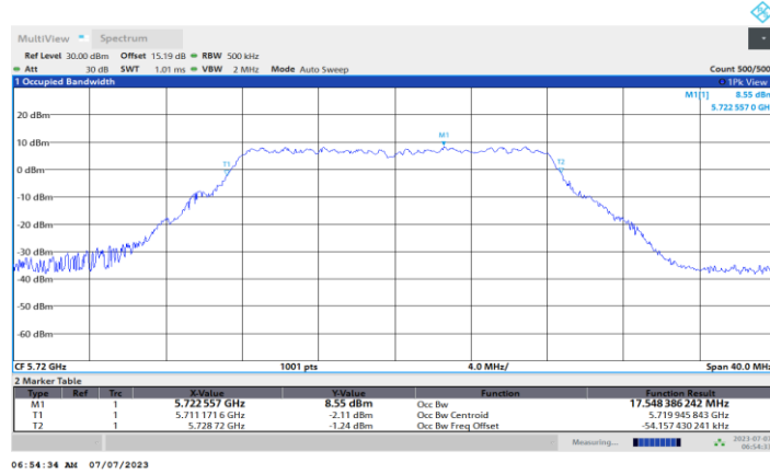
11A-CDD_Ant3_5720
