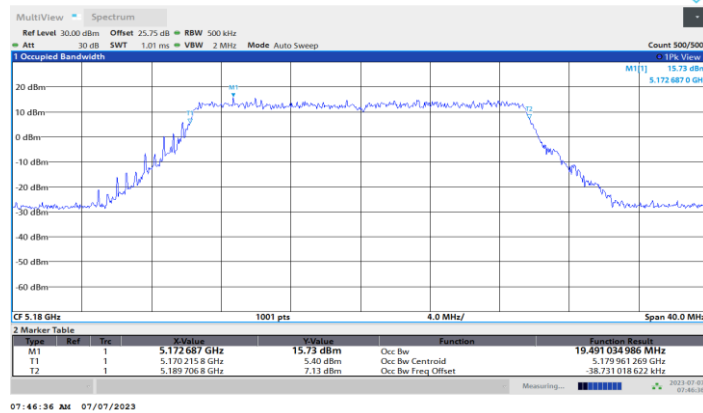
11BE20MIMO_Ant2_5180
