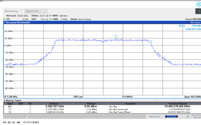
11BE20MIMO_Ant2_5580
