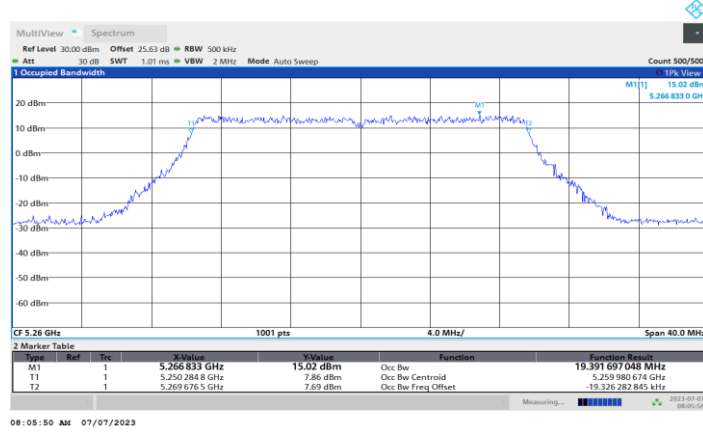
11BE20MIMO_Ant1_5260
