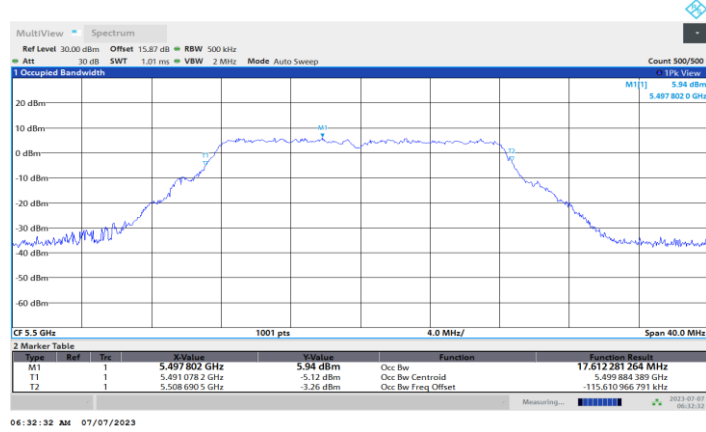
11A-CDD_Ant2_5500
