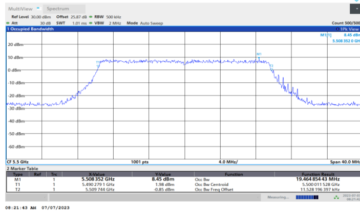
11BE20MIMO_Ant2_5500
