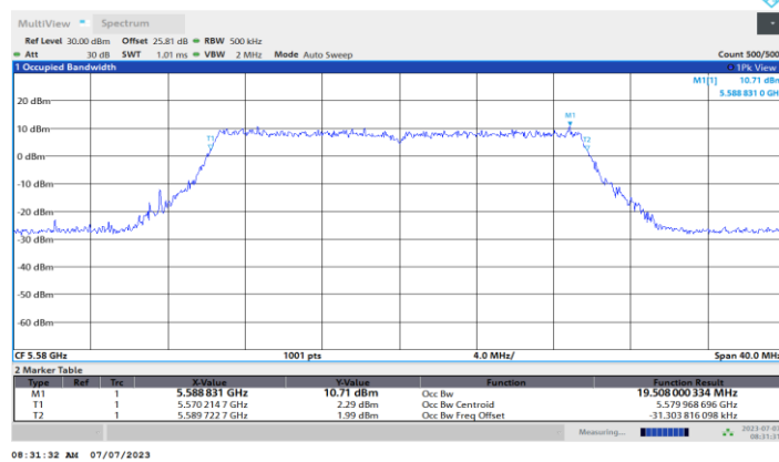
11BE20MIMO_Ant1_5580
