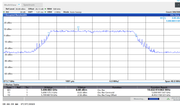
11BE20MIMO_Ant2_5700
