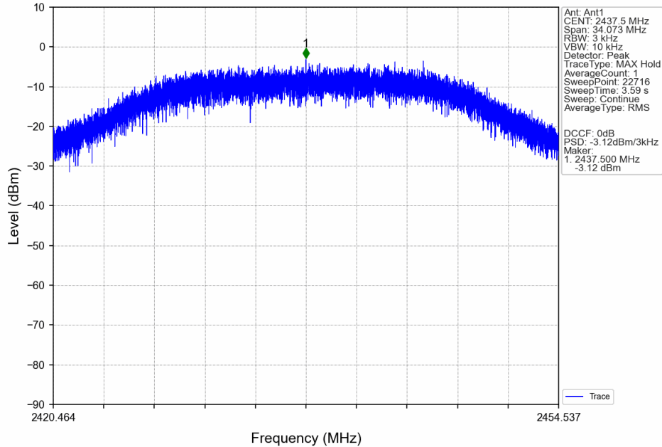
40M_MCH_2437.5MHz_MIMO_NTNV
