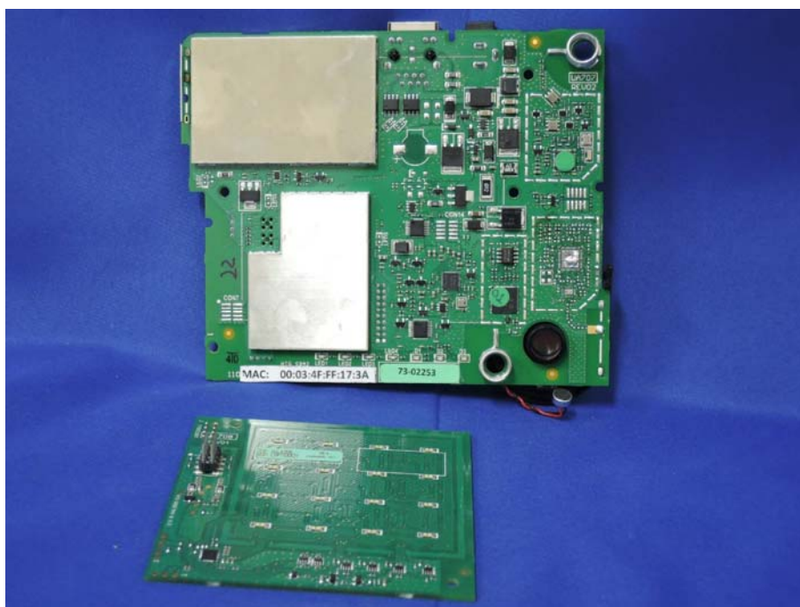
(15) EUT Photo
