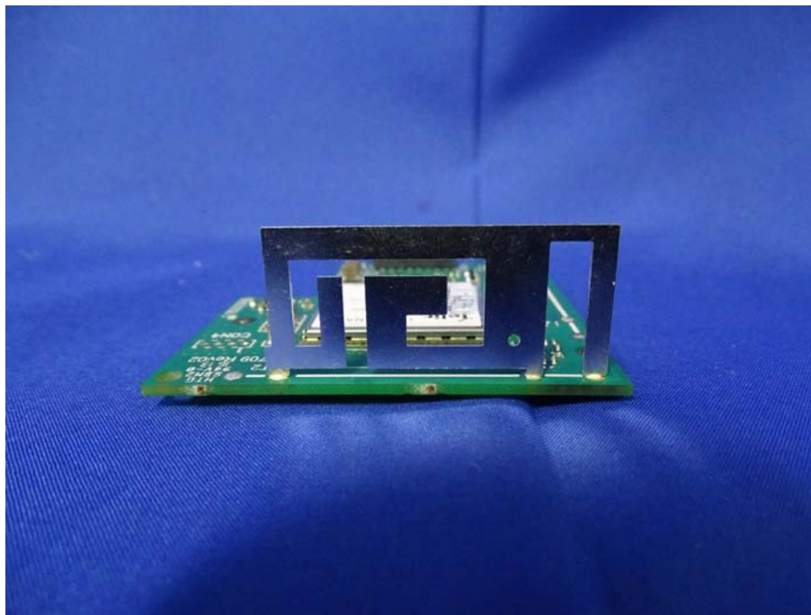
(9) EUT Photo
