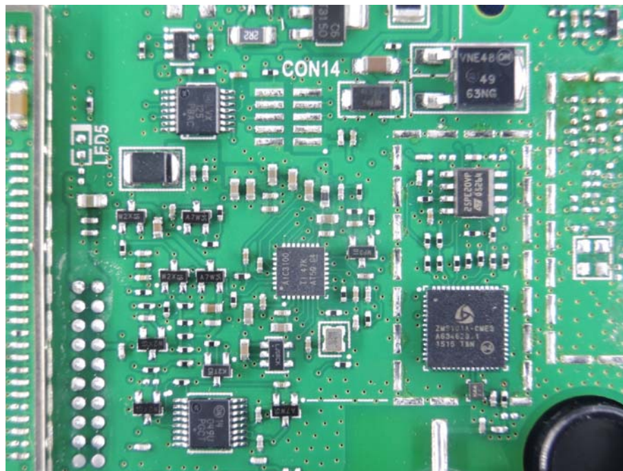
(24) EUT Photo
