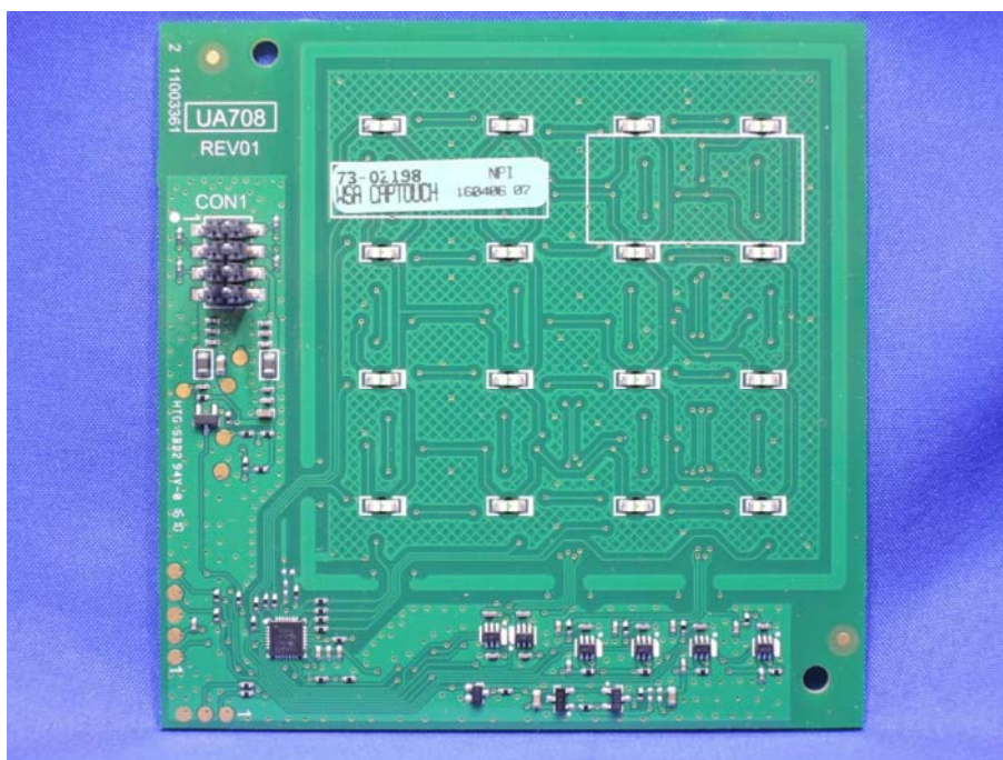
(17) EUT Photo
