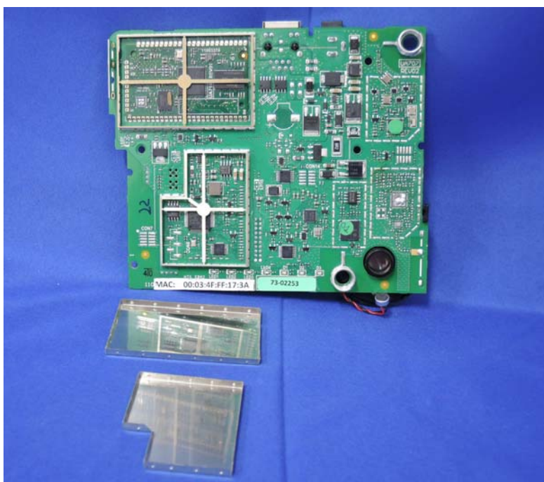
(19) EUT Photo
