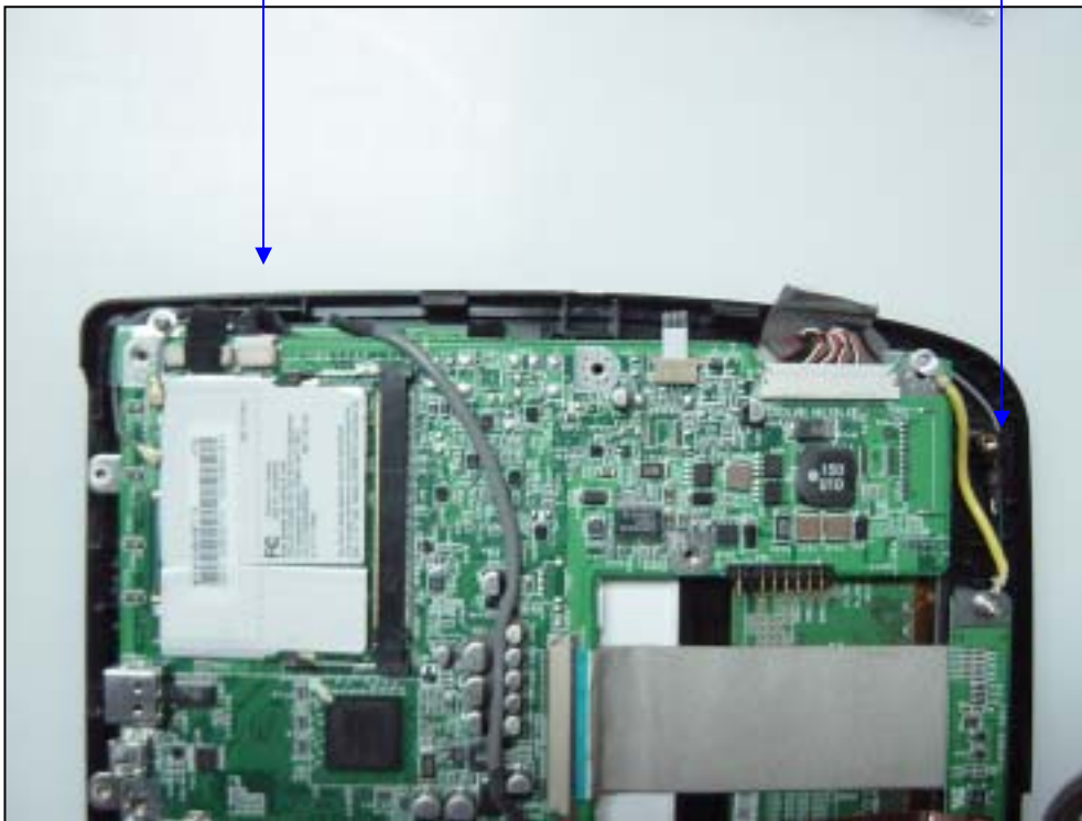
Aux Ant.
