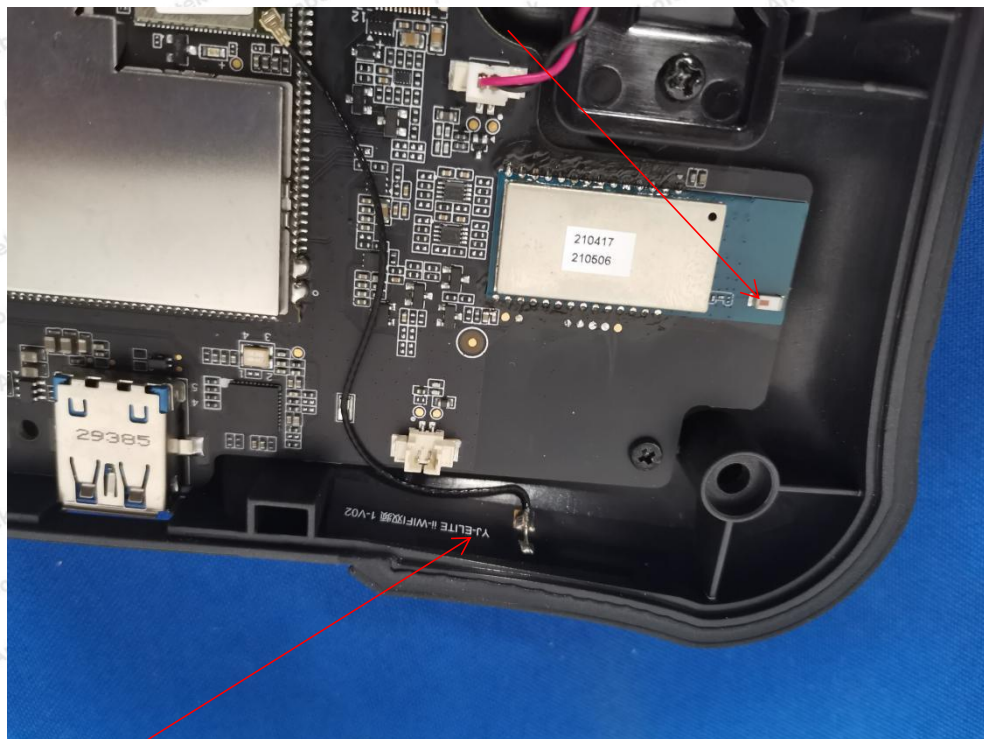
WLAN ANT1
