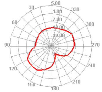
2480.000MHz H
