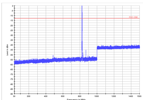
NB-IOT Band 5 CH-Middle 15KHz 30MHz-1.5GHz
