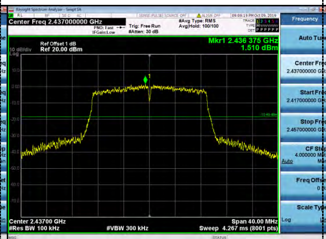
802.11n(HT20) CH06
