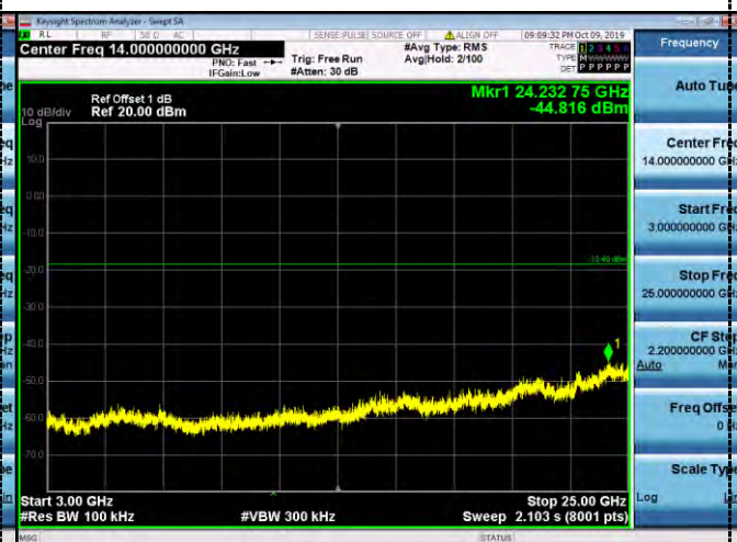
3GHz-25GHz
