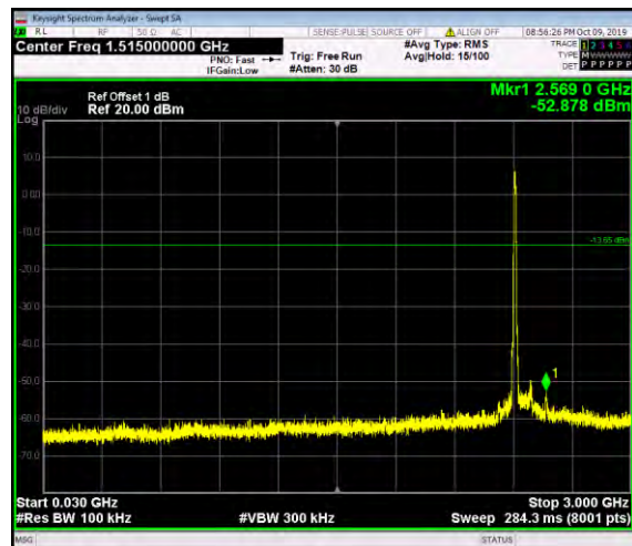
30MHz-3GHz
