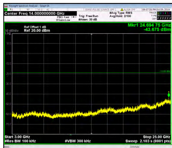
3GHz-25GHz
