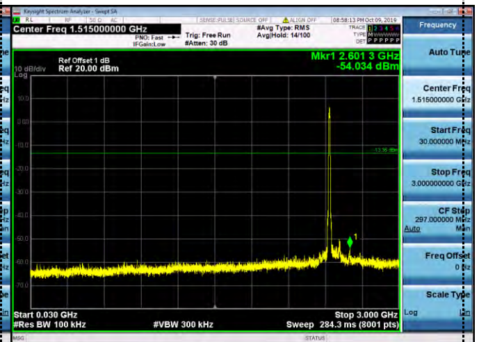
30MHz-3GHz
