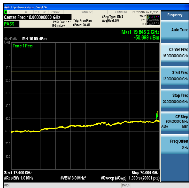
NTNV-n66-PC3-15-45-M-DFT-BPSK-Edge_1RB_Left- 12000-20000-PASS
