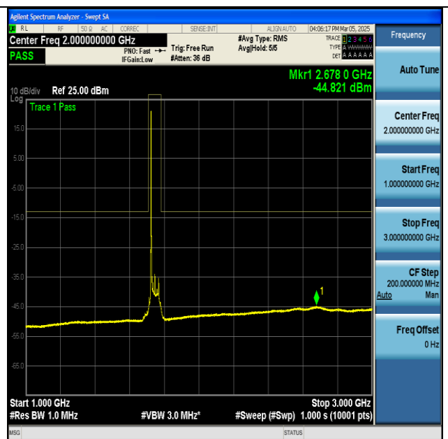
NTNV-n66-PC3-15-45-M-CP-QPSK-Edge_1RB_Left-1000-3000-PASS
