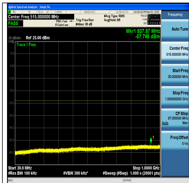
NTNV-n66-PC3-15-45-M-CP-QPSK-Edge_1RB_Left-30-1000-PASS
