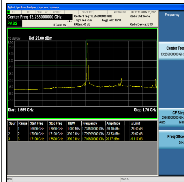
NTNV-n66-PC3-15-40-L-CP-QPSK-Edge_1RB_Left-PASS
