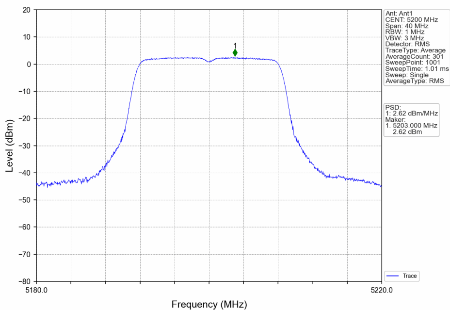
802.11a_MCH_5200MHz_Ant1_NTNV
